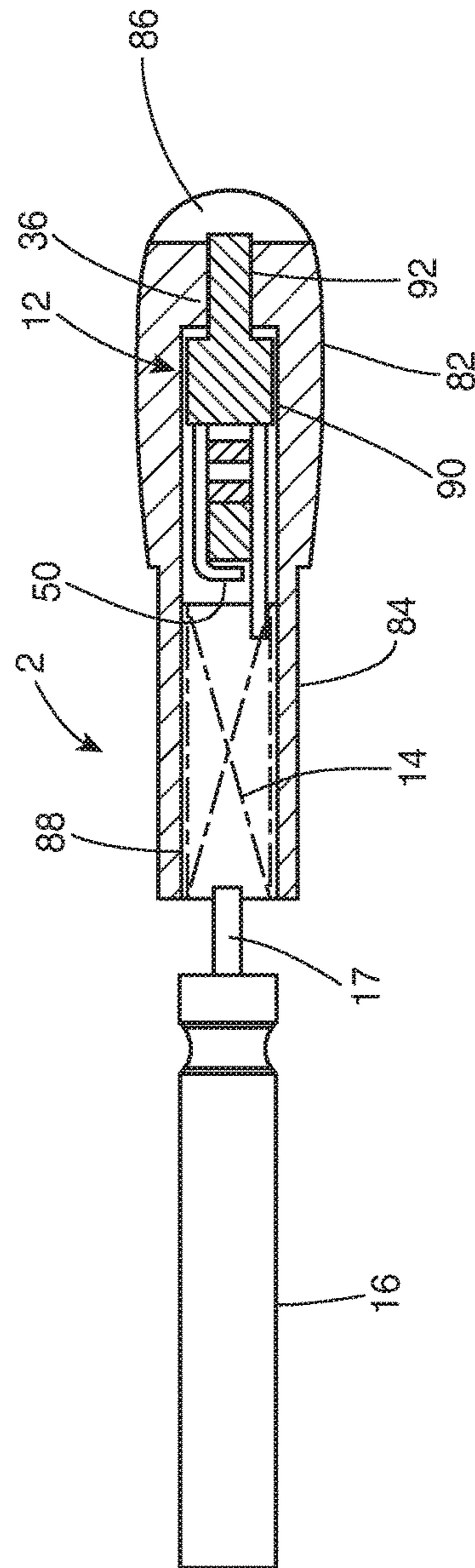
FIG. 7
