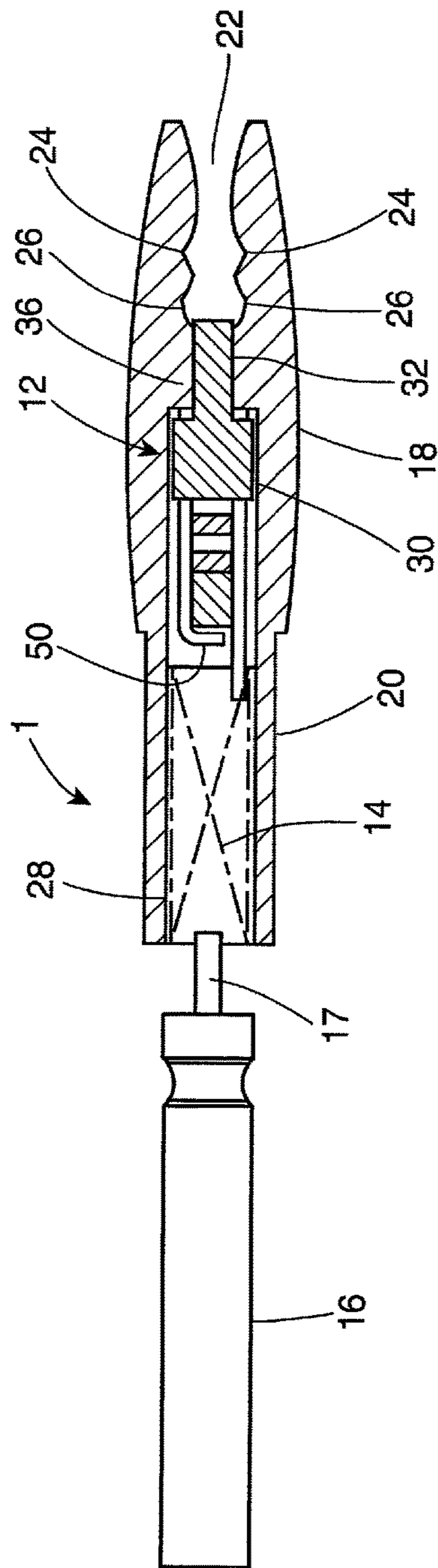
FIG. 2
