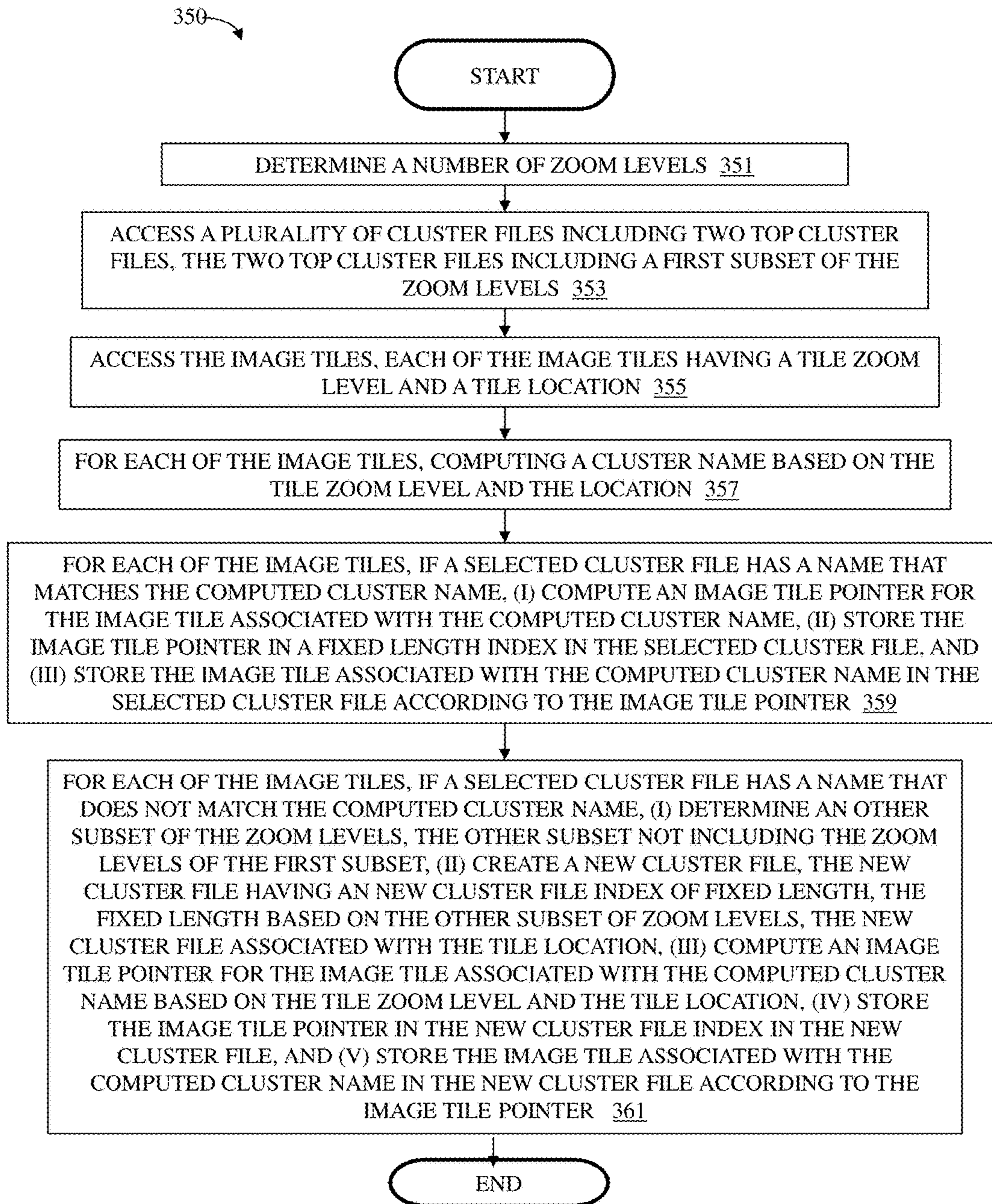
FIG. 15B
