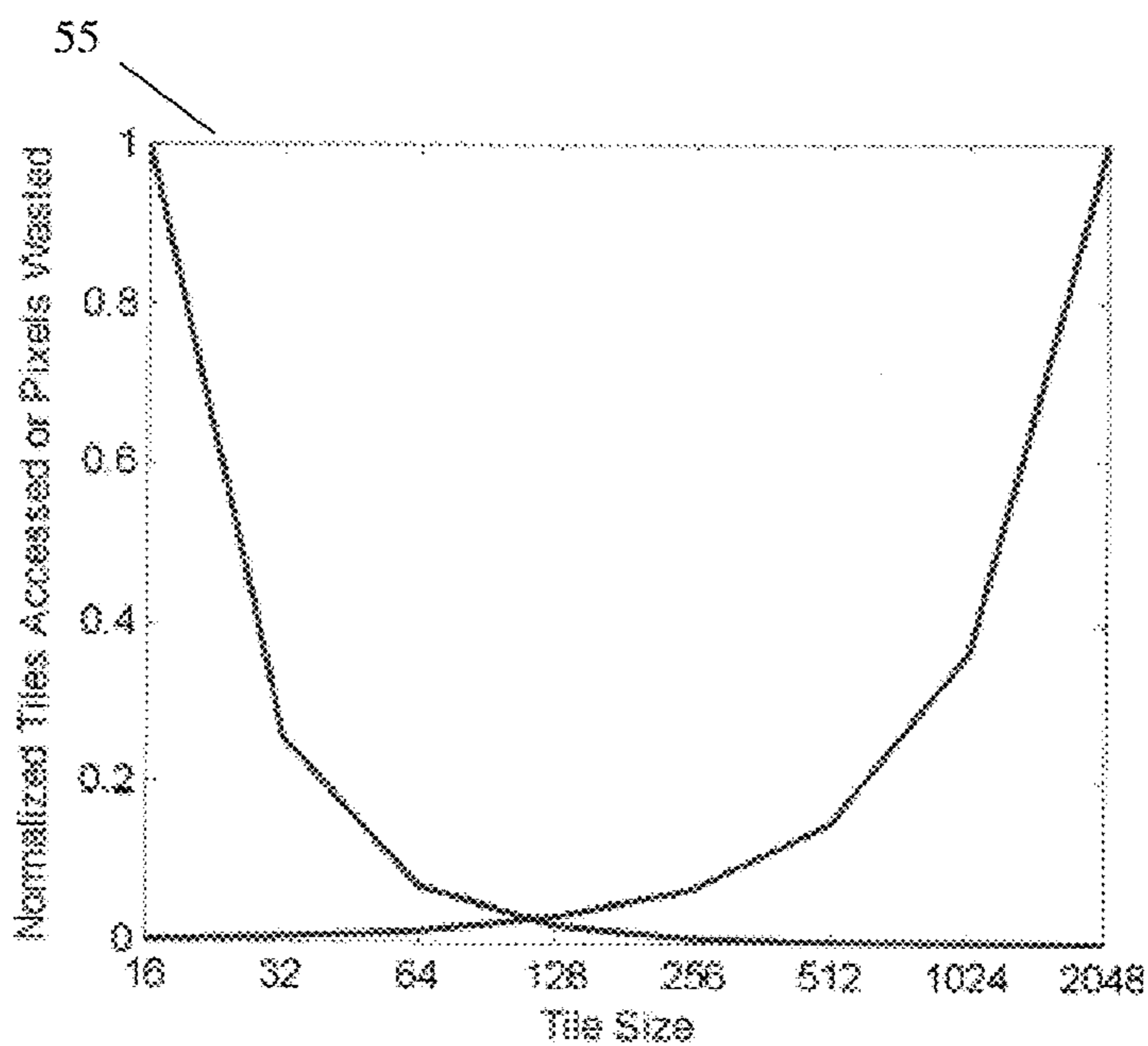
FIG. 9A
