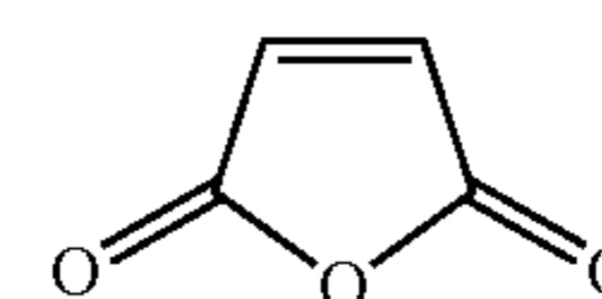
Maleic anhydride
