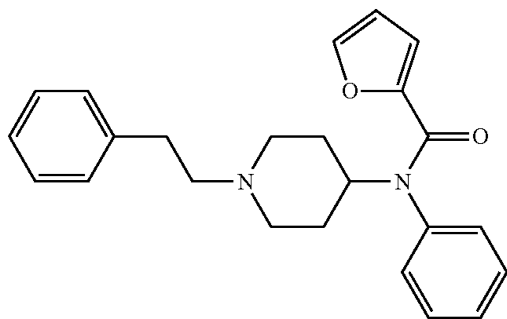
Furanylfentanyl
