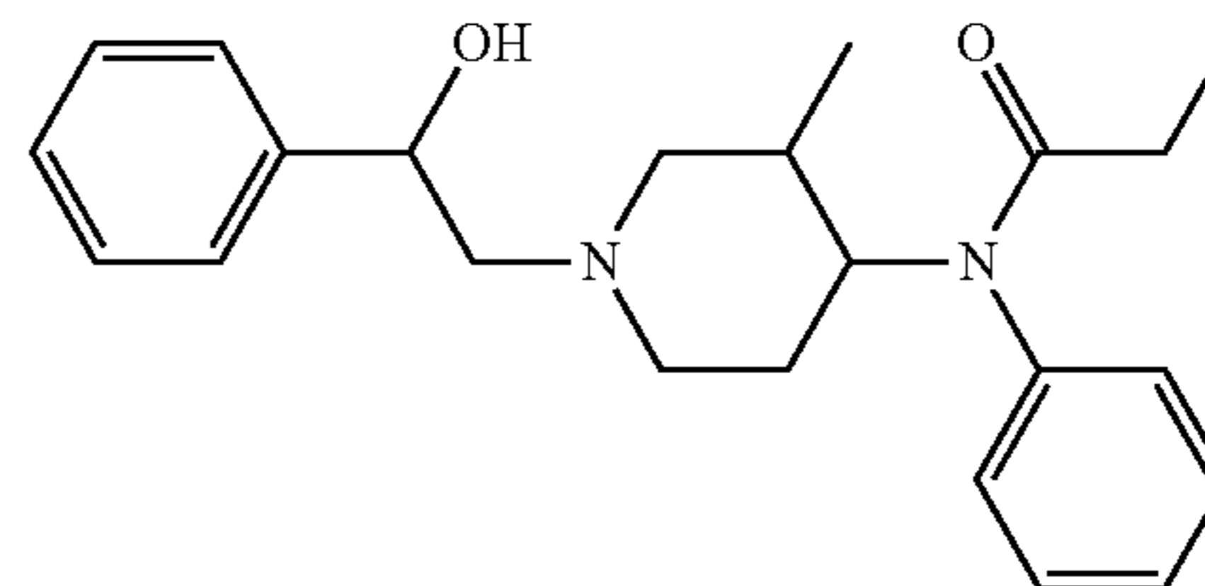
Ohmefentanyl
