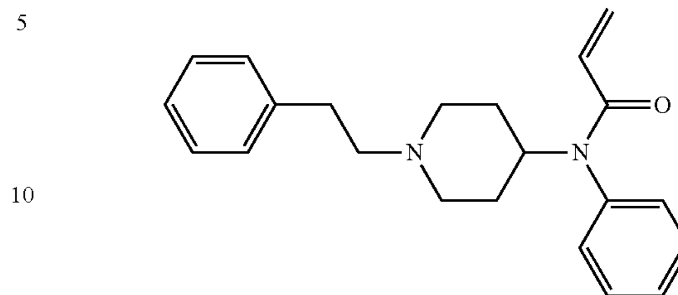
Acrylfentanyl
