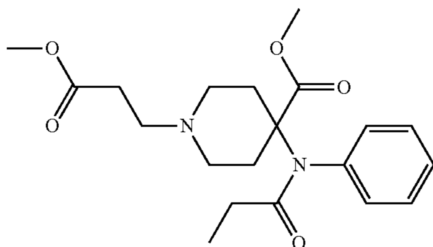
Remifentanyl
