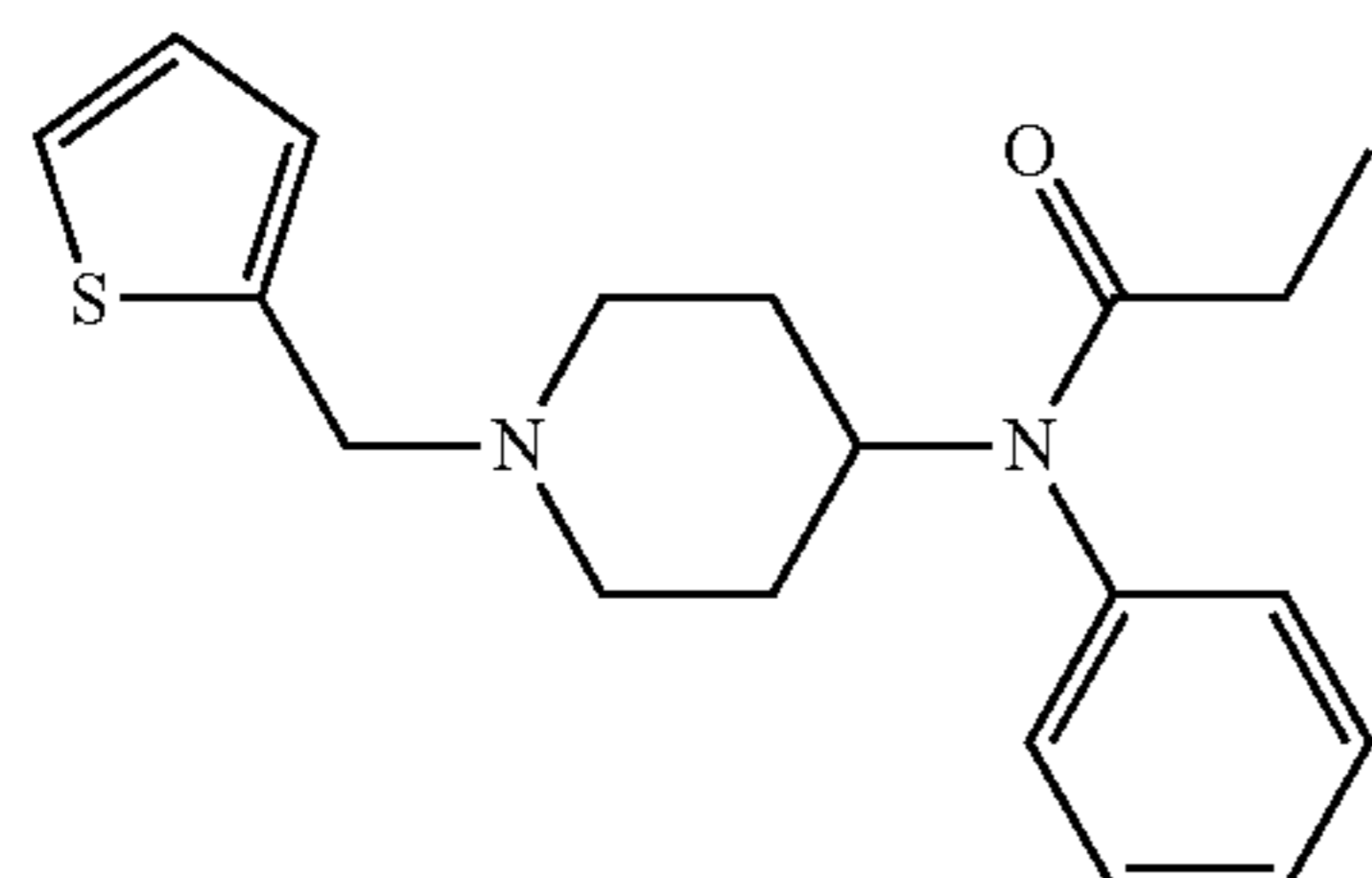
Thenylfentanyl
