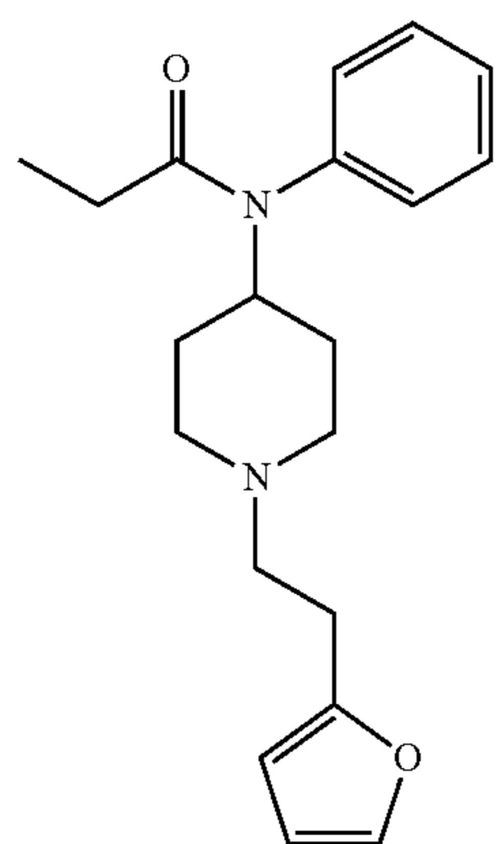
Furanylethylfentanyl
