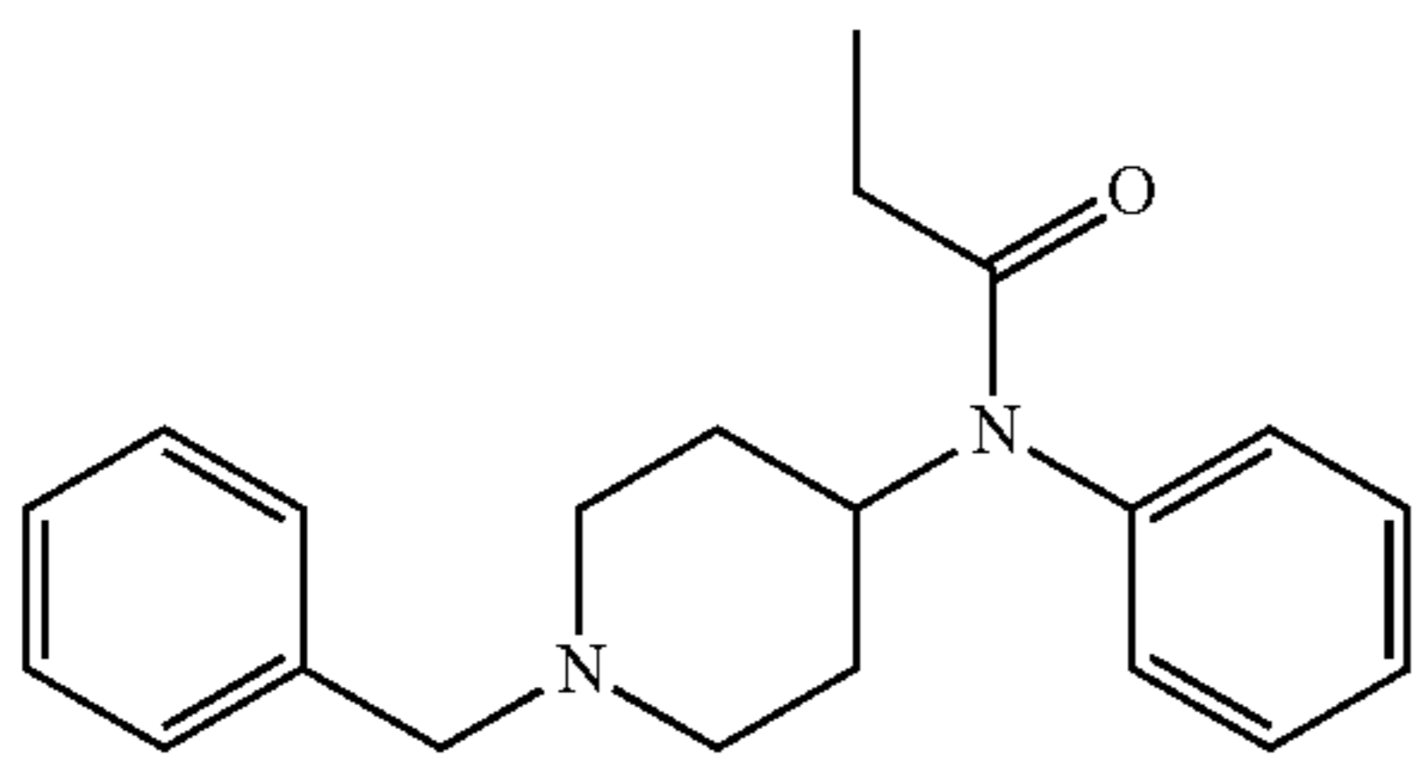
Benzylfentanyl
