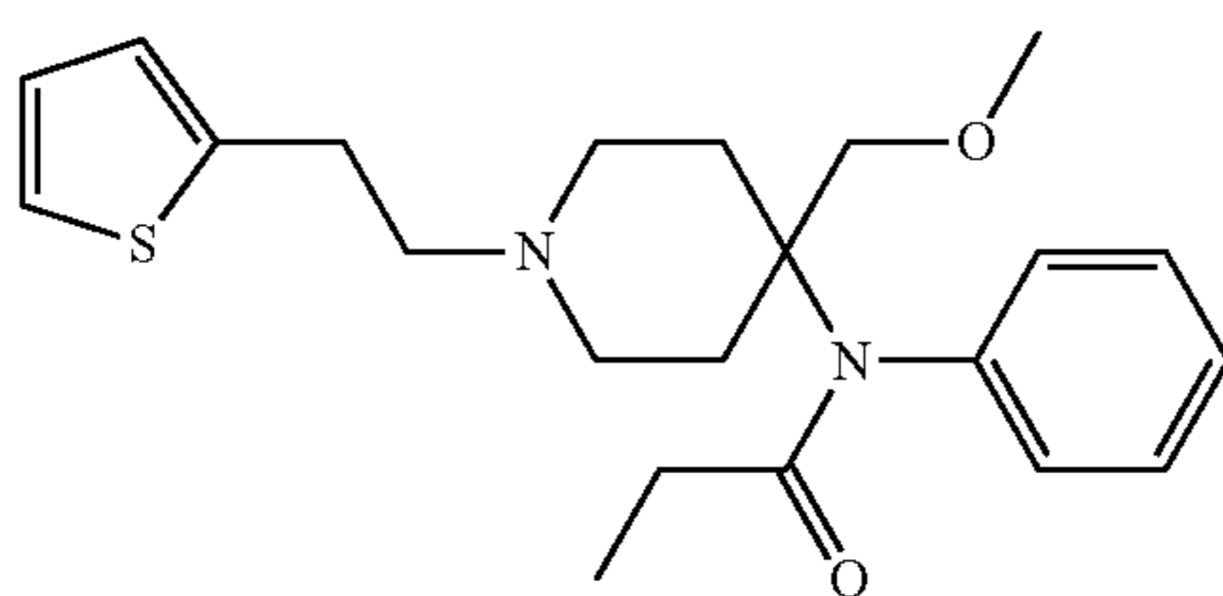
Sufentanyl
