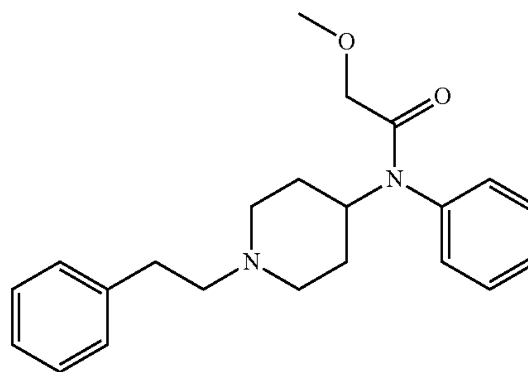
Methoxyacetylfentanyl
