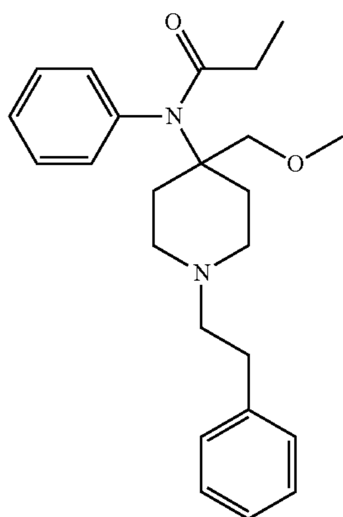
R-30490
