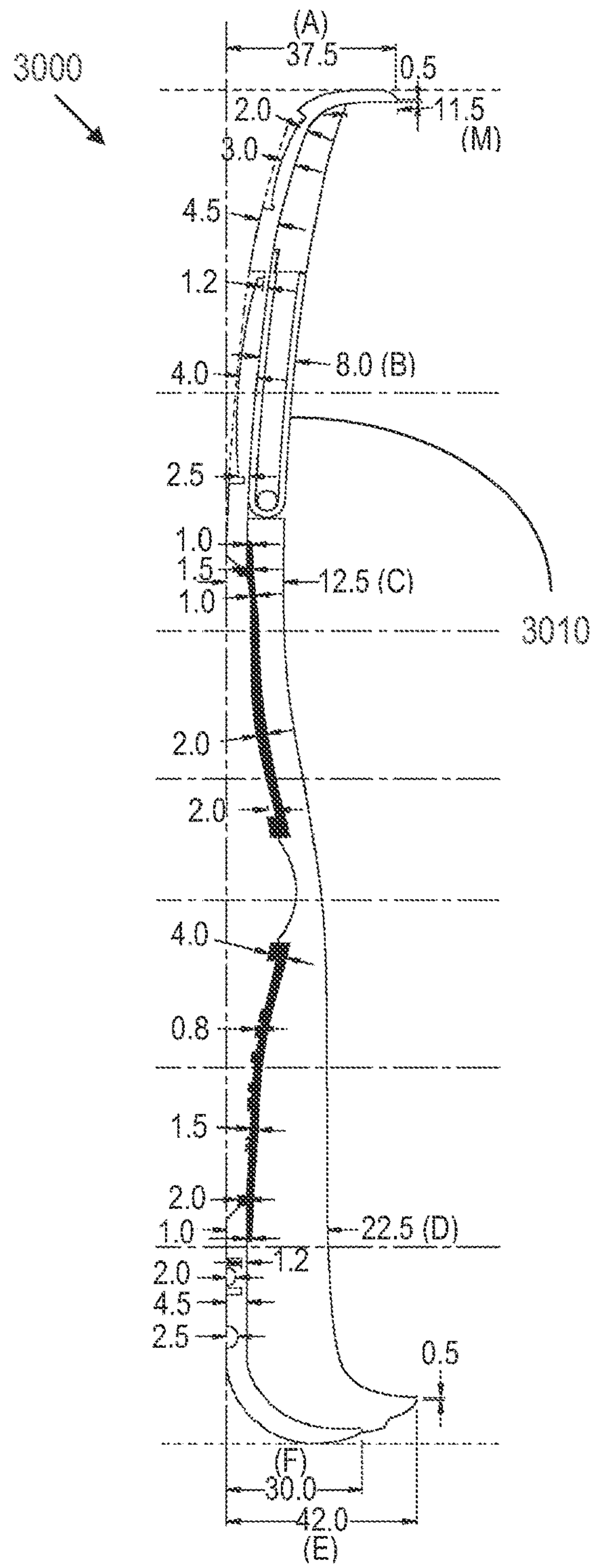
SECTION A-A'
