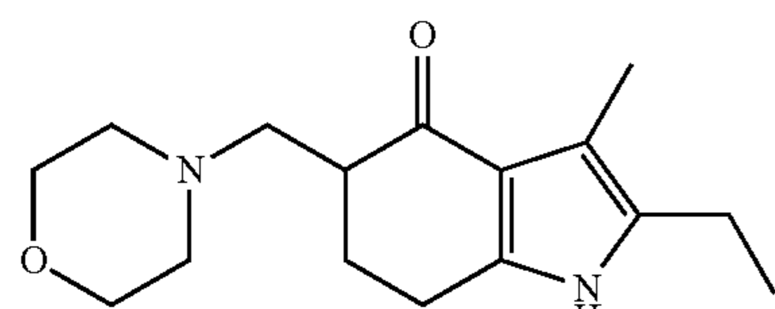
SUMO-3 isomer
