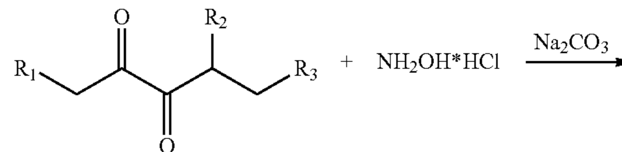
Diones
