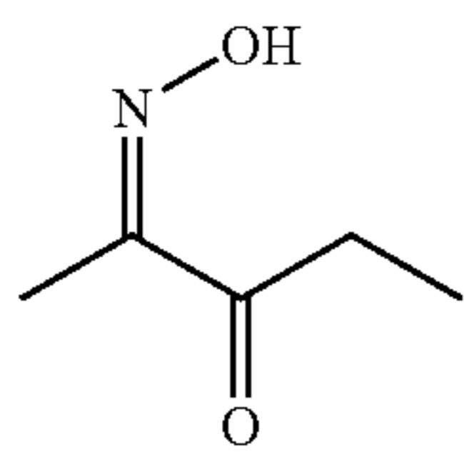
2,3-Pentanedione-2-oxime (SUMO-1)
