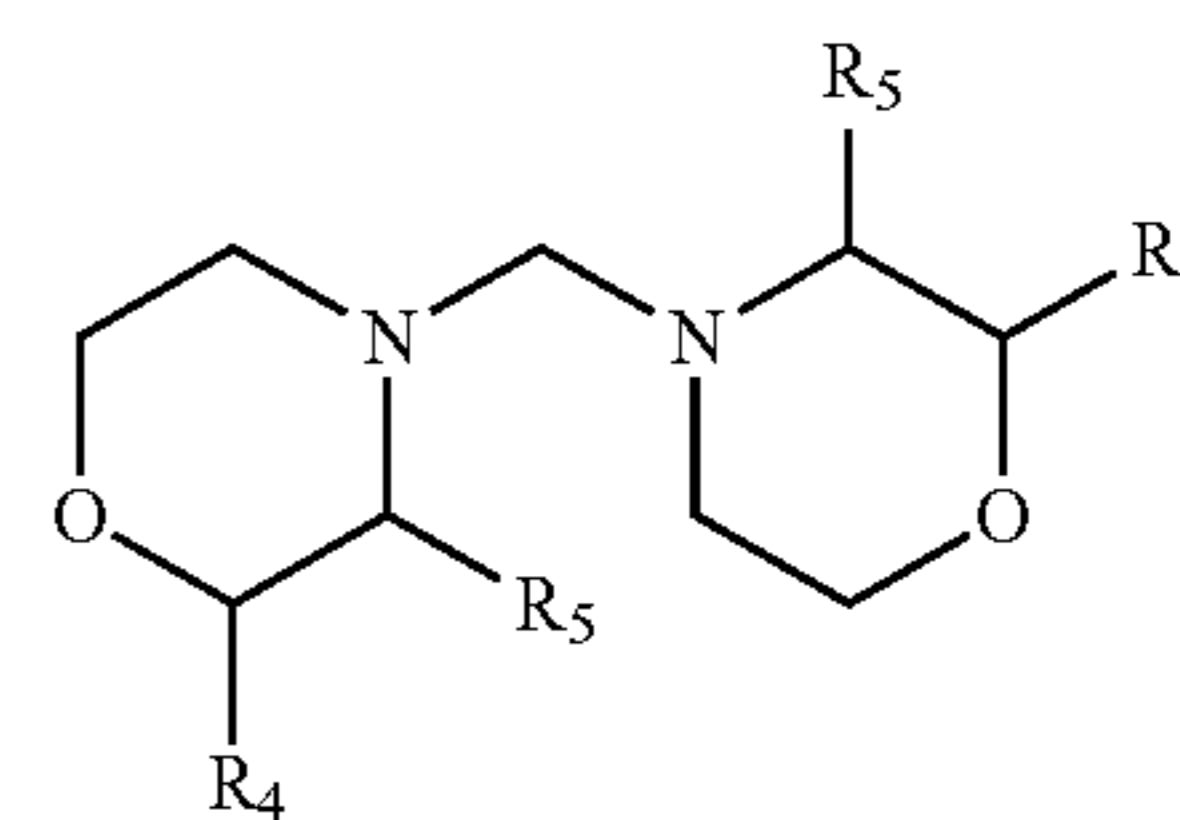
Bismorpholinomethane Analogs
