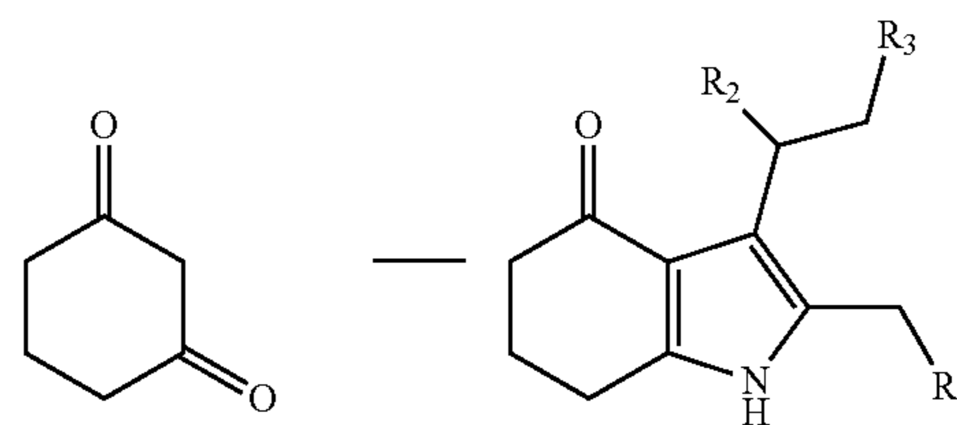
1,3-Cyclohexanedione
