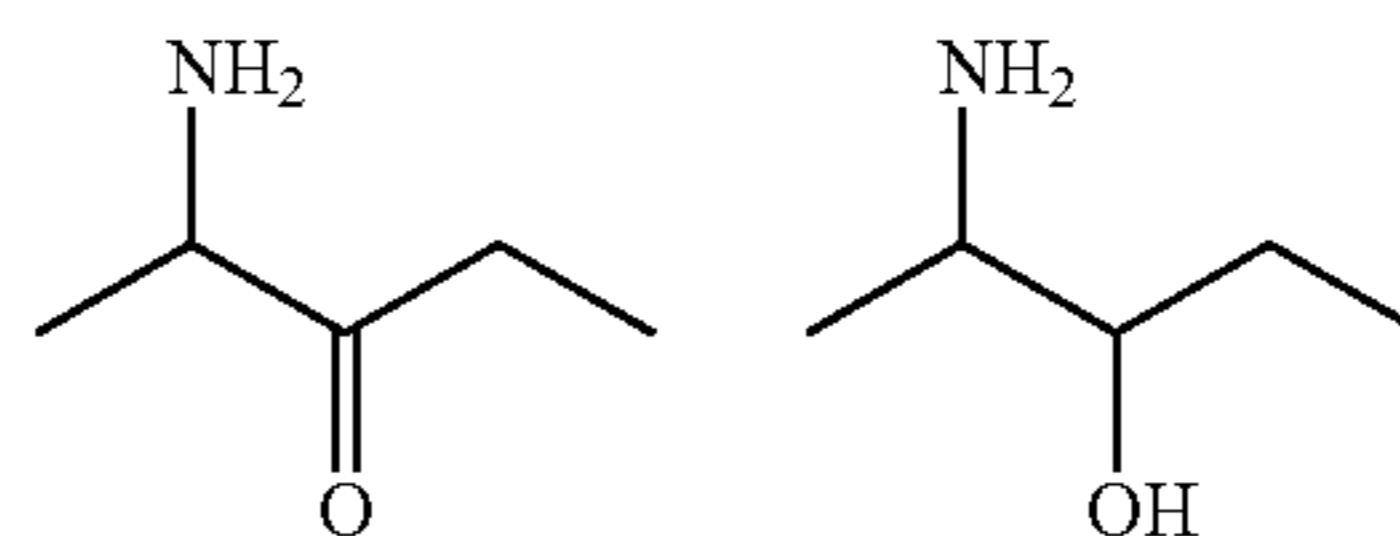
2-Amino-pentan-3-one 2-Amino-pentan-3-ol
