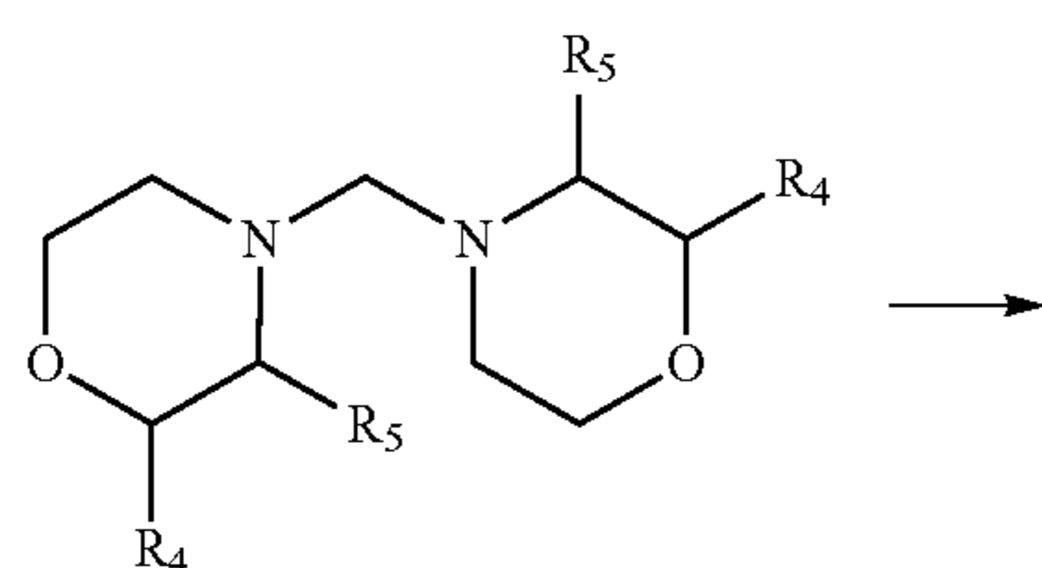
Bismorpholinomethane Analogs
