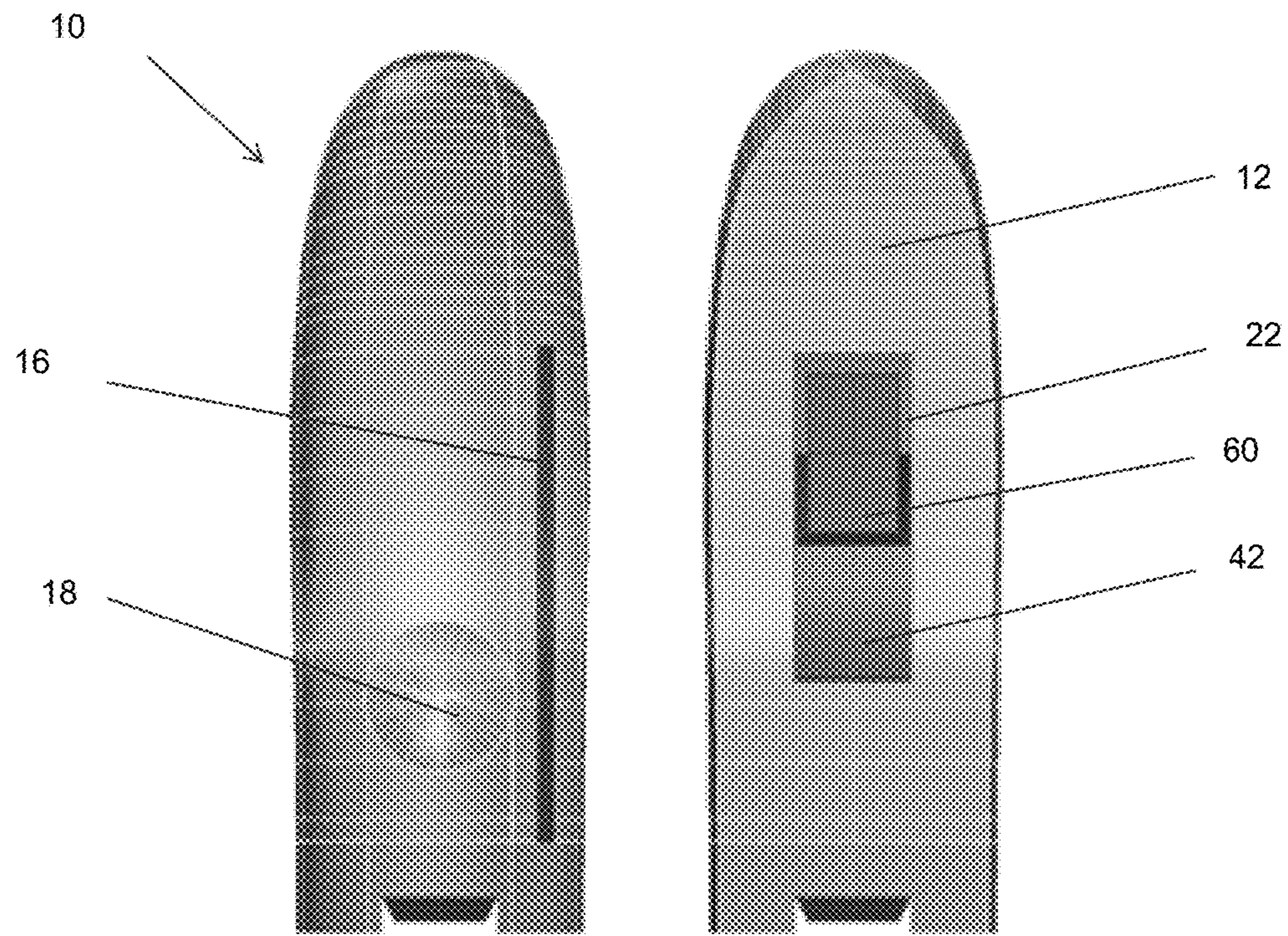
FIG. 4A
