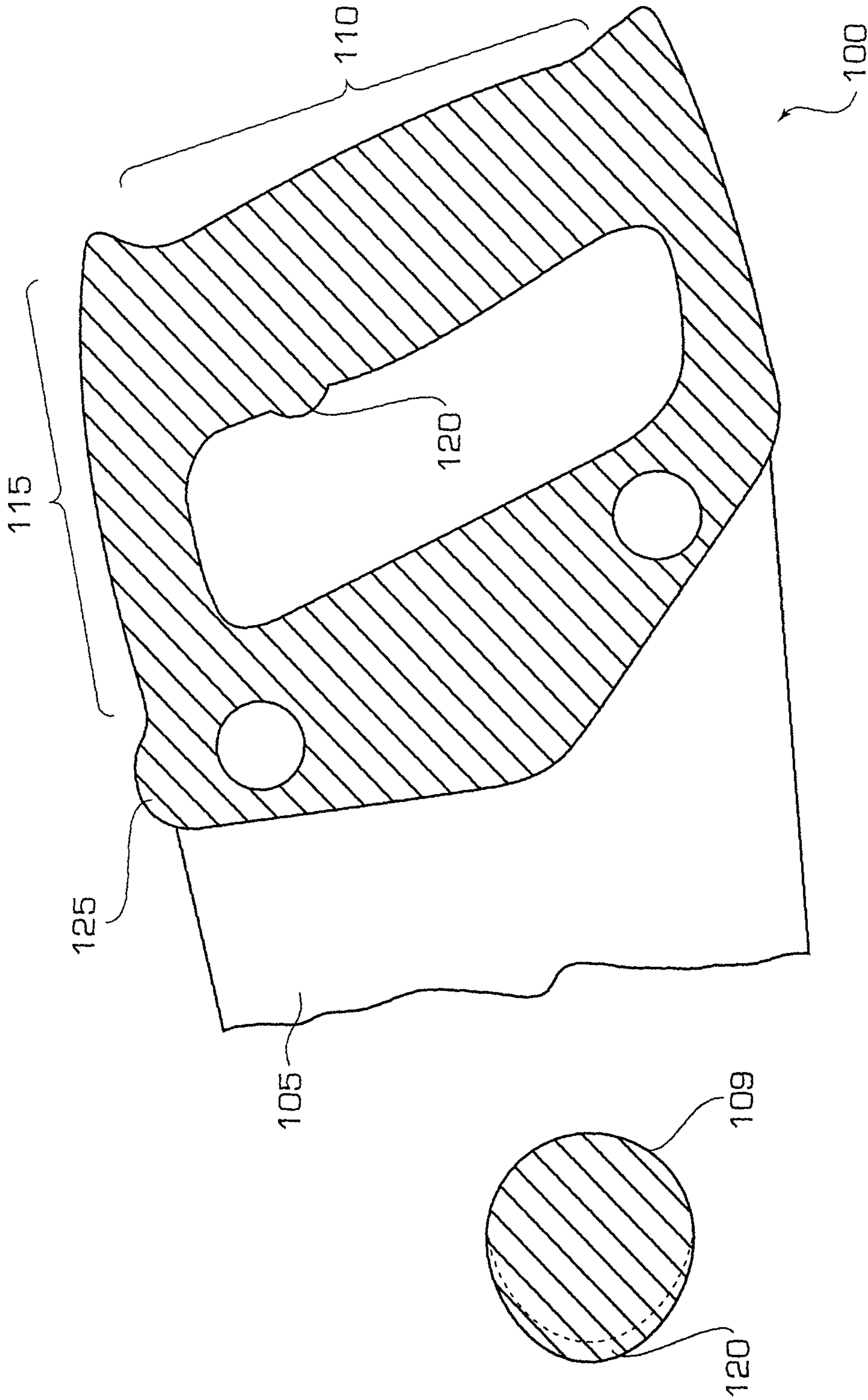
FIG. 1B
