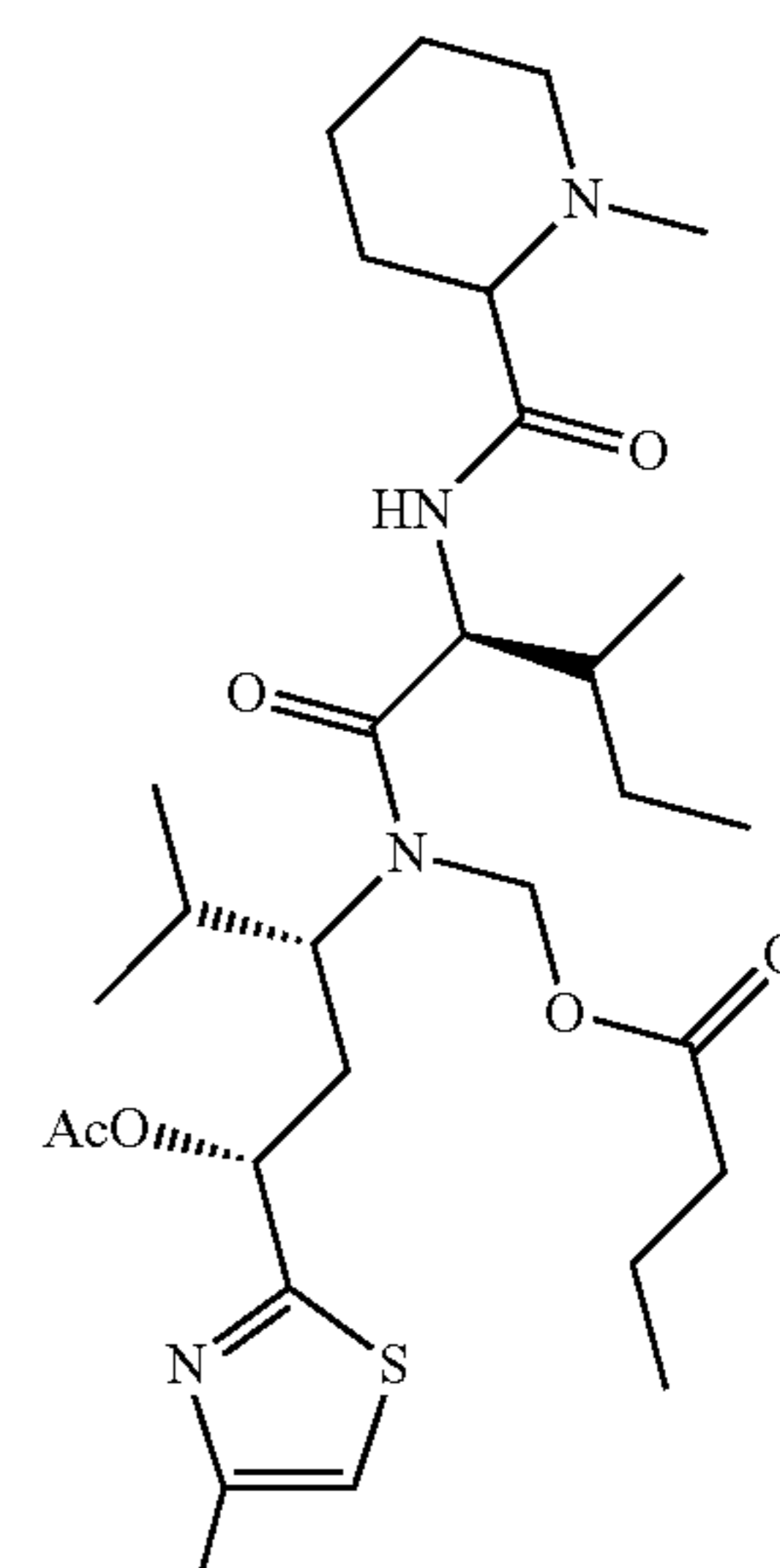
Conjugate 24
