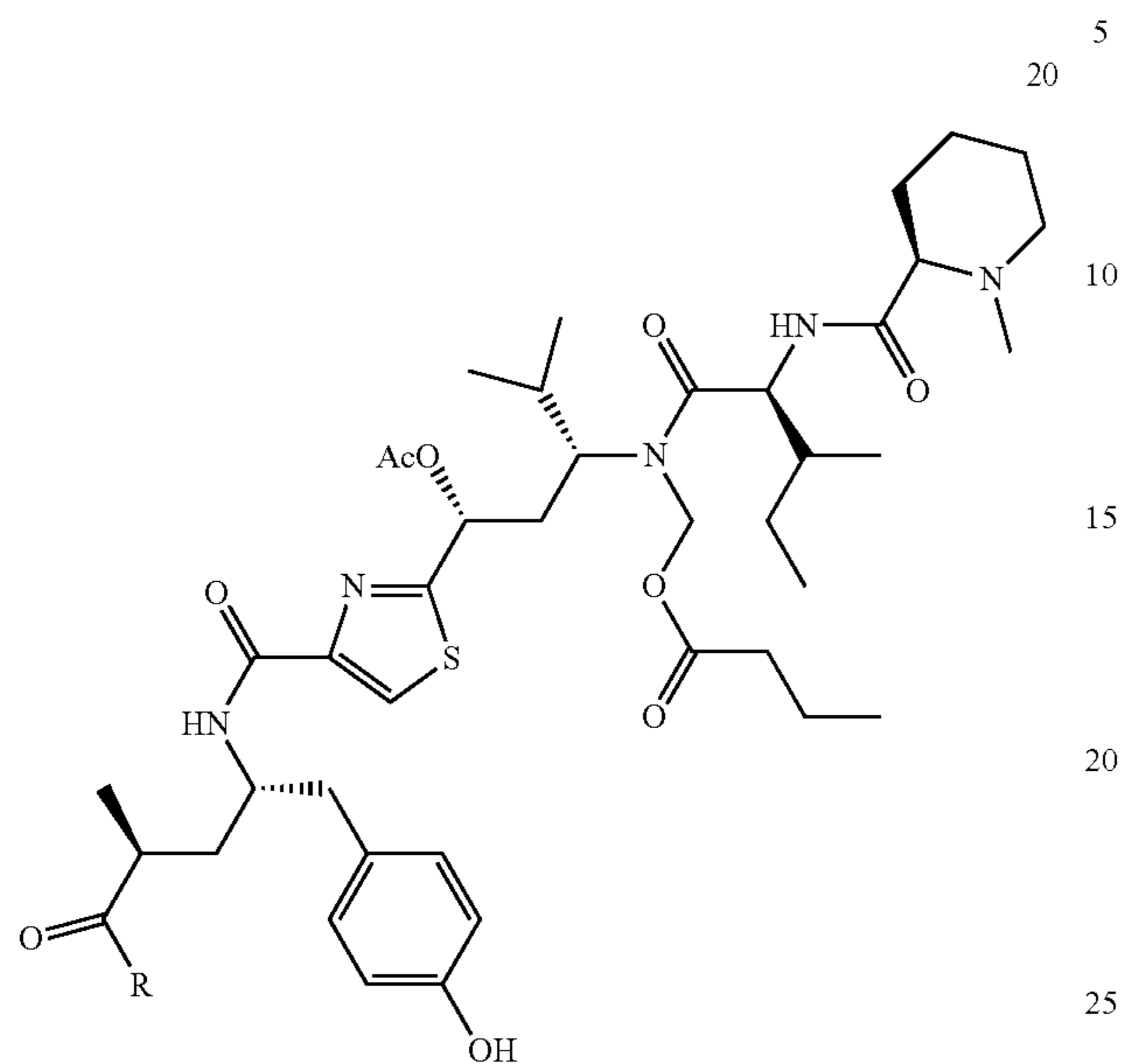
Tubulysin B: R = OH Tubulysin B hydrazide: R = NHNH 2
