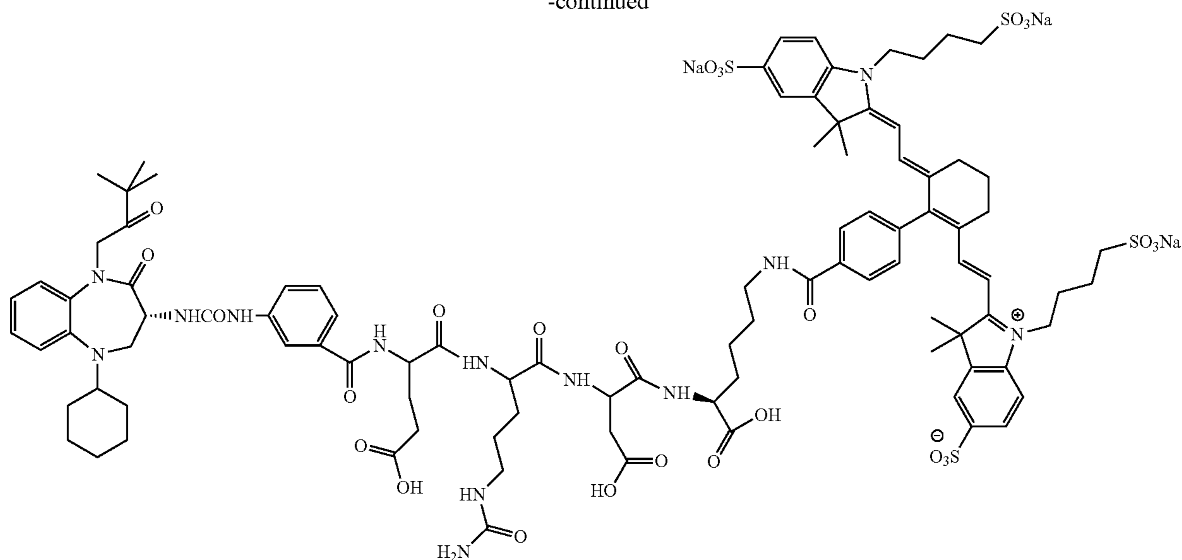
Conjugate 19
