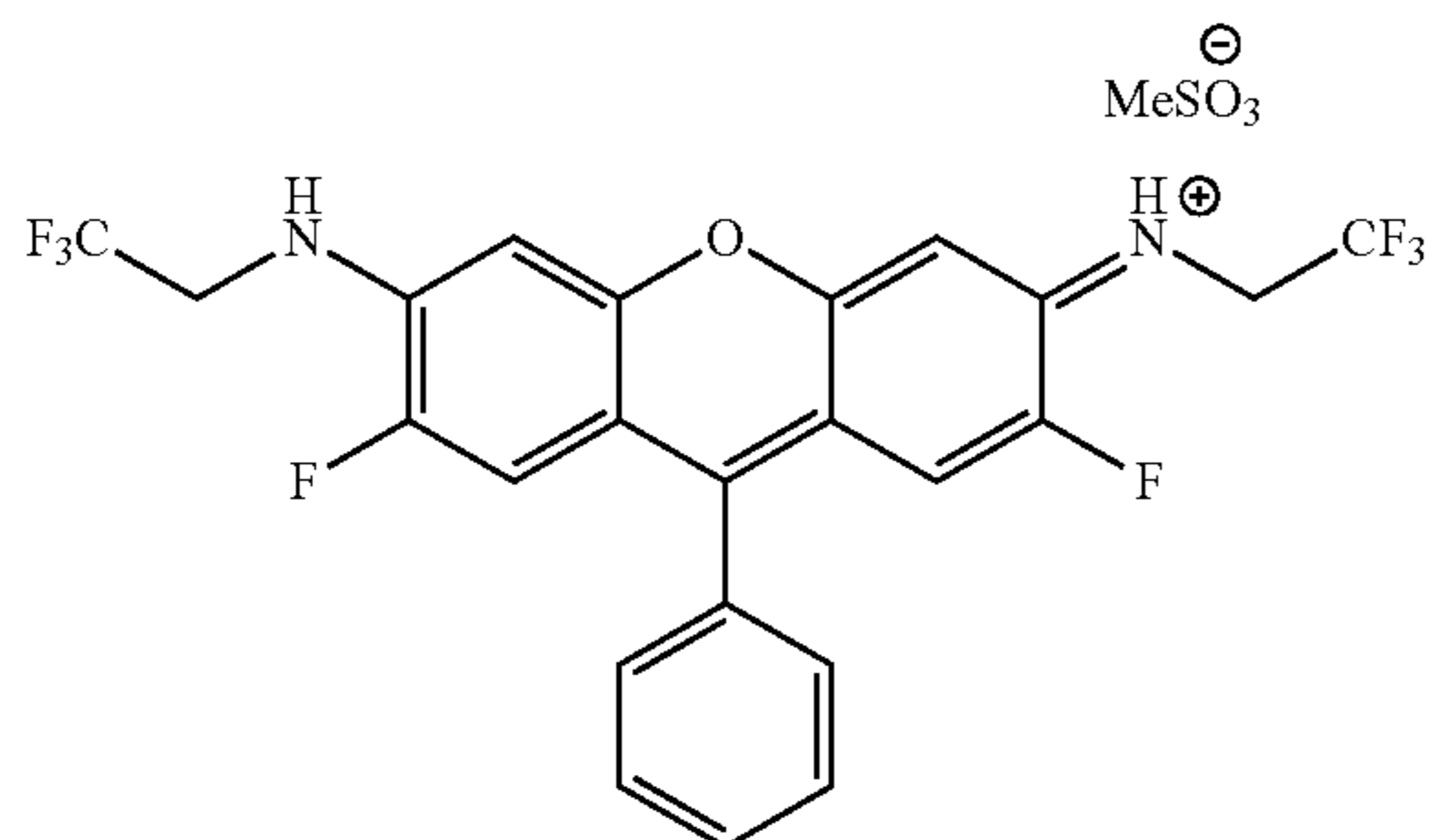
(Z)-N-(2,7-difluoro-9-phenyl-6-((2,2,2-trifluoroethyl)amino)-3H-xanthen-3-ylidene)-2,2,2-trifluoroethan-1-aminium methanesulfonate
