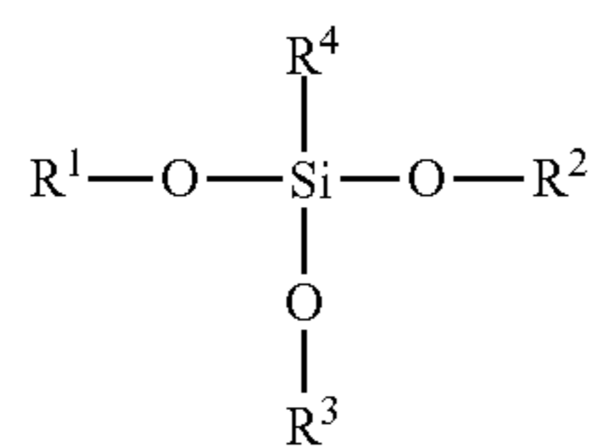
Alkoxy silane
