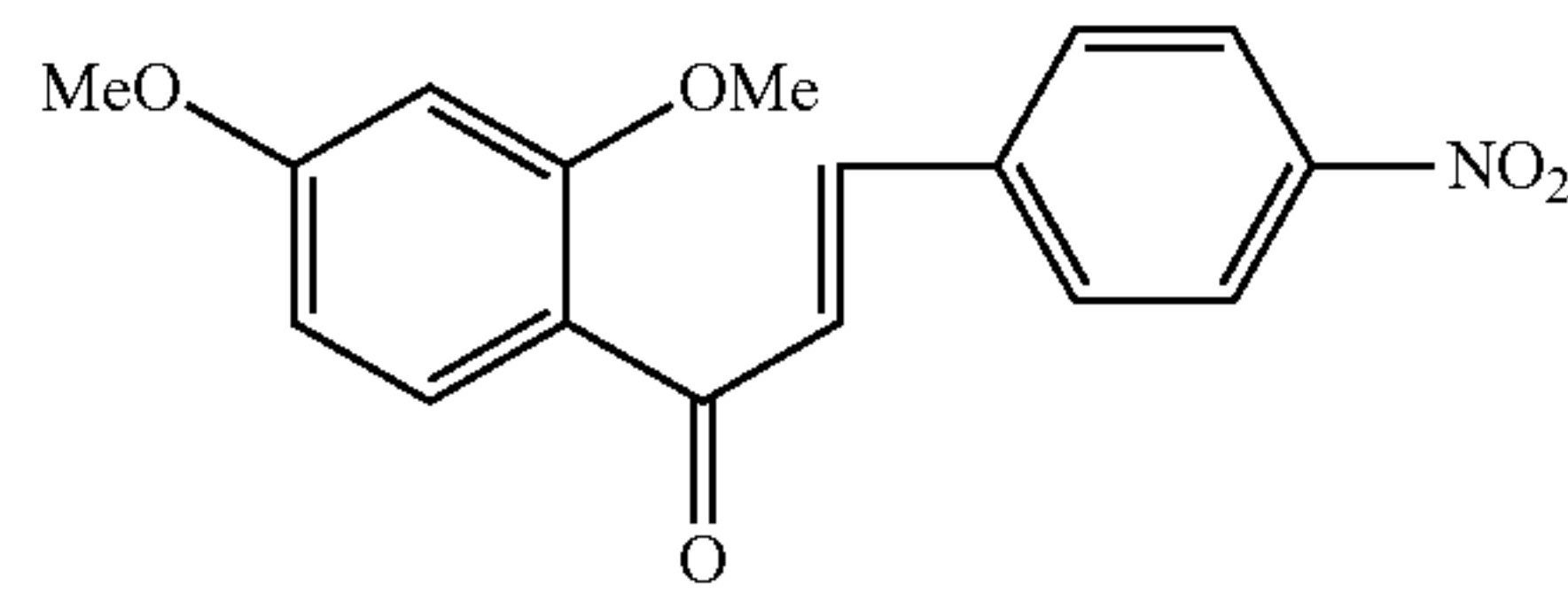
55
