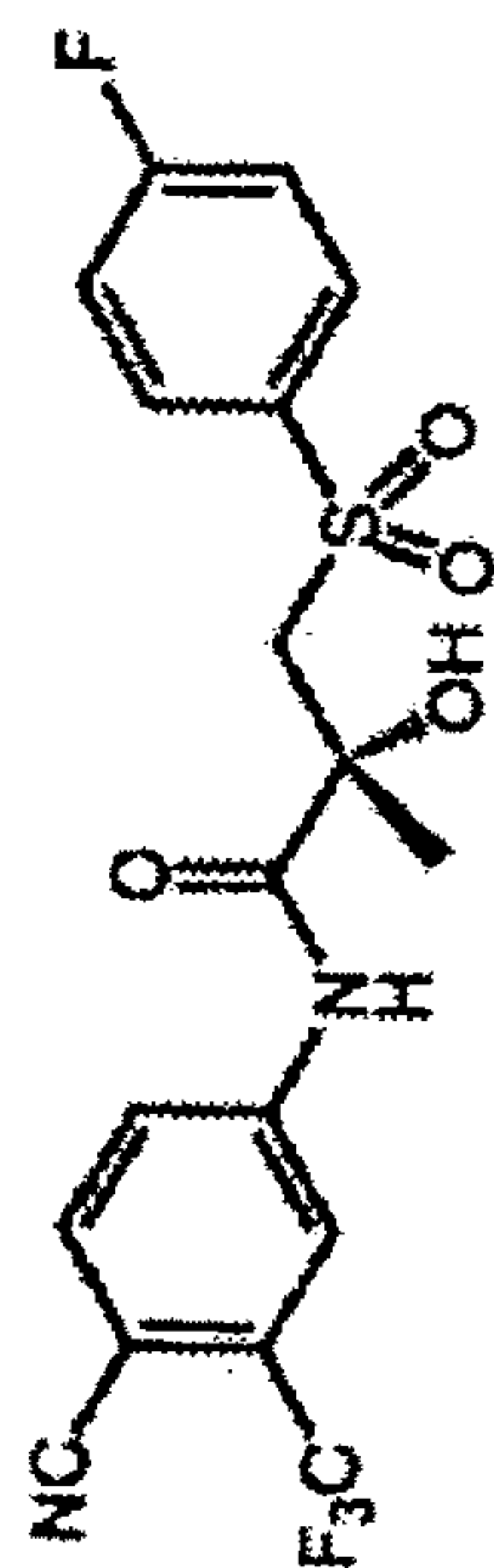
Bicalutamide
