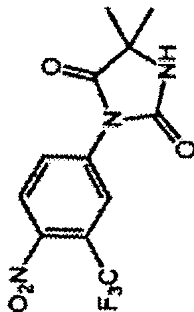
Nilutamide
