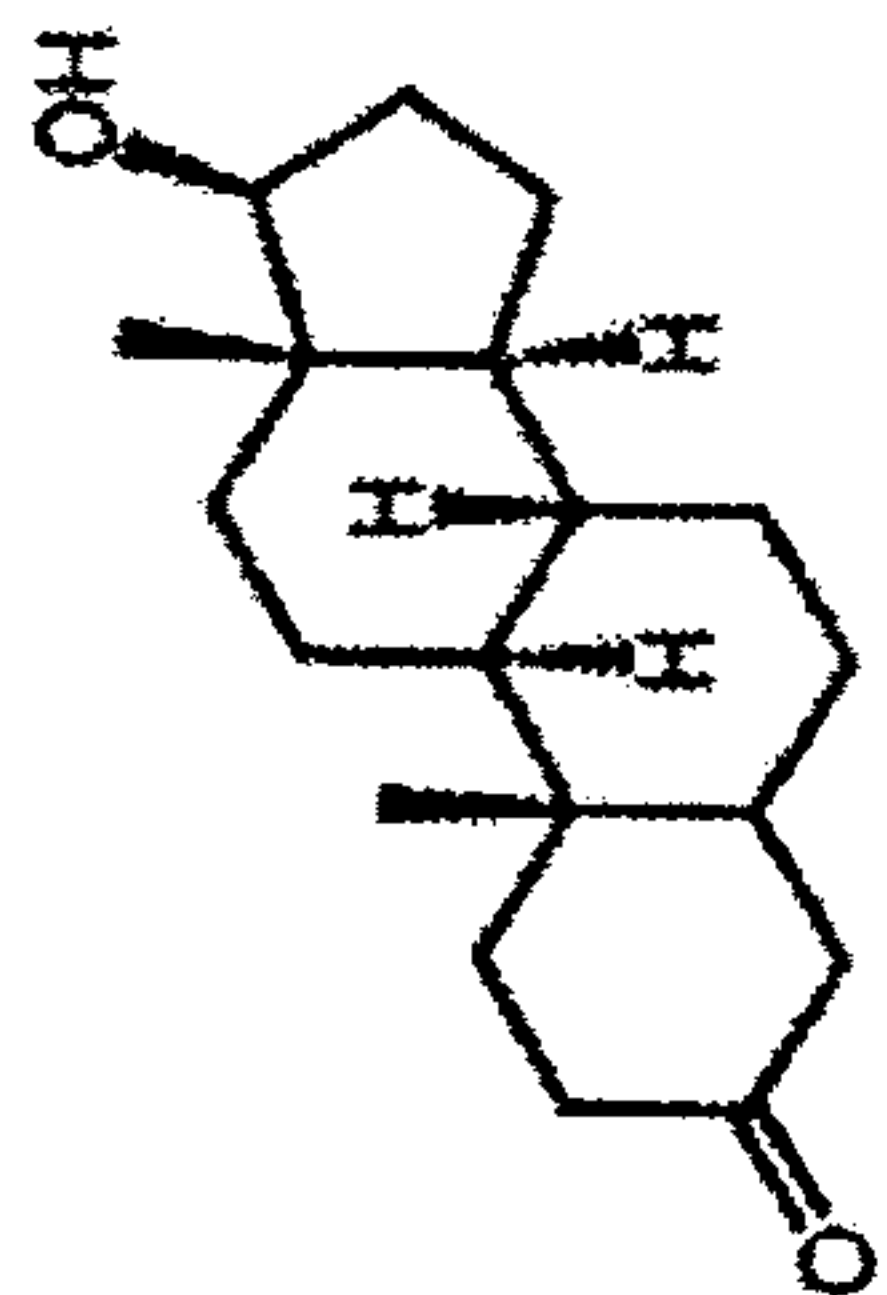
DHT
