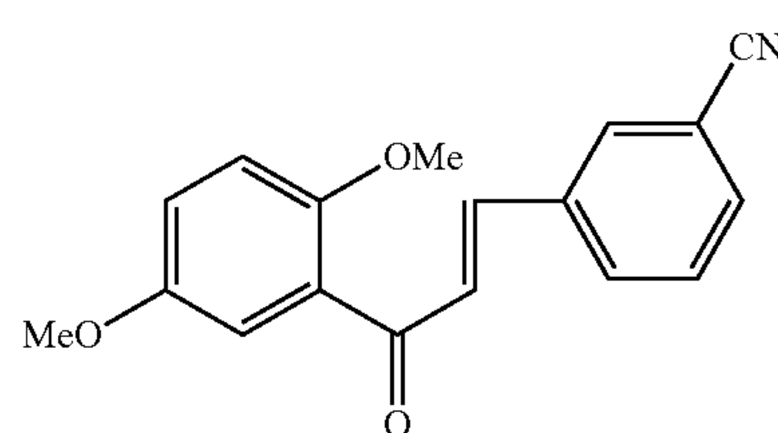
15
