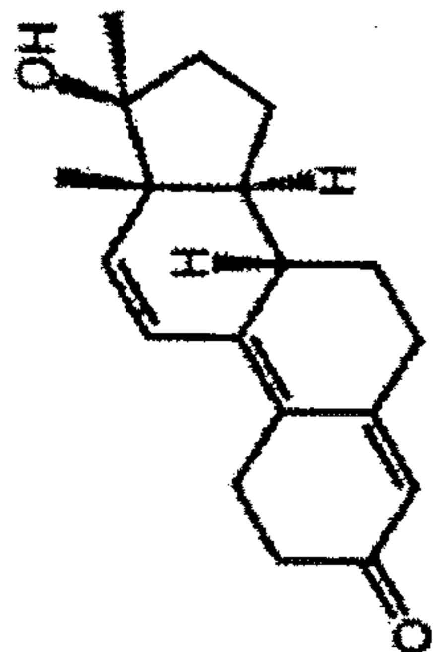
R1881
