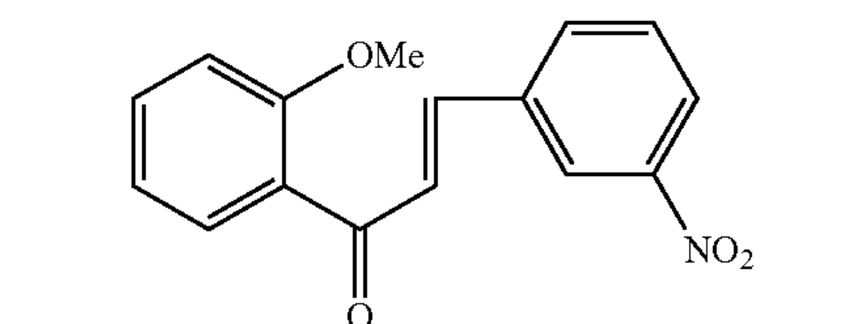
60
