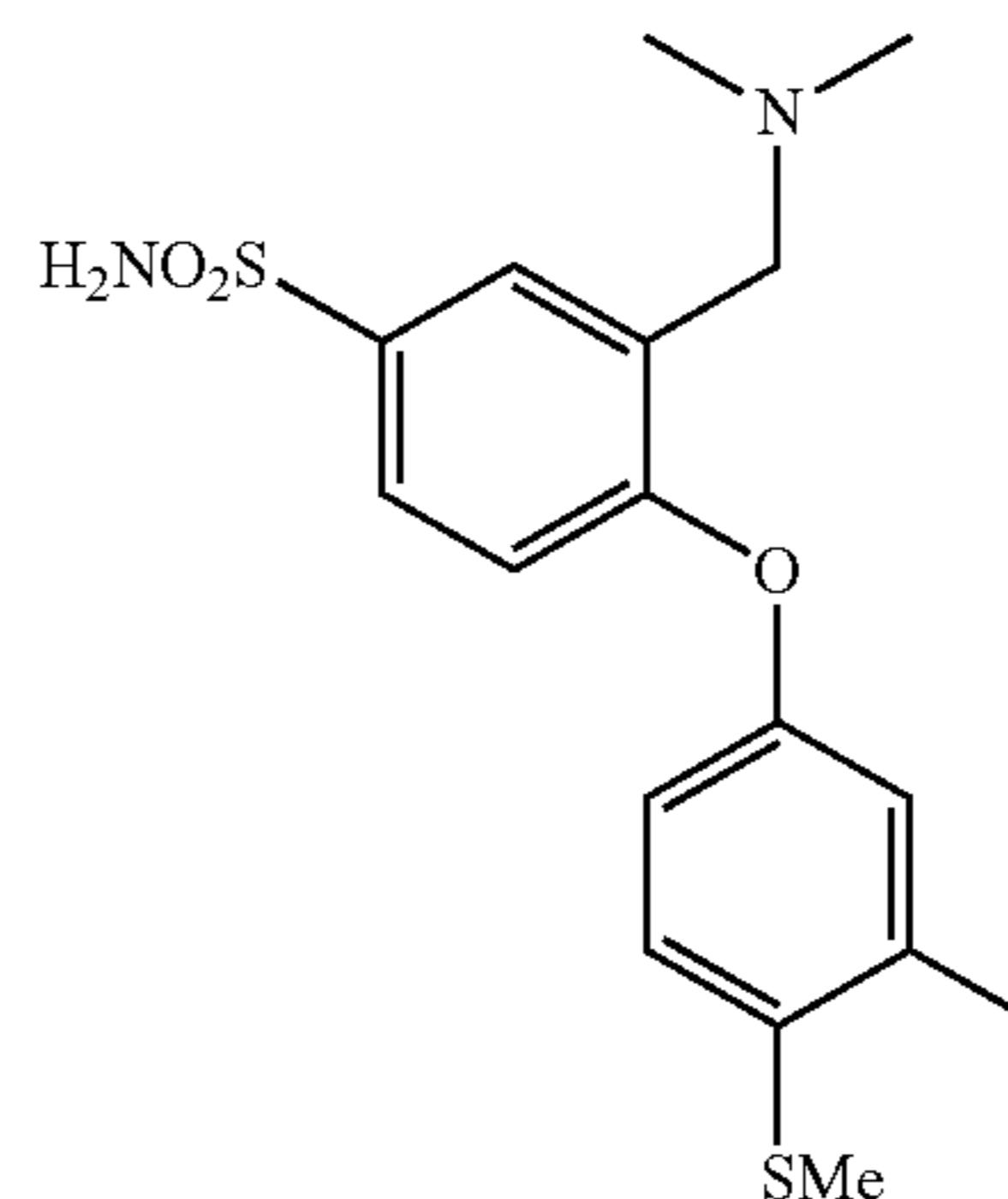
UK-416244
