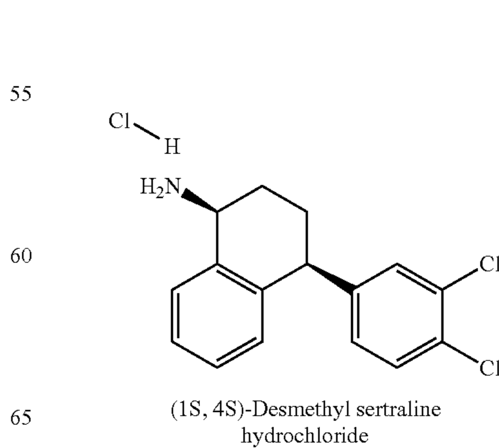
Sertraline-CME
