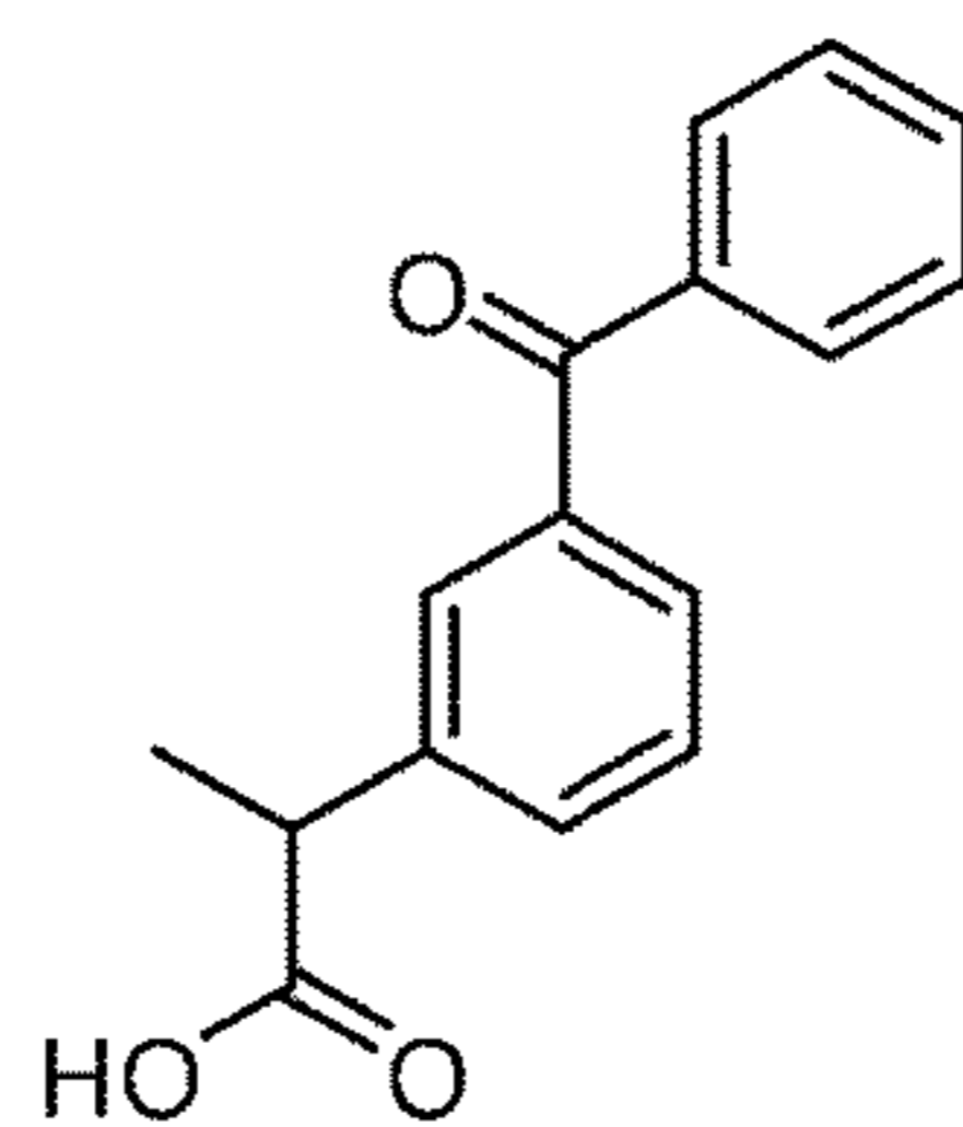
Ketoprofen
