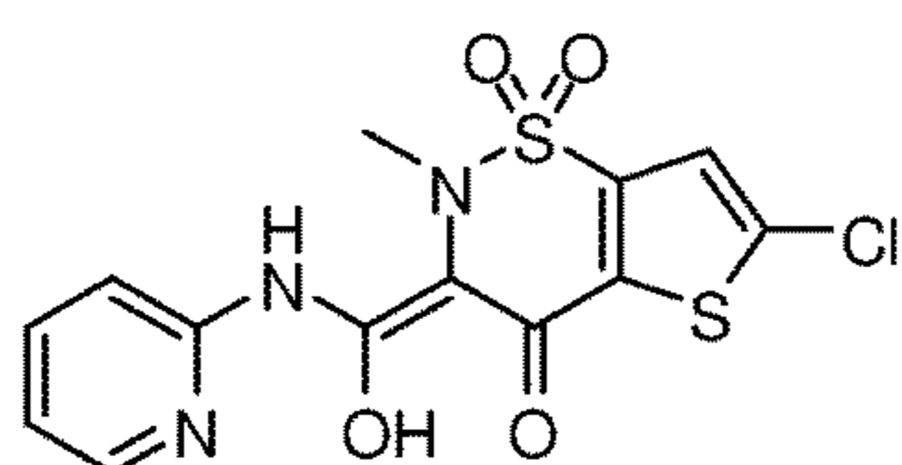
Lornoxicam
