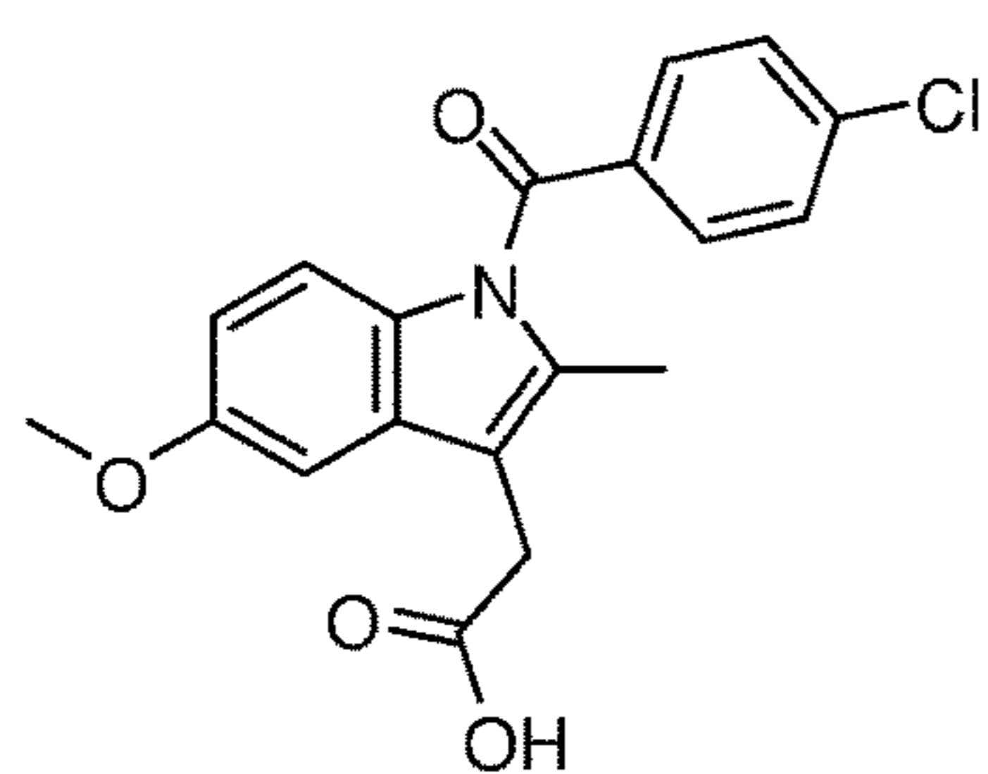
Indomethacin
