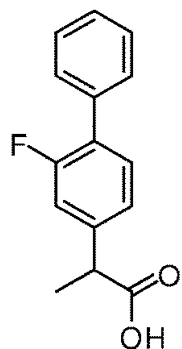
Flurbiprofen
