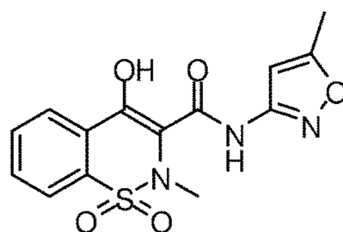
Isoxicam
