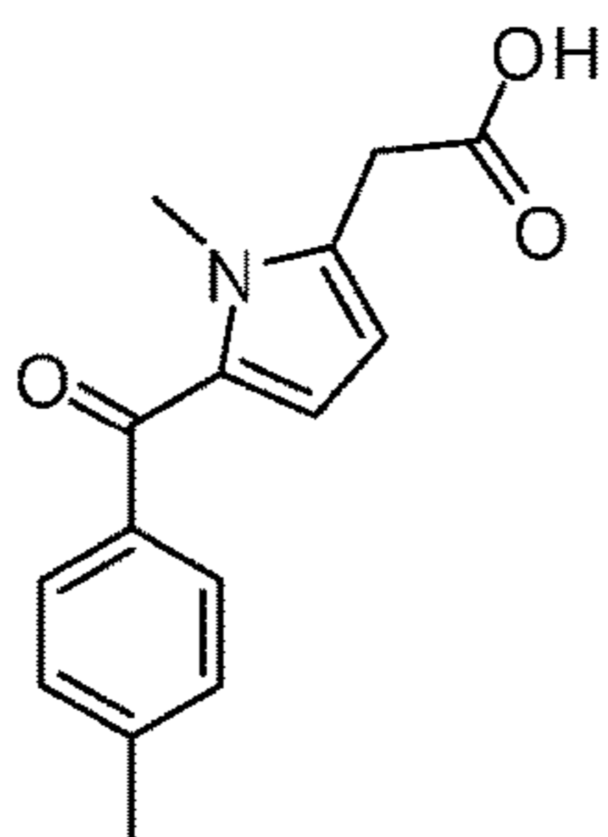
Tolmetin
