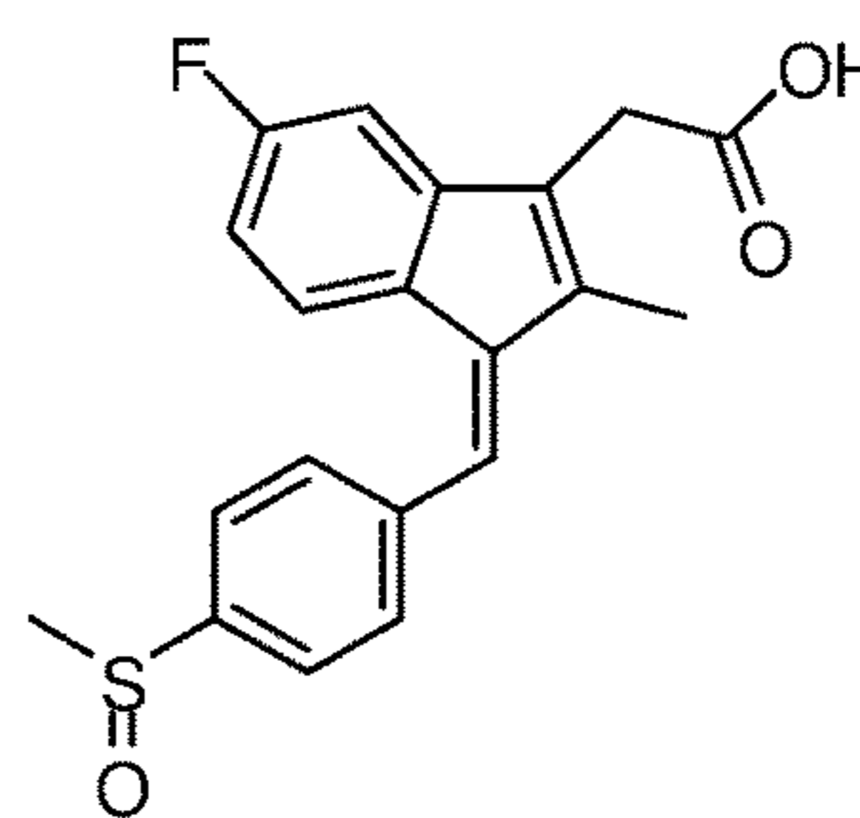
Sulindac
