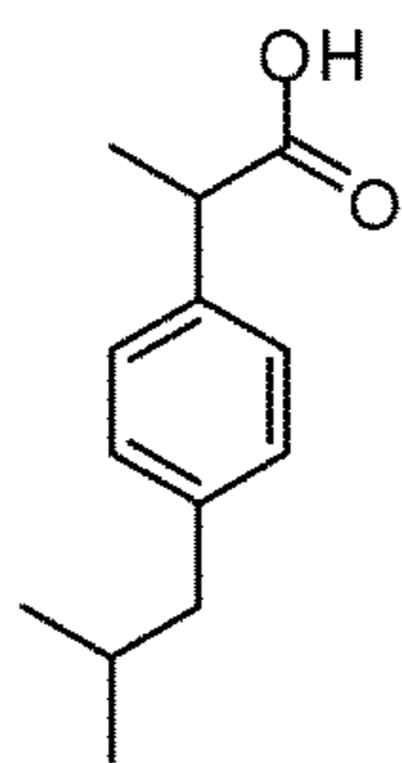
Ibuprofen
