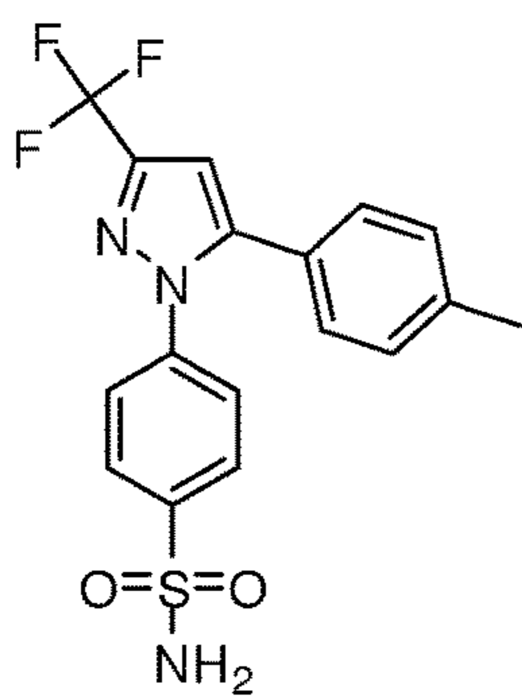
Celecoxib
