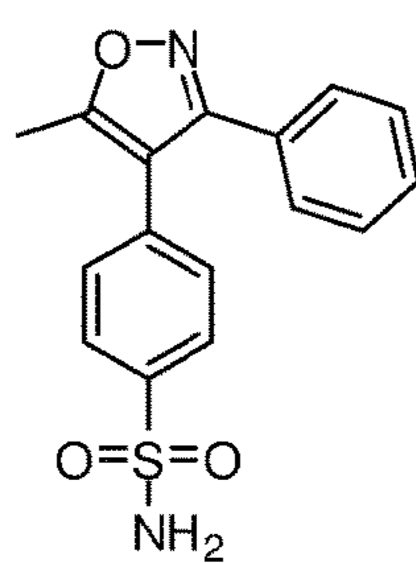
Valdecoxib
