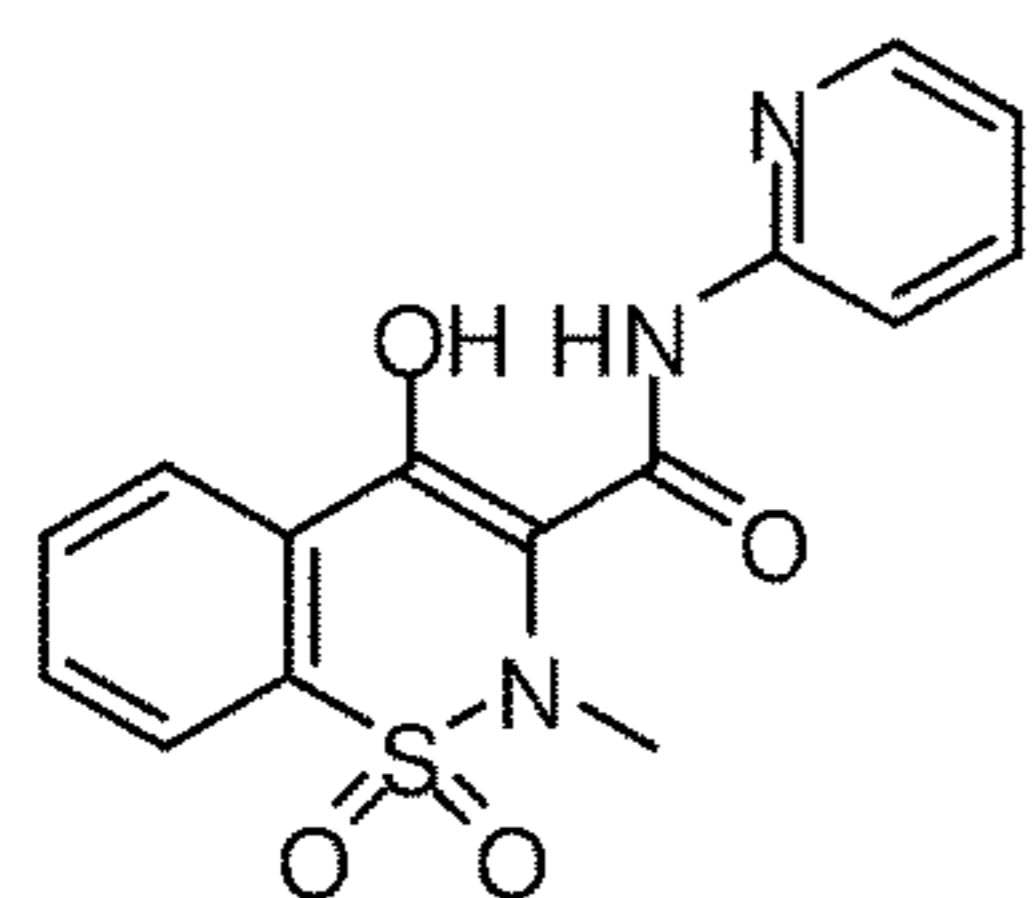
Piroxicam
