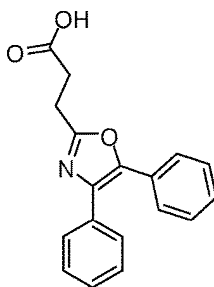
Oxaprozin
