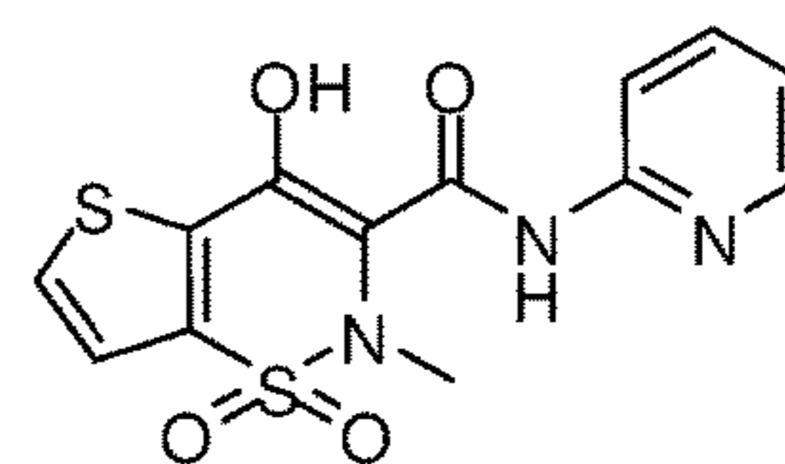
Tenoxicam
