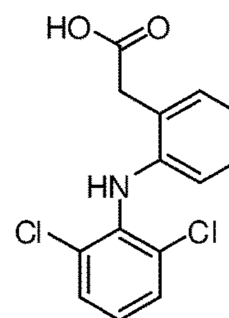
Diclofenac
