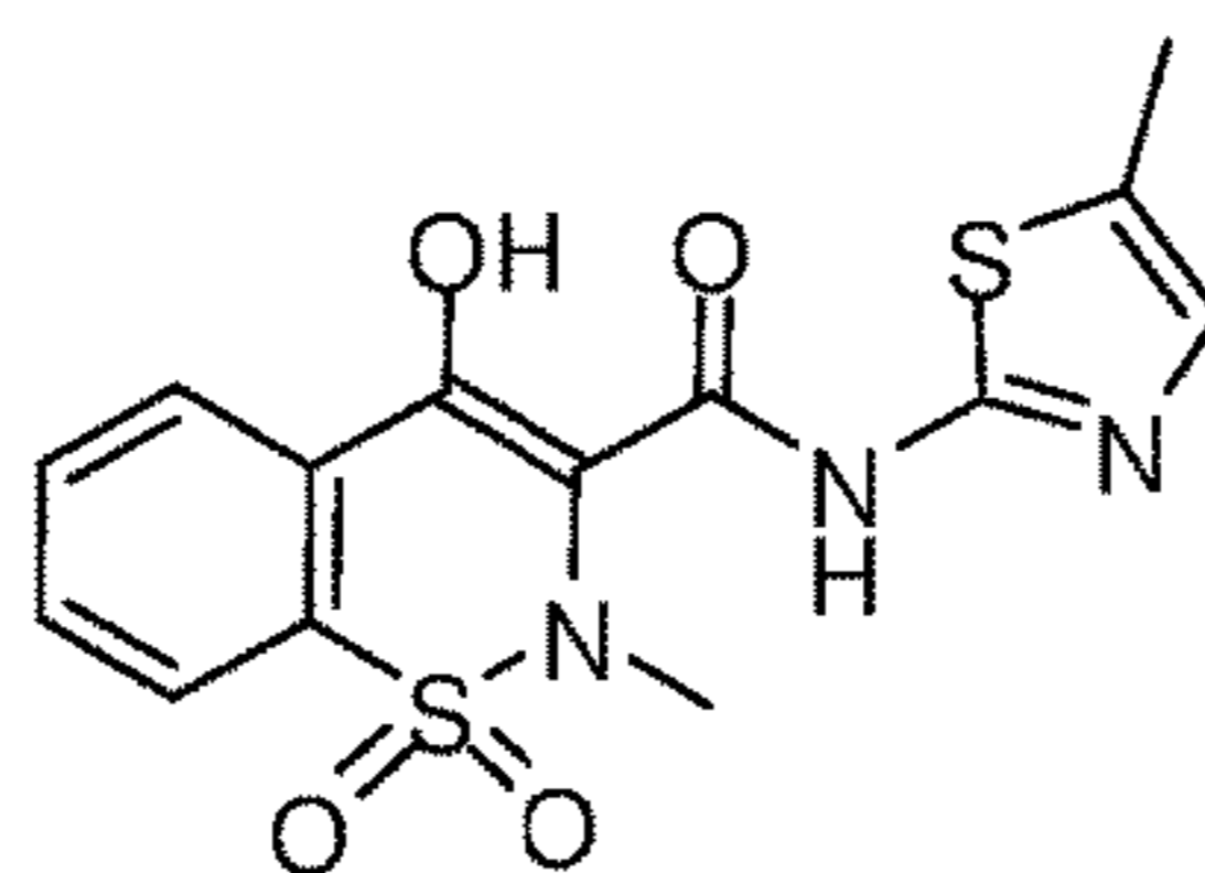
Meloxicam
