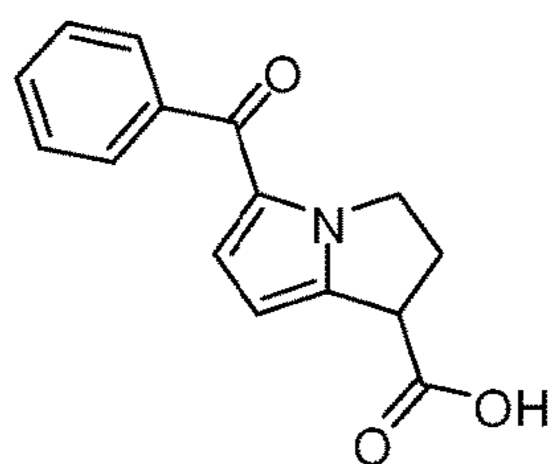
Ketorolac
