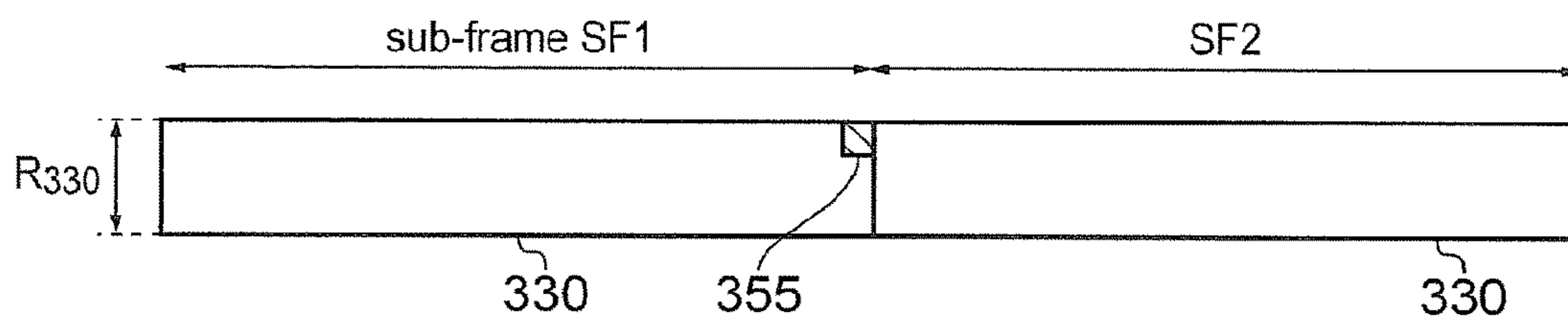
FIG. 11C
