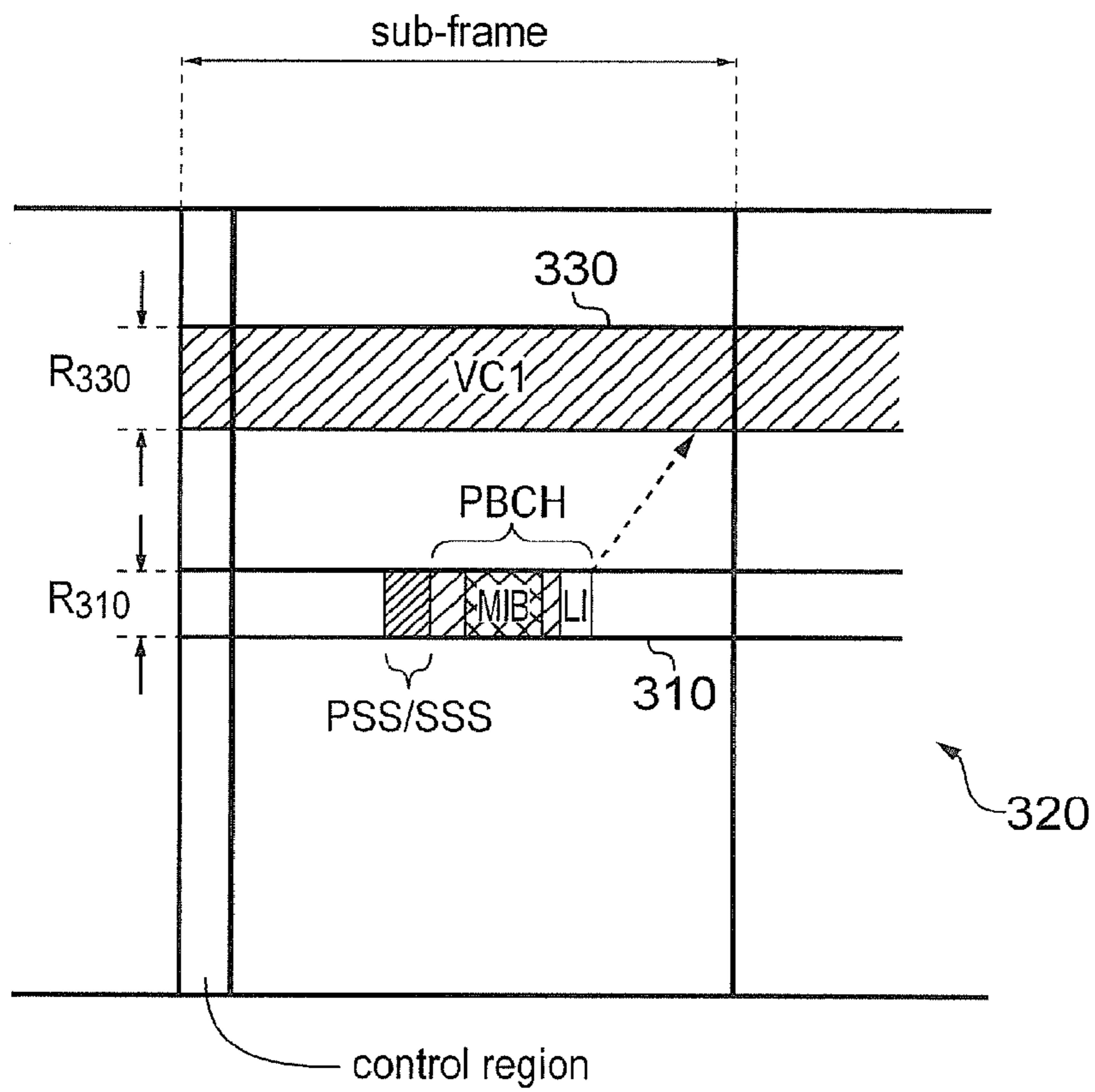
FIG. 9
