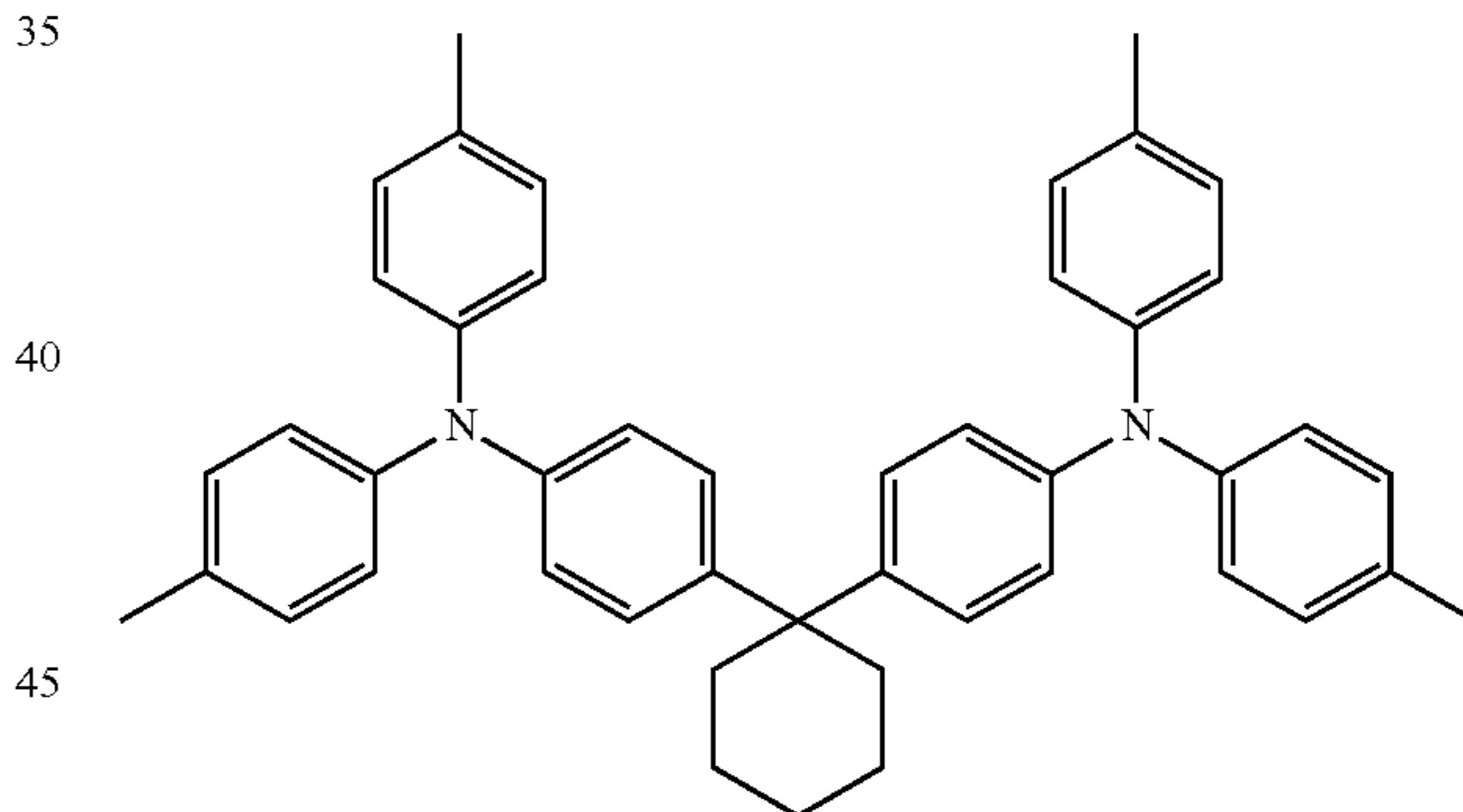
TAPC
