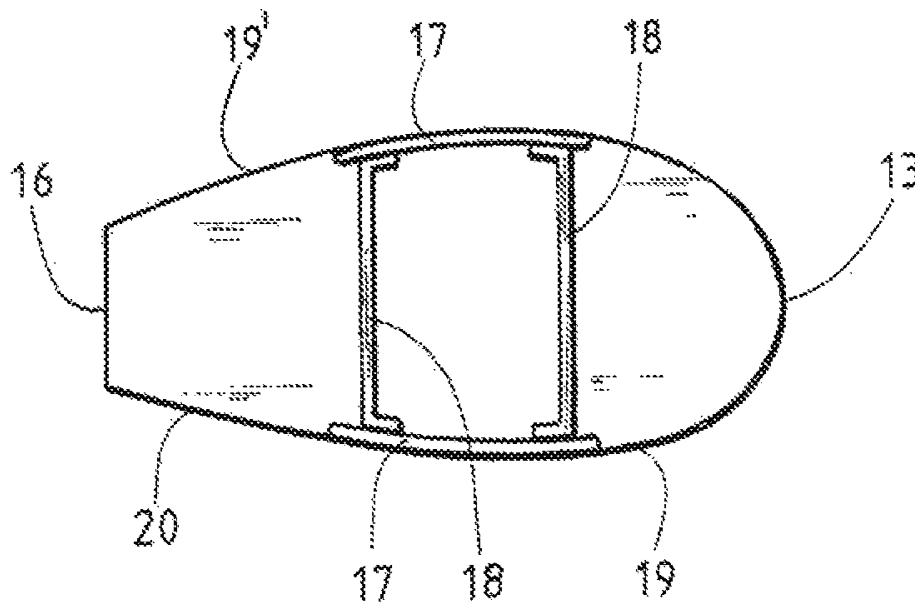
Fig. 2 (A-A)
