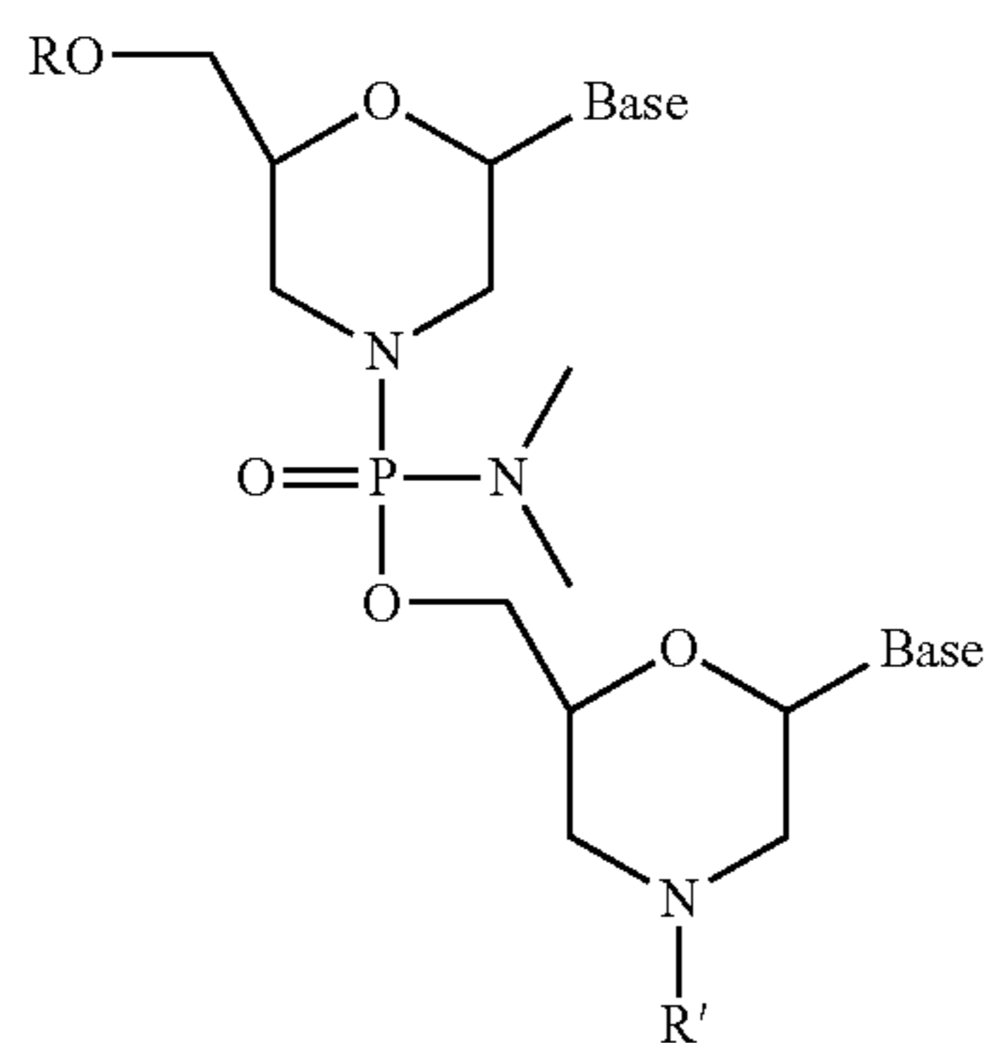
Morpholino
