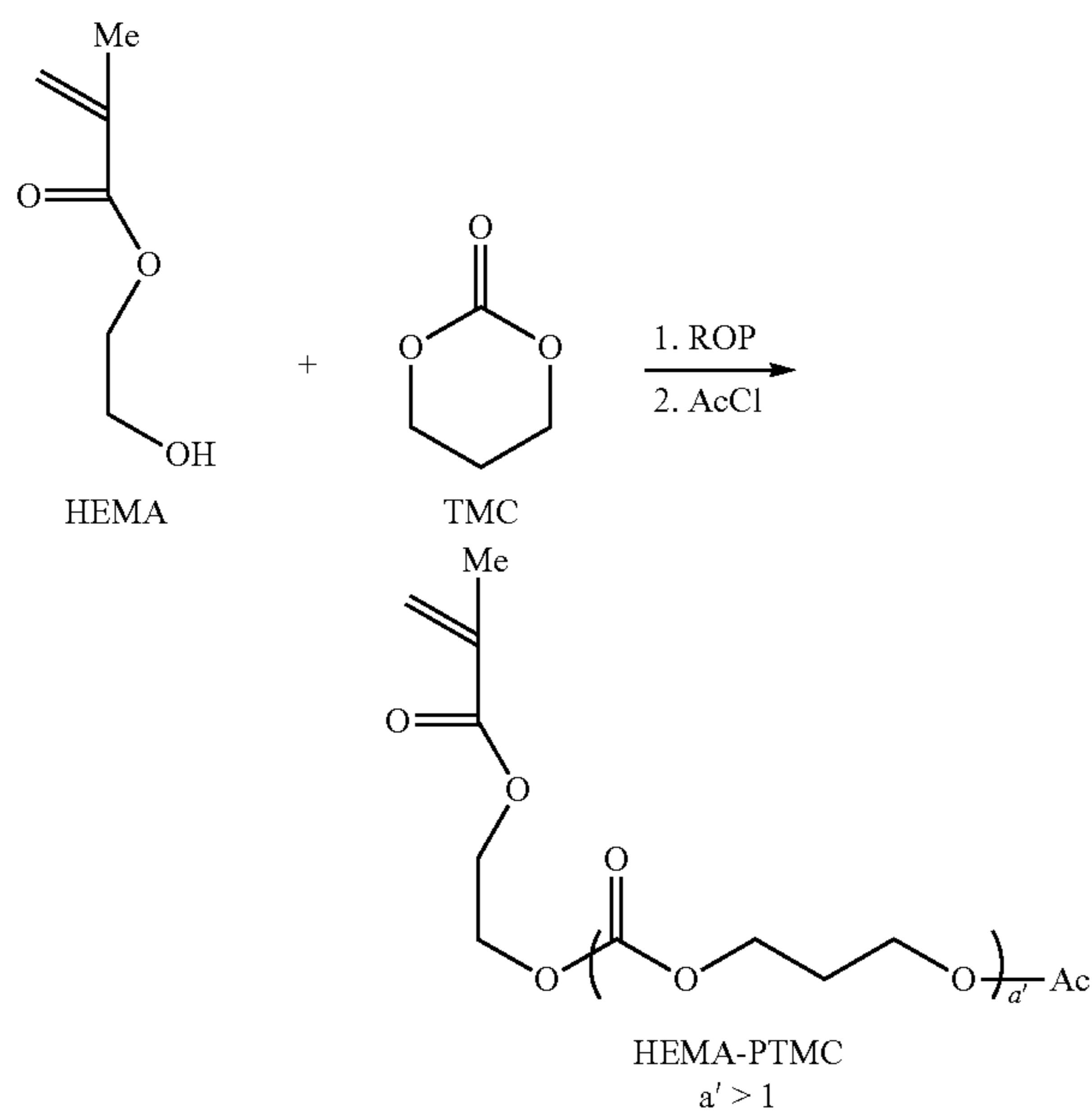
Scheme 17.
