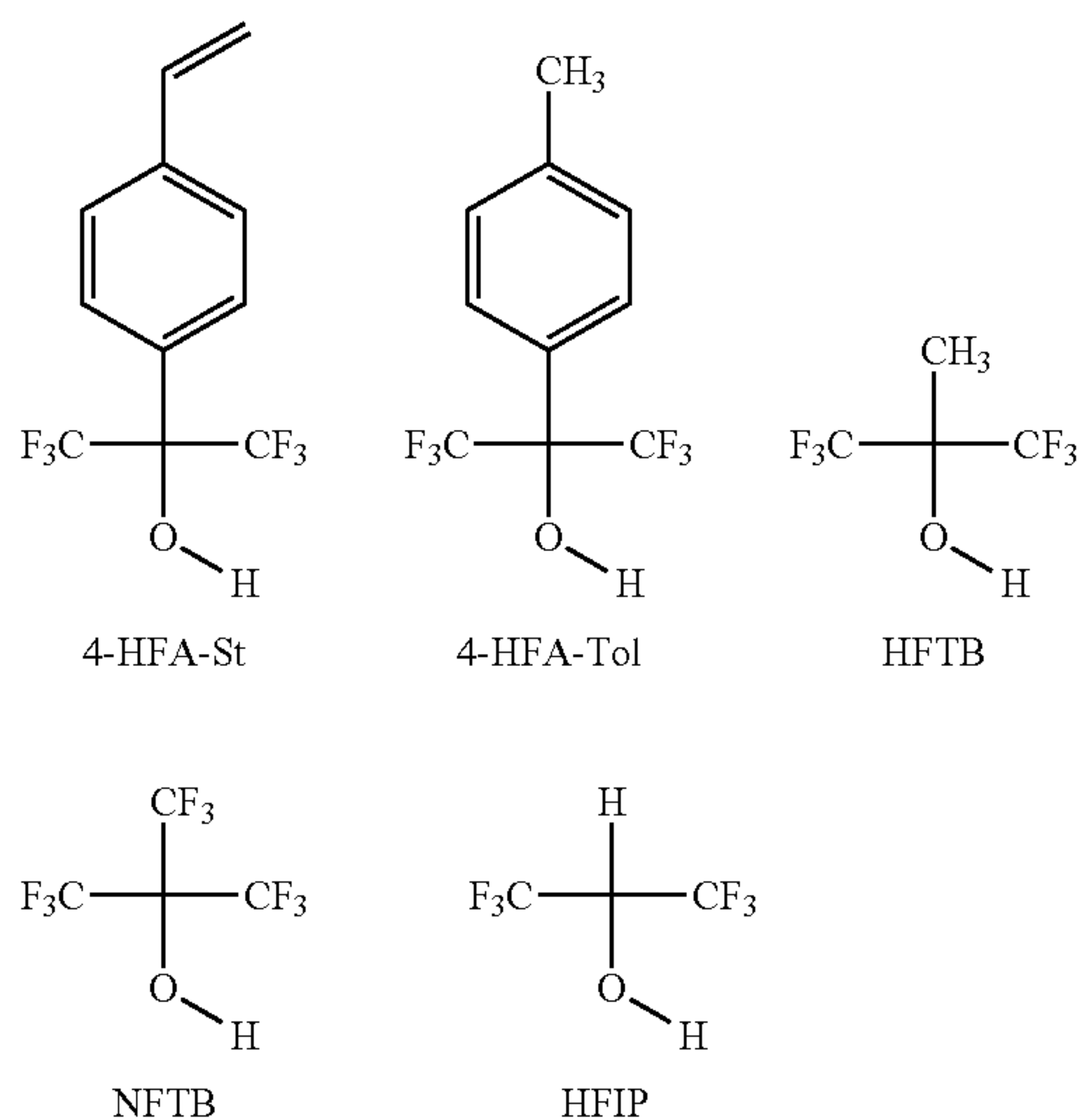
Scheme 23.
