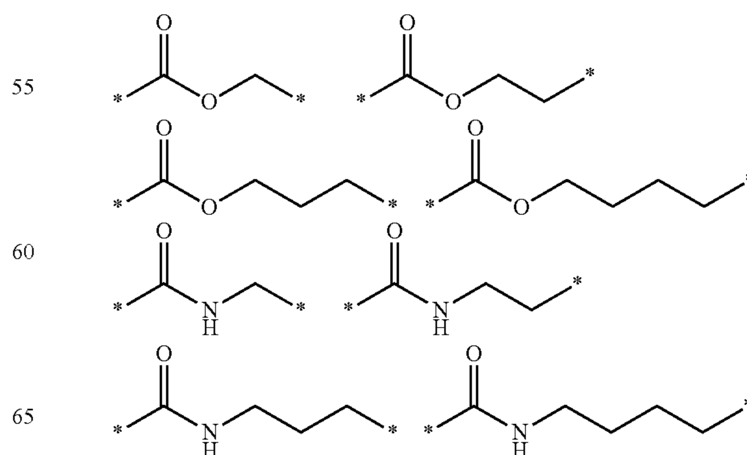
Scheme 14.
