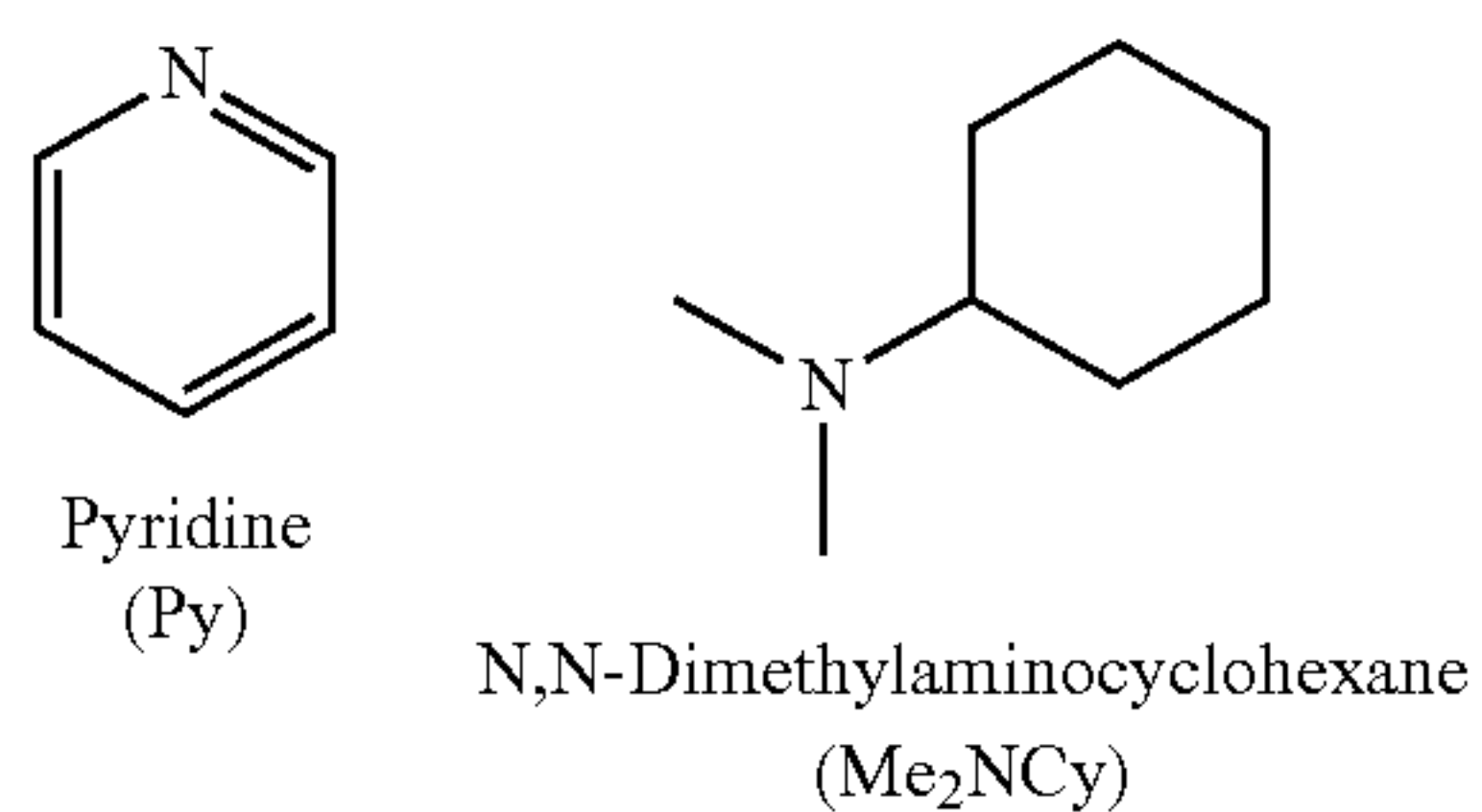
Scheme 25.
