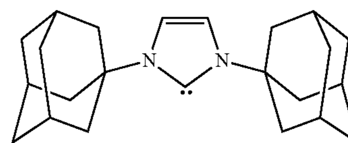
1,3-Bis(1-adamantyl)imidazol-2-ylidene
