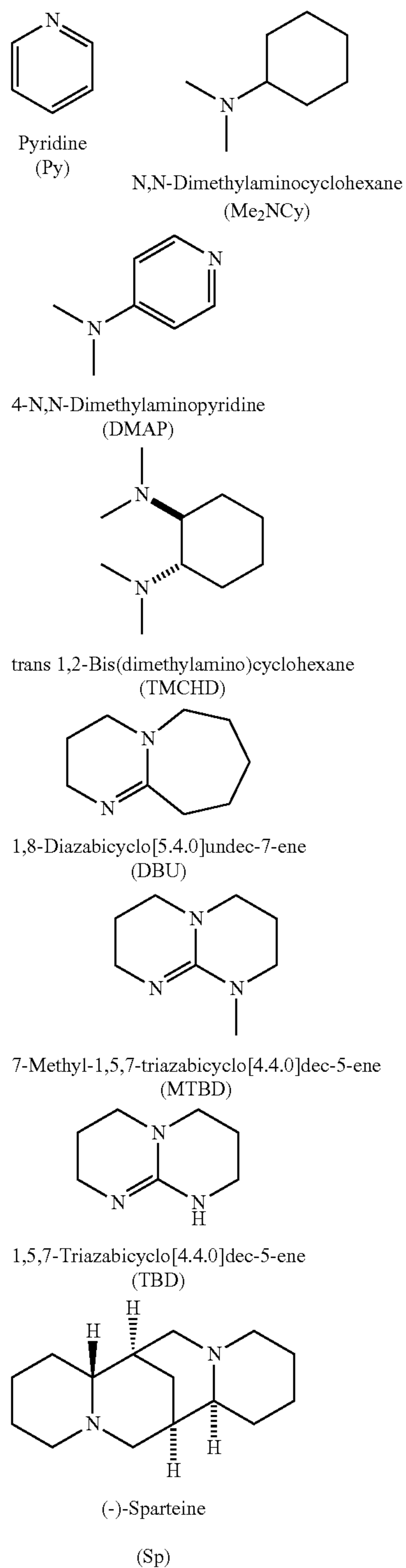
Scheme 25.
