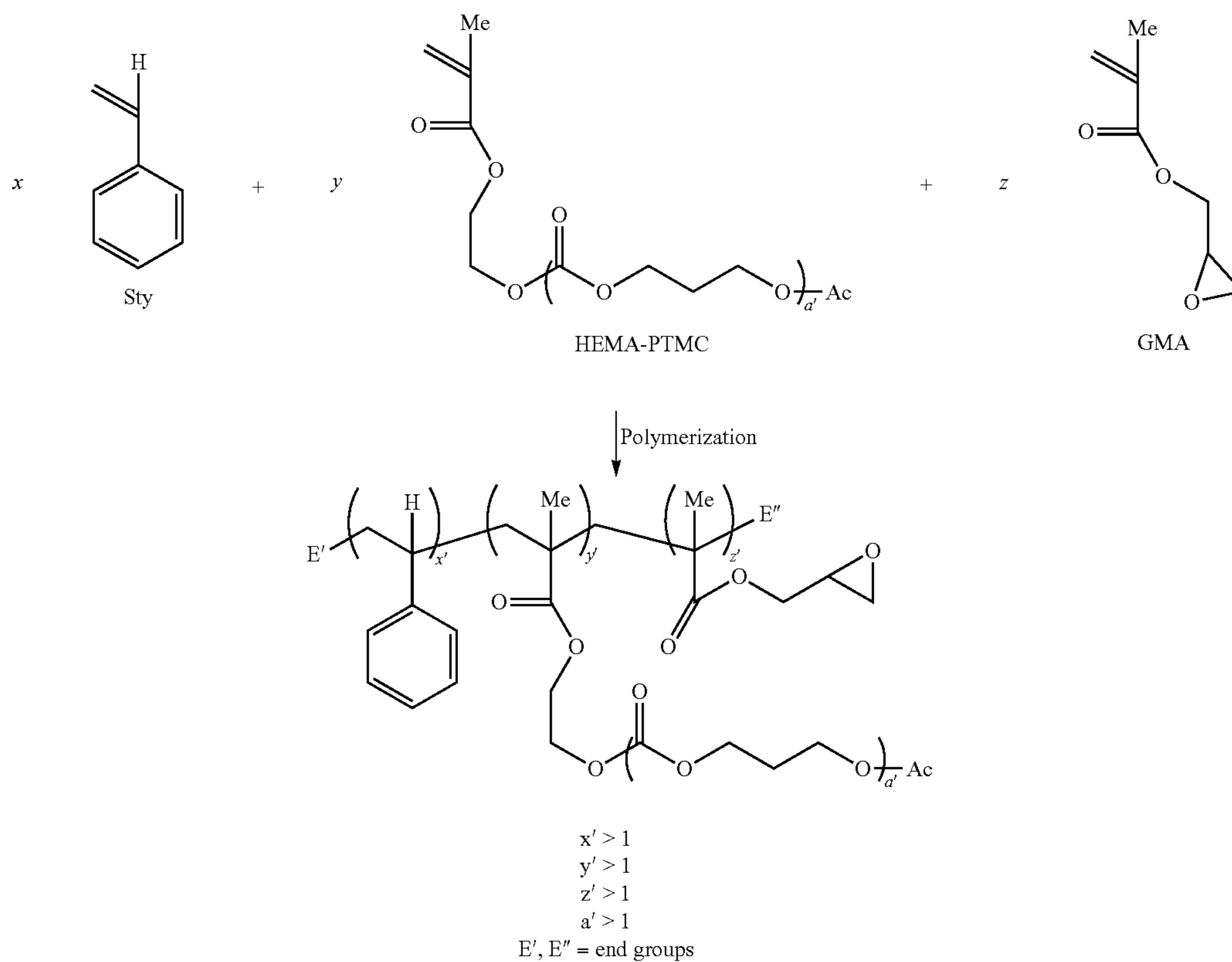
Scheme 16.
