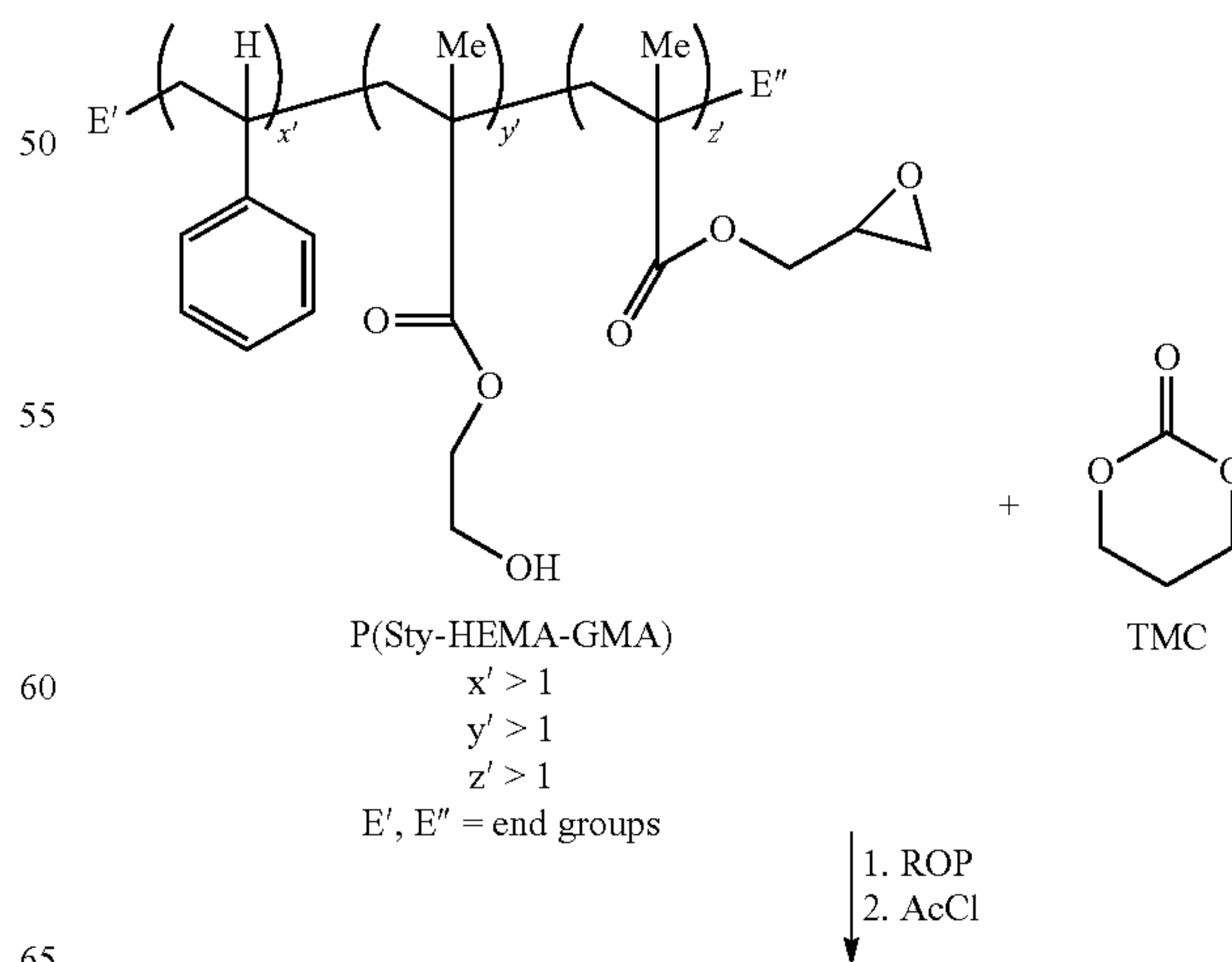
Scheme 18.
