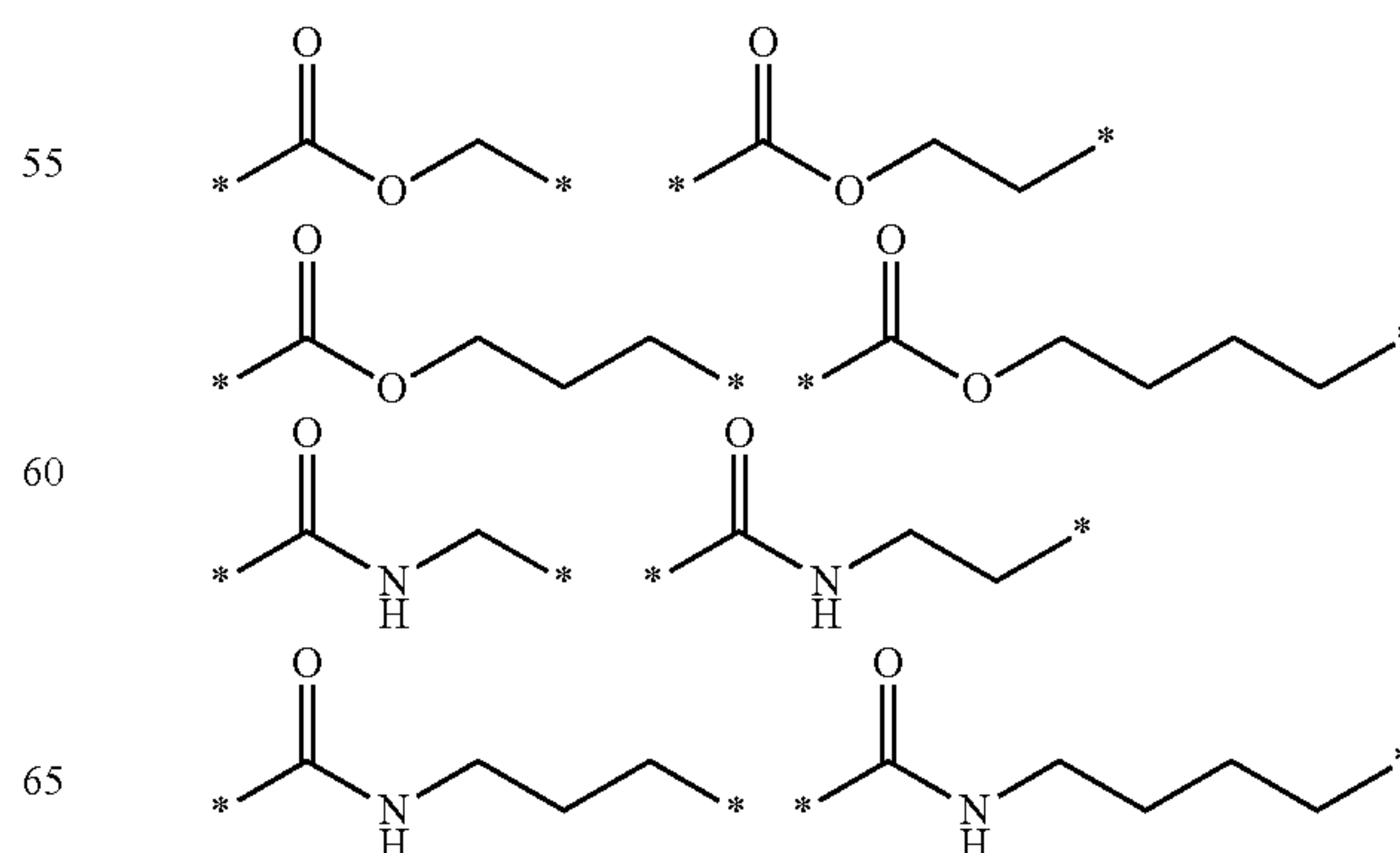
Scheme 14.
