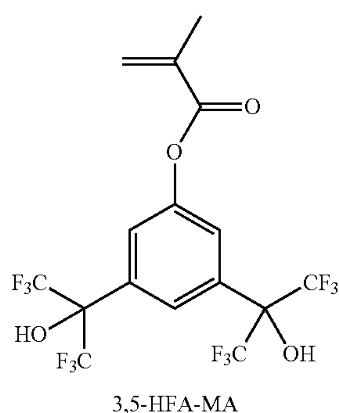
Scheme 24.
