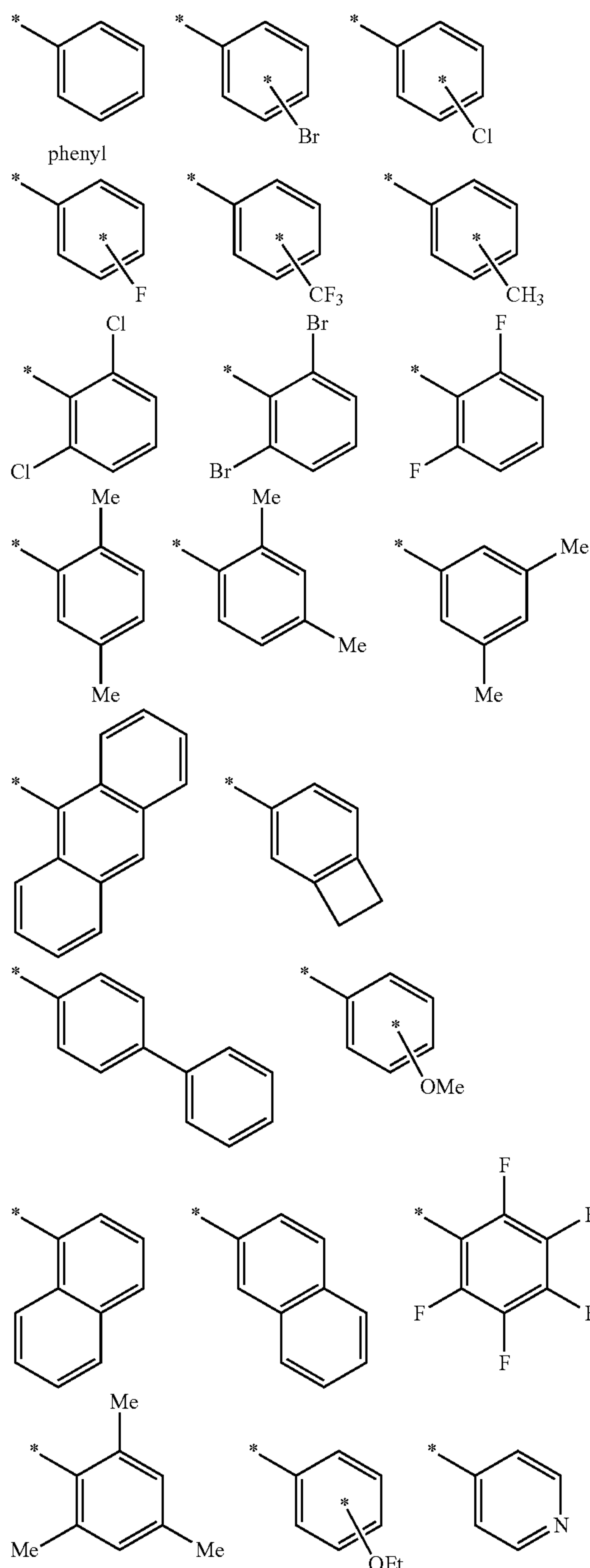
Scheme 19.
