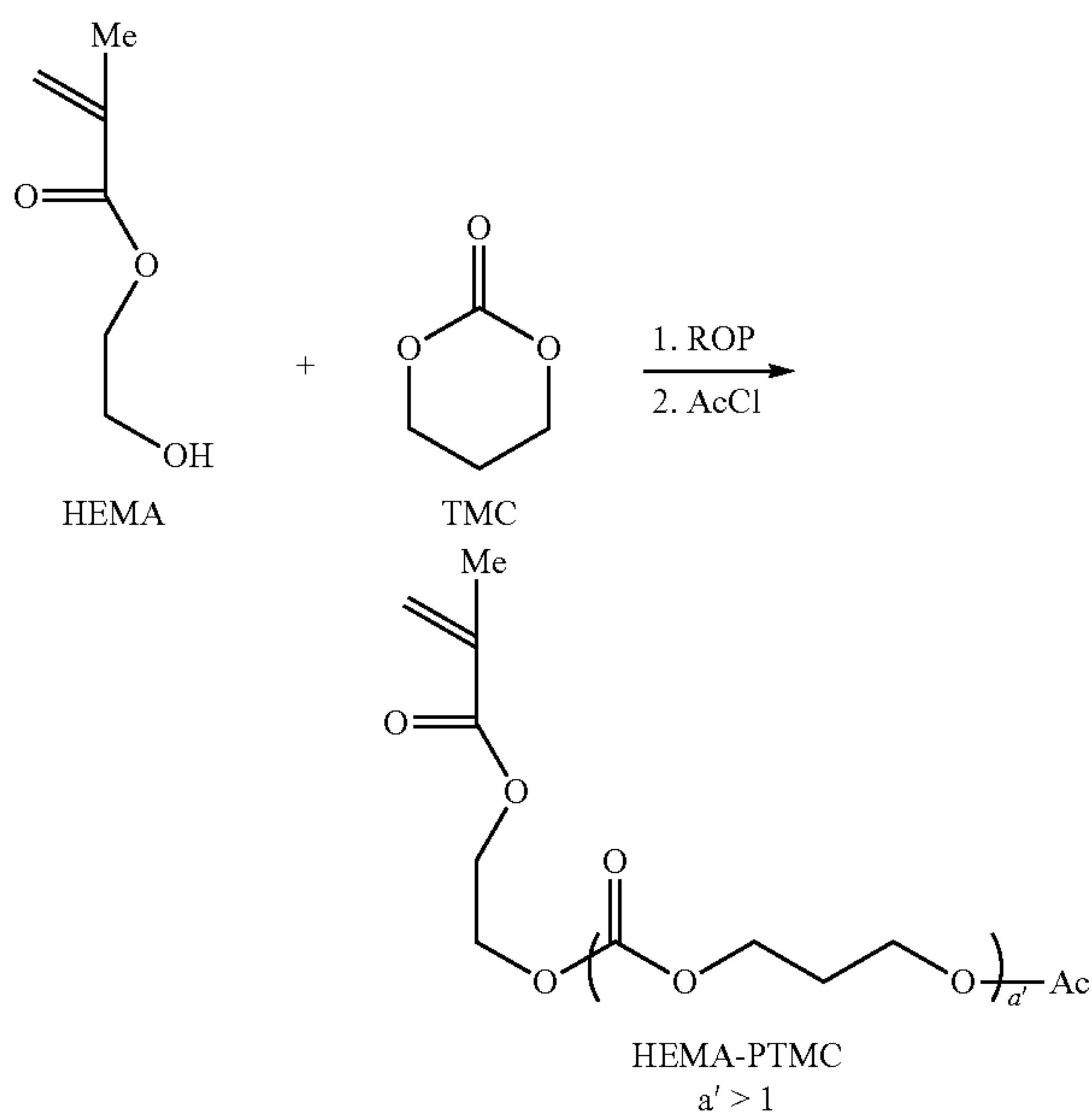
Scheme 17.
