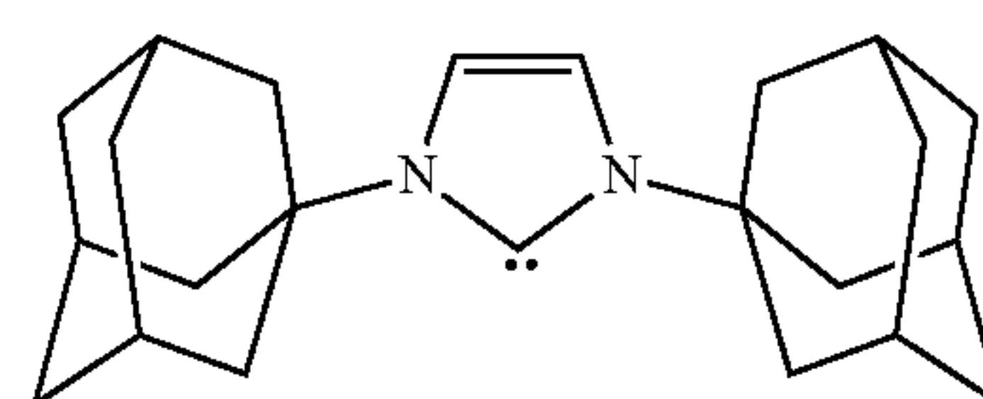
1,3-Bis(1-adamantyl)imidazol-2-ylidene
