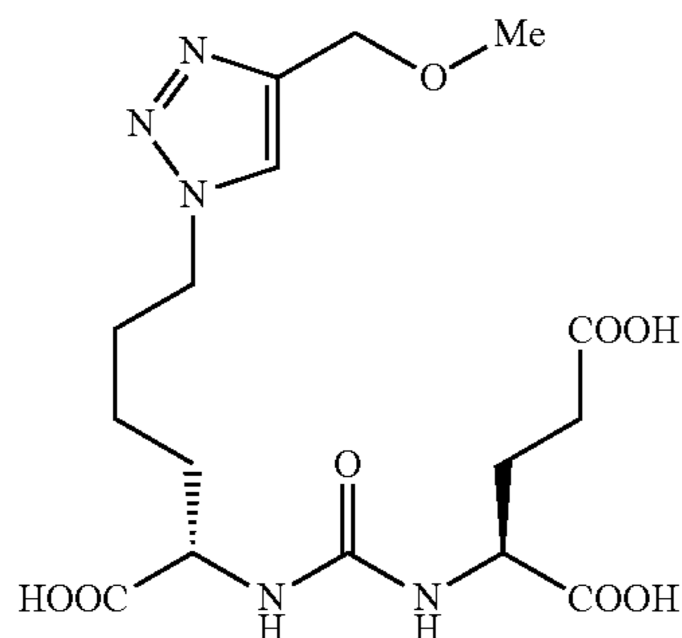
(S)-2-(3-((S)-1-carboxy-5-(4-(methoxymethyl)-1H-1,2,3-triazol-1-yl)pentyl)ureido)pentanedioic acid (8)
