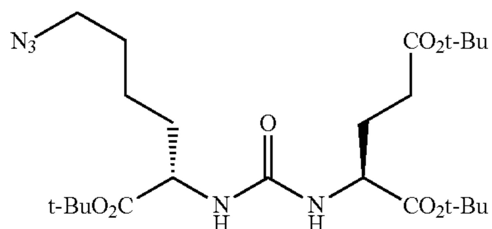
(S)-di-tert-butyl 2-(3-((S)-6-azido-1-tert-butoxy-1-oxohexan-2-yl)ureido)pentanedioate (14)
