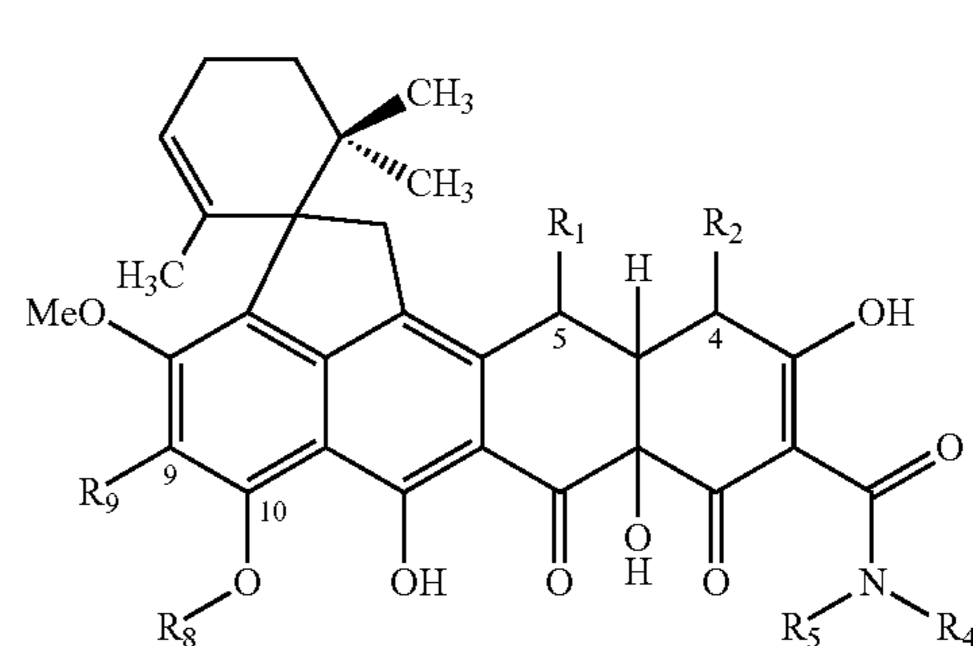
(V)
