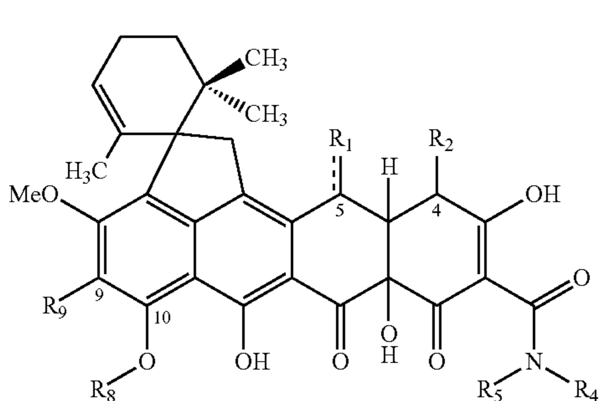
(IV)
