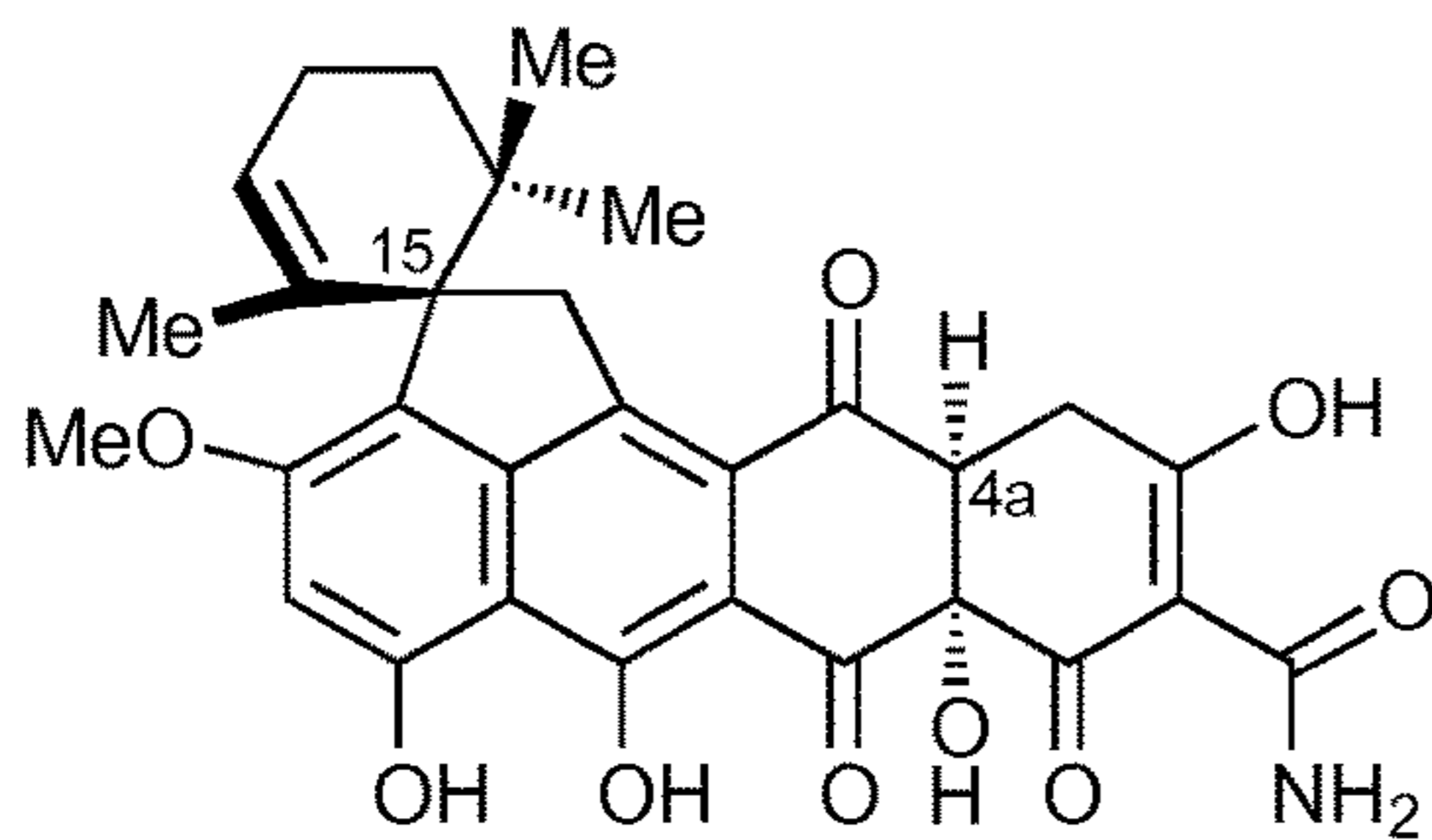
(±)-V2
