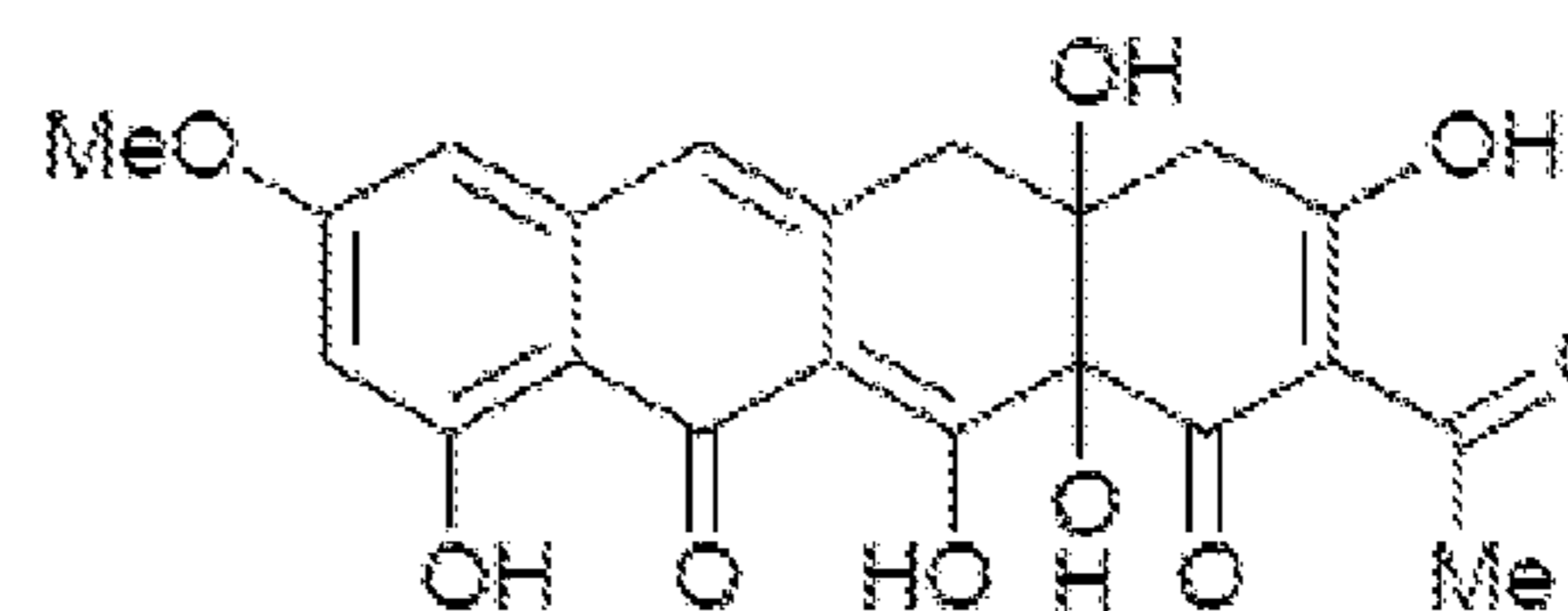
14: BMS-192548
