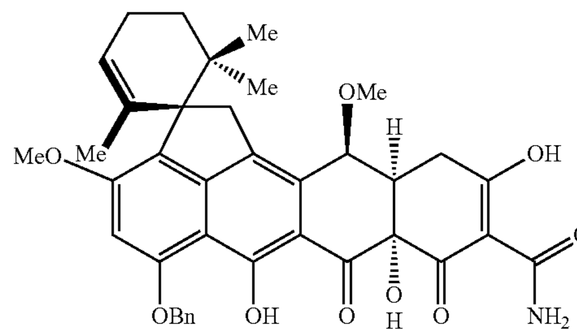
V6
