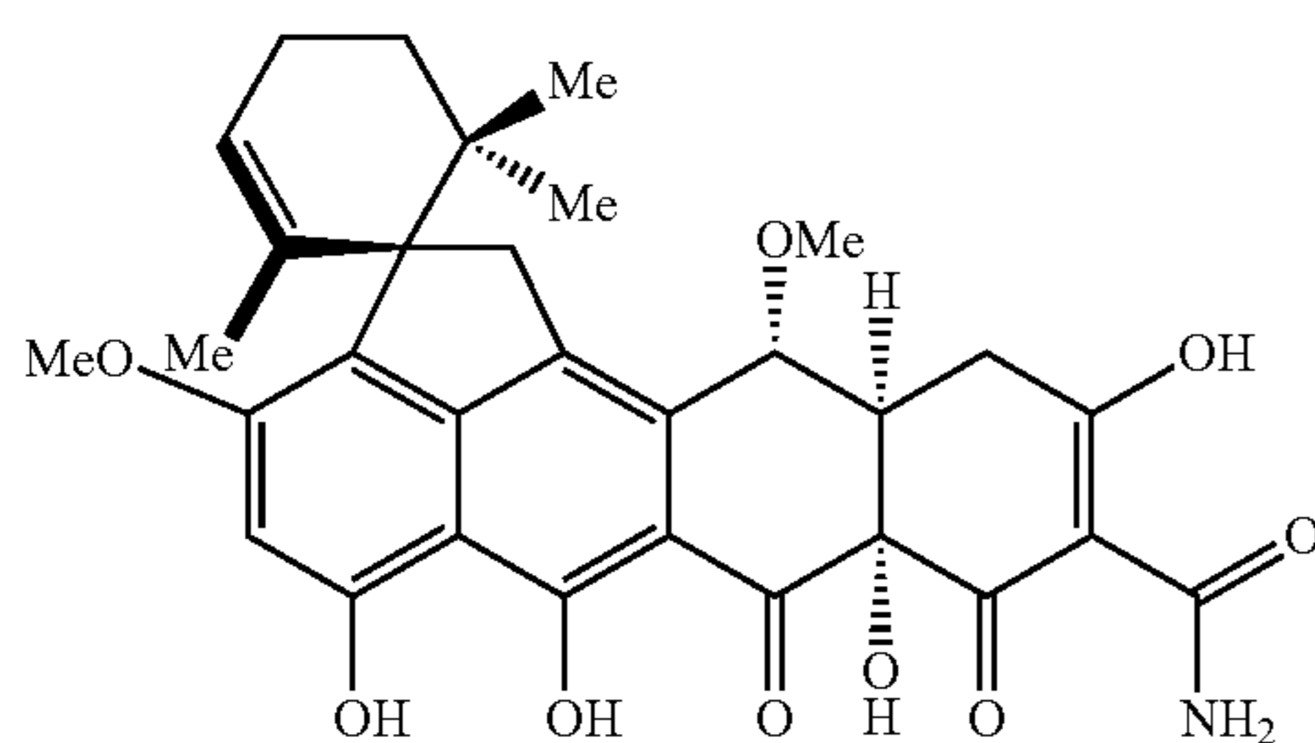
V5
