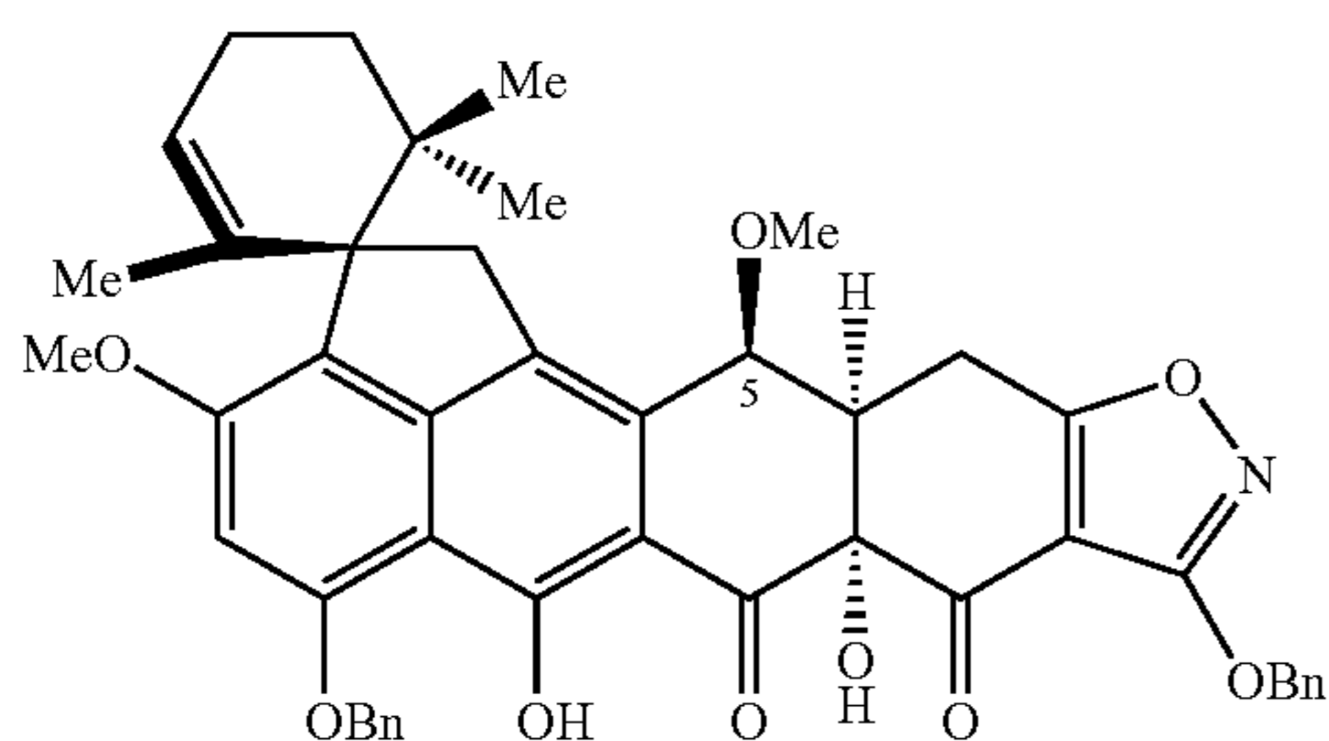
5-epi-15
