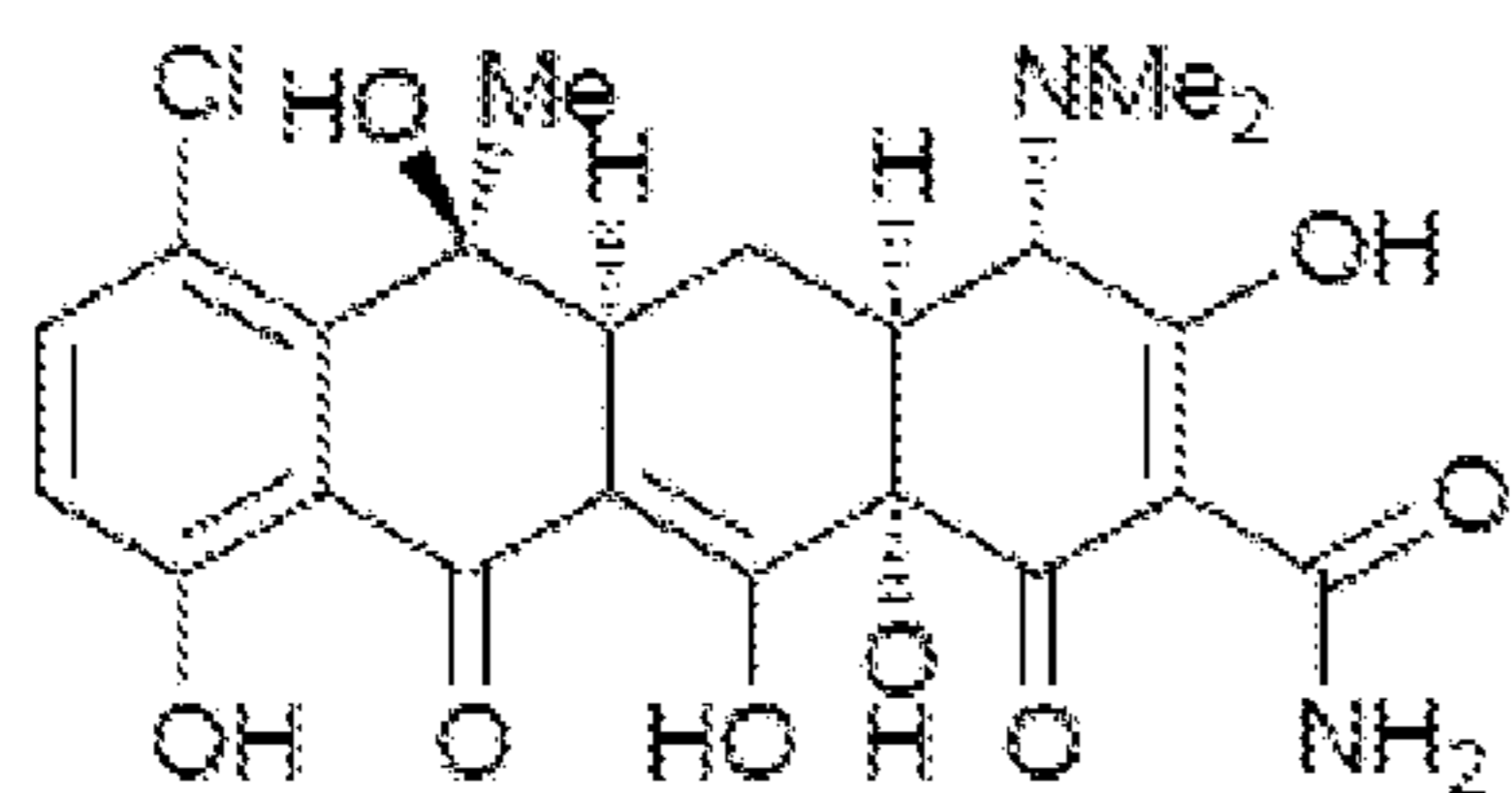
4: chlortetracycline (Aureomycin®)
