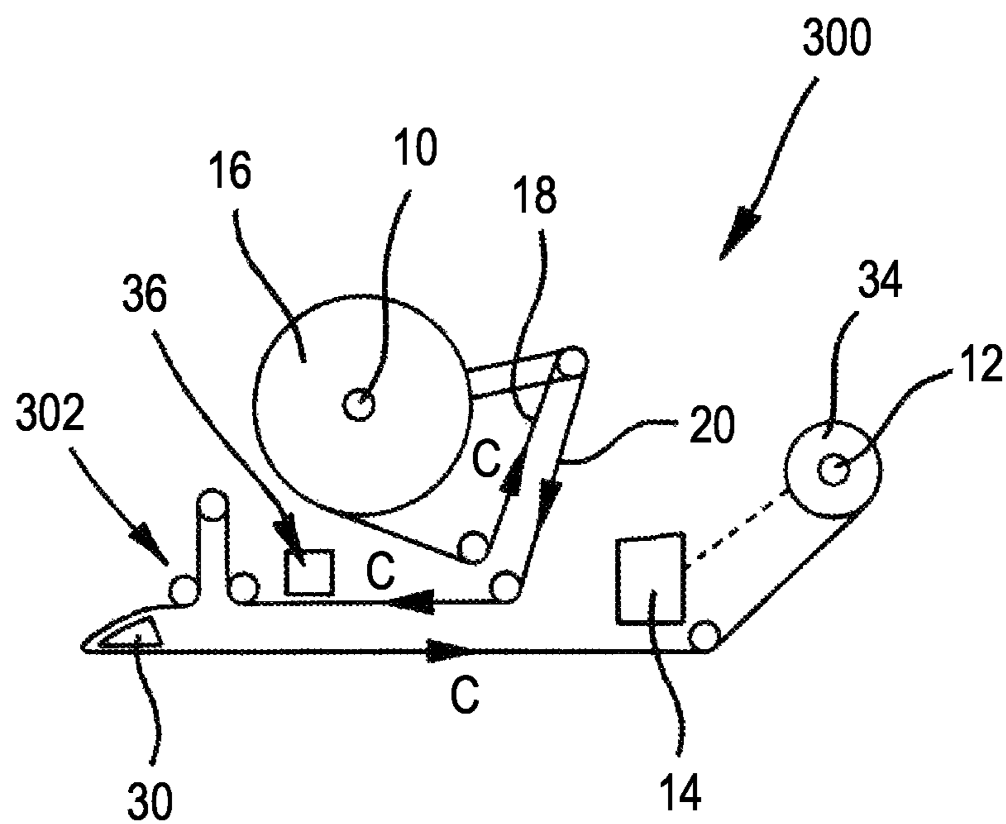
Fig. 28
