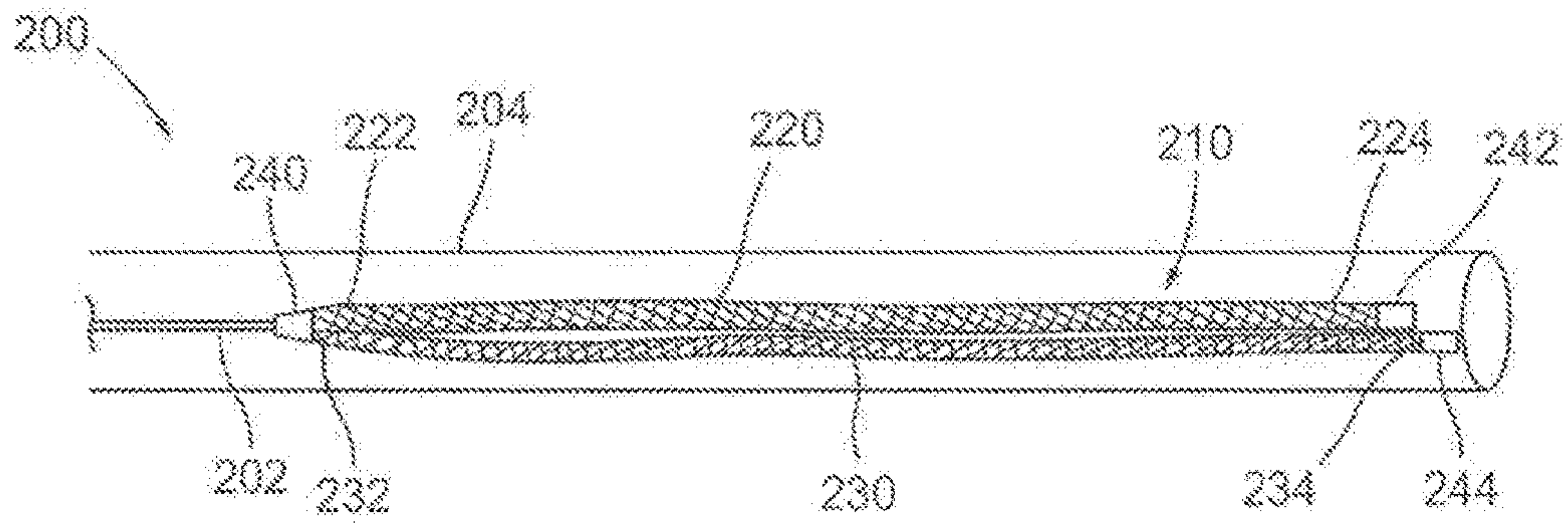
FIG. 5A
