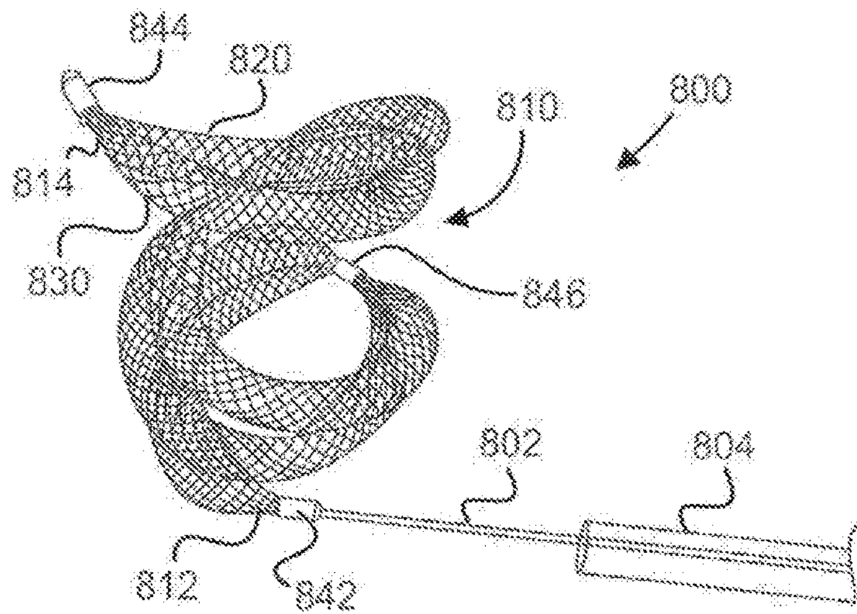
FIG. 11
