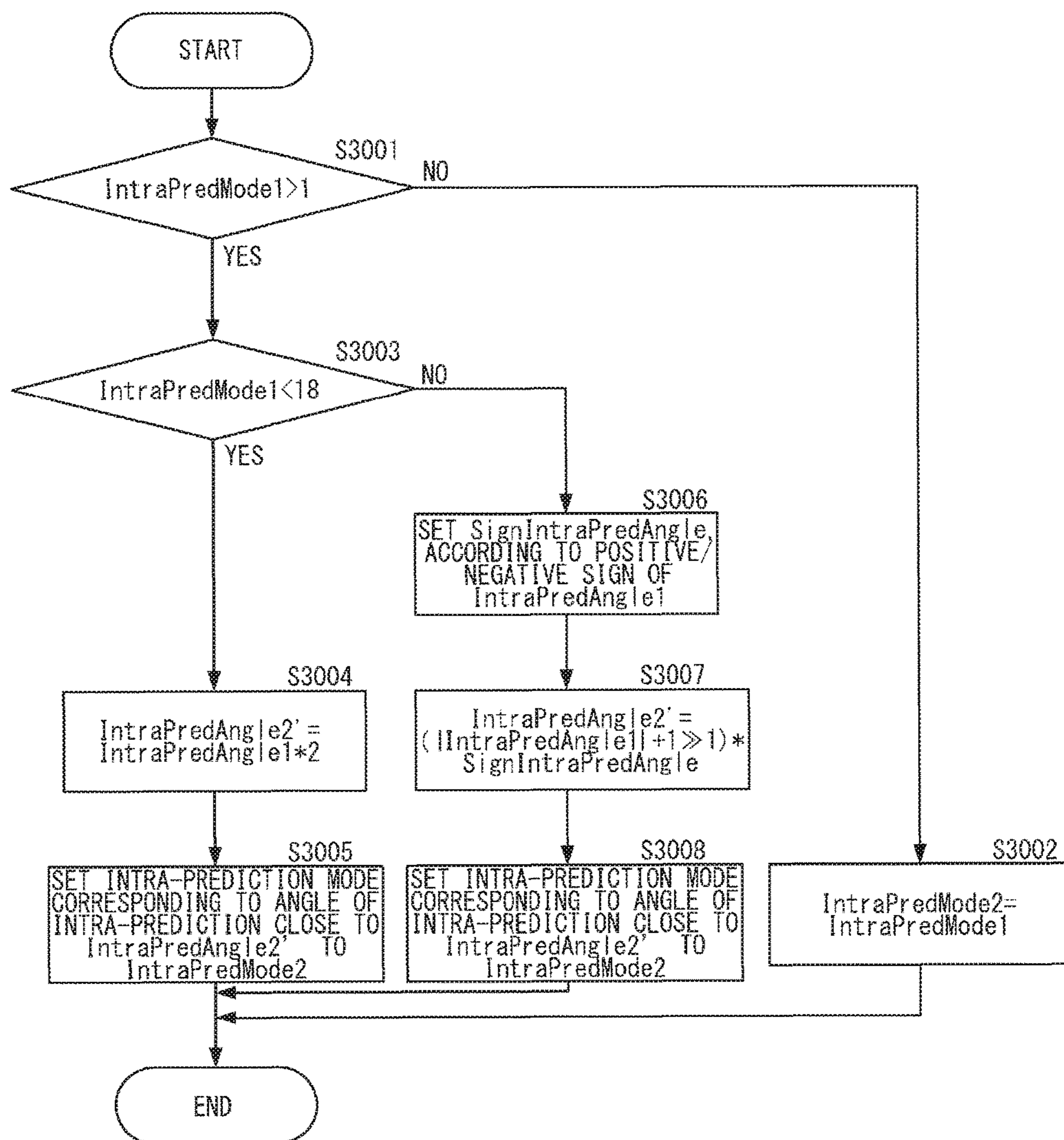
FIG.23
