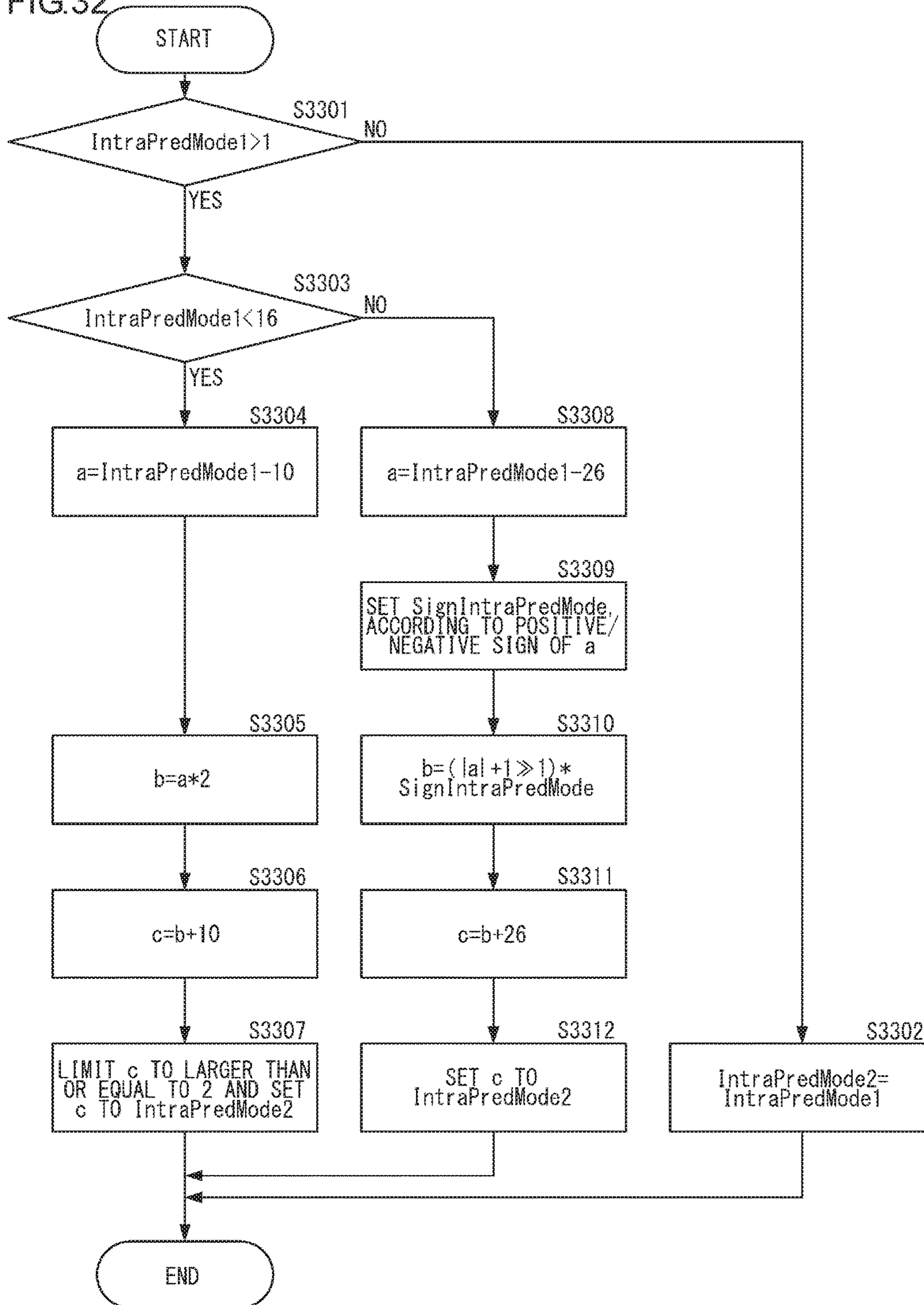
FIG.32
