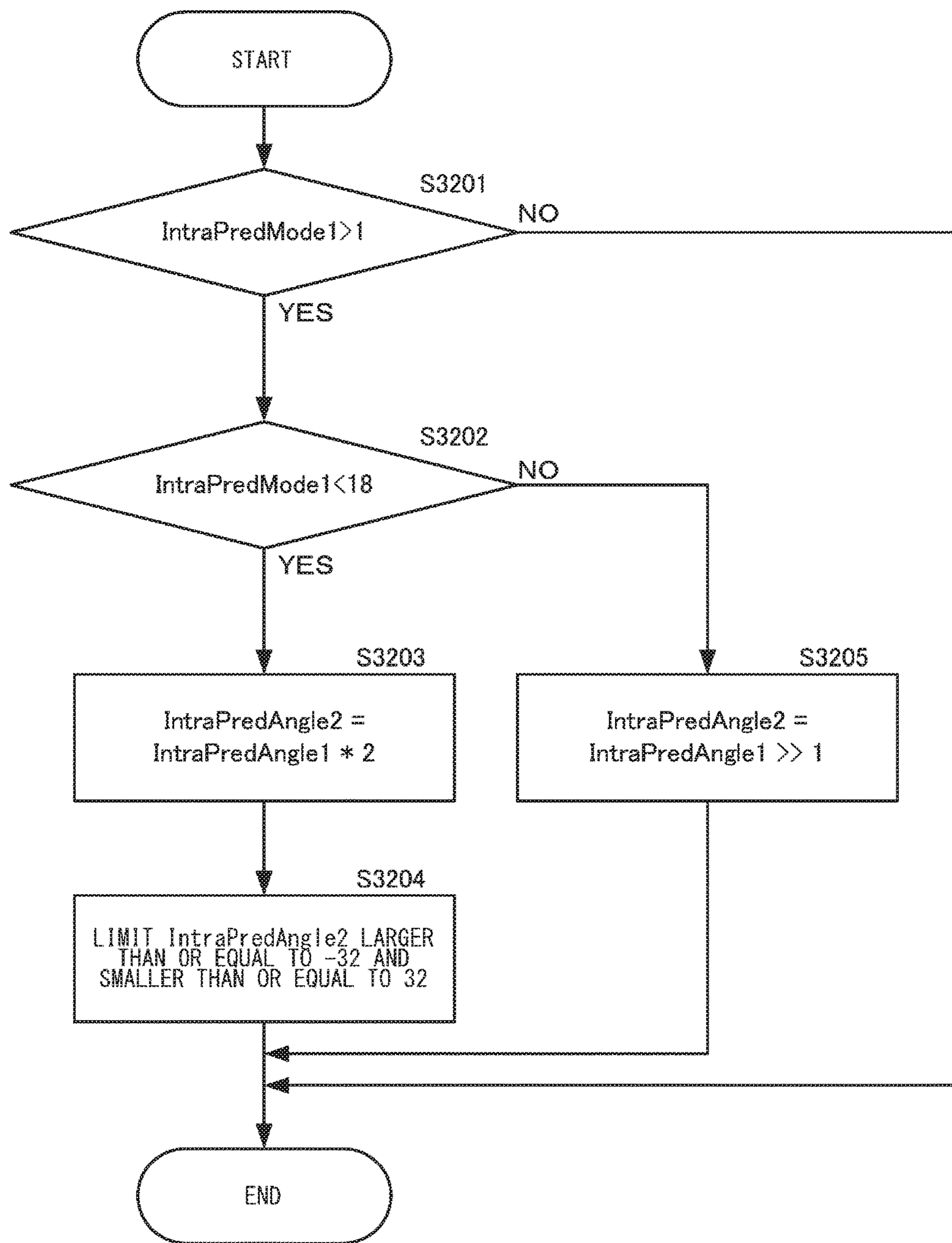
FIG.29
