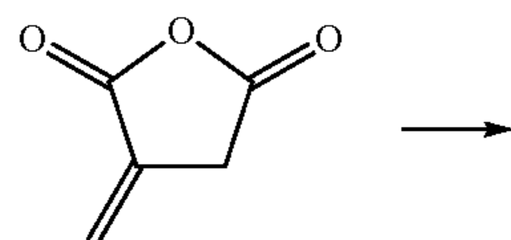
Itaconic anhydride
