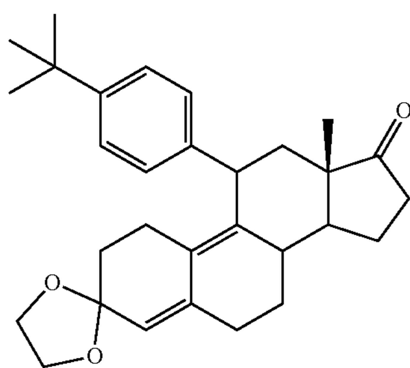
3,3-Ethylendioxy-11 \beta -[4-p-(t-butyl)phenyl]estra-4,9-dien-17-one (4f)
