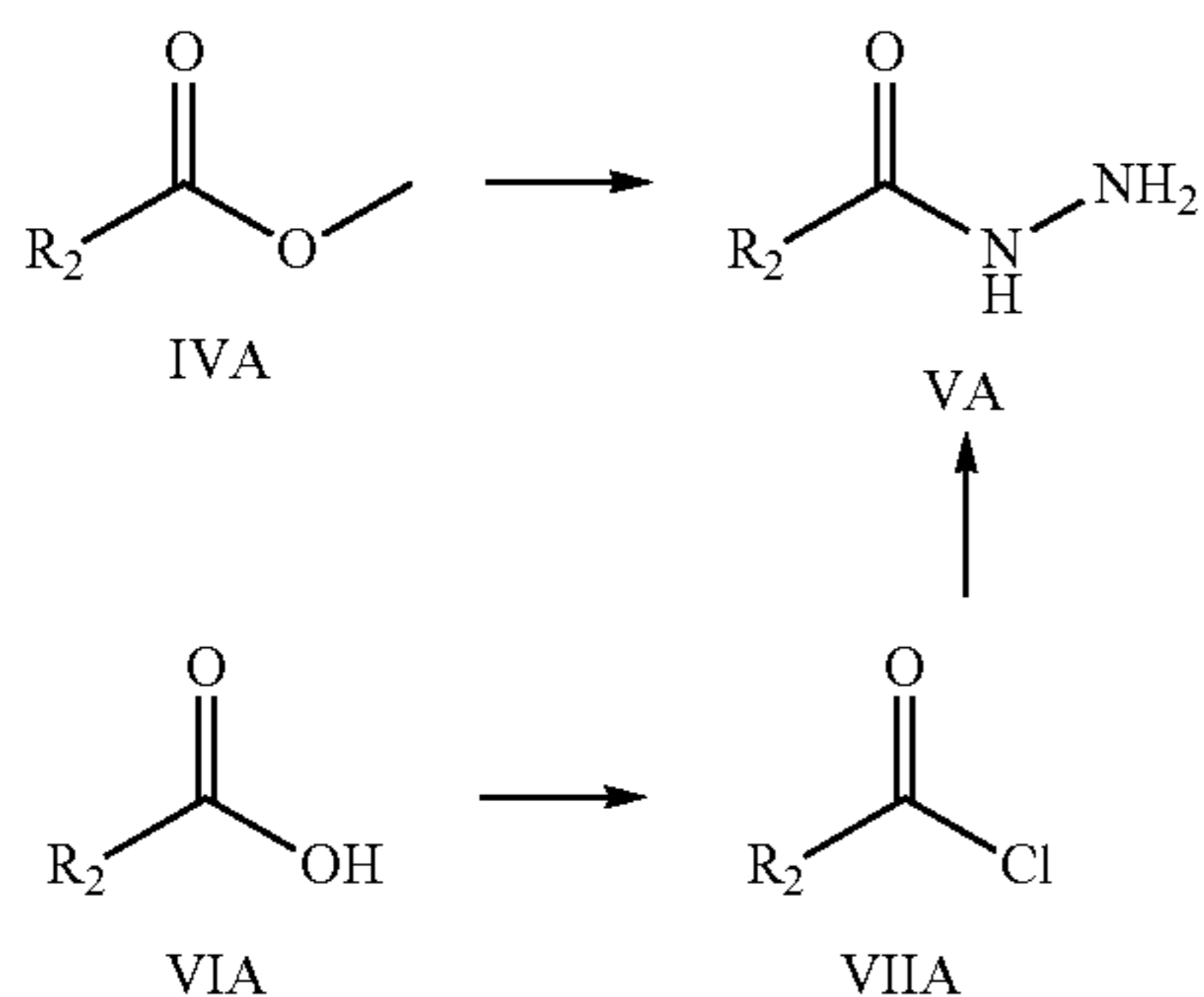
Scheme 2A
