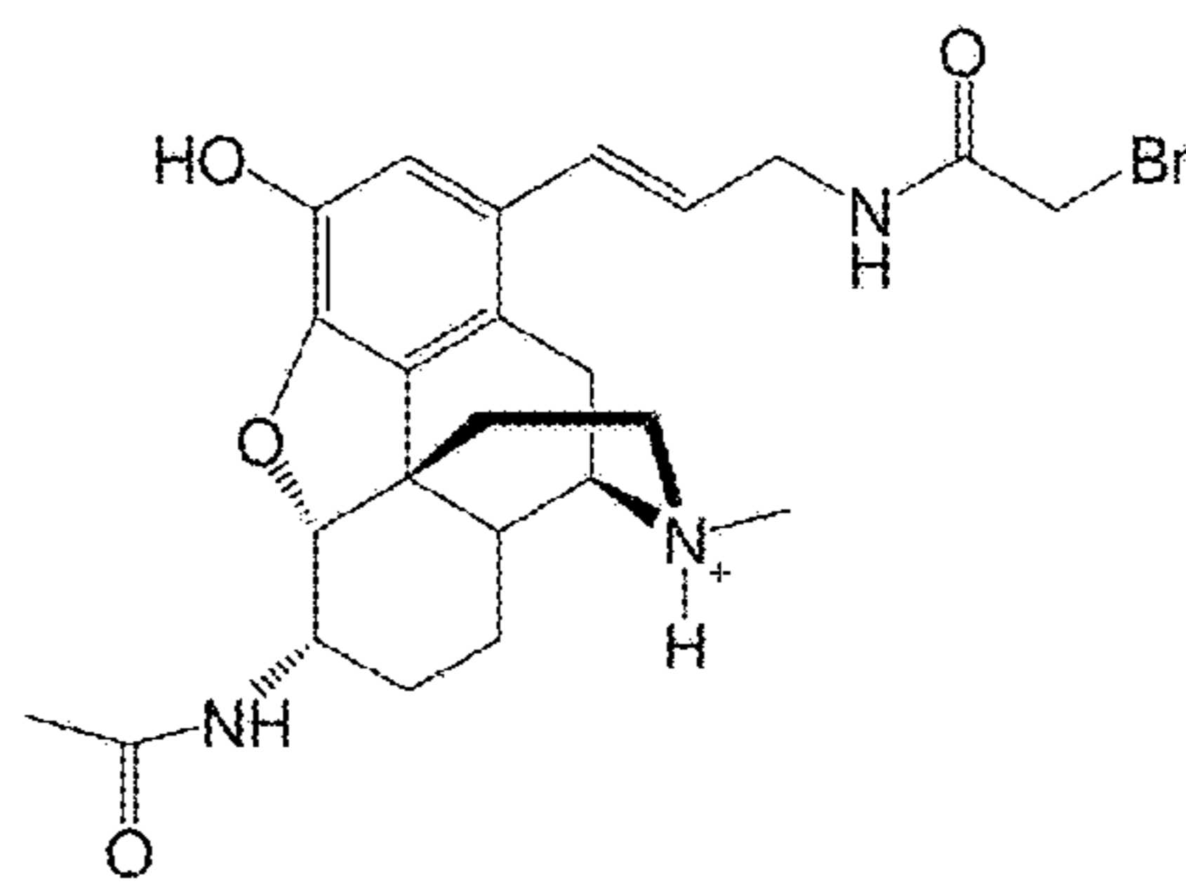
1-Aminopropenyl-N-Bromoacetyl-6-AHM
