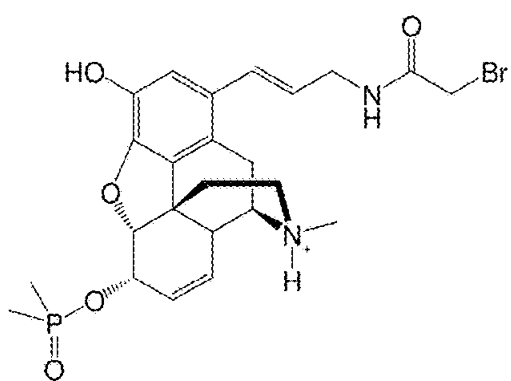
1-Aminopropenyl-N-Bromoacetyl-6PM
