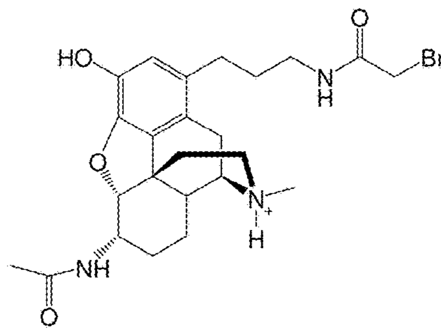
1-Aminopropenyl-N-Bromoacetyl-6-AHM
