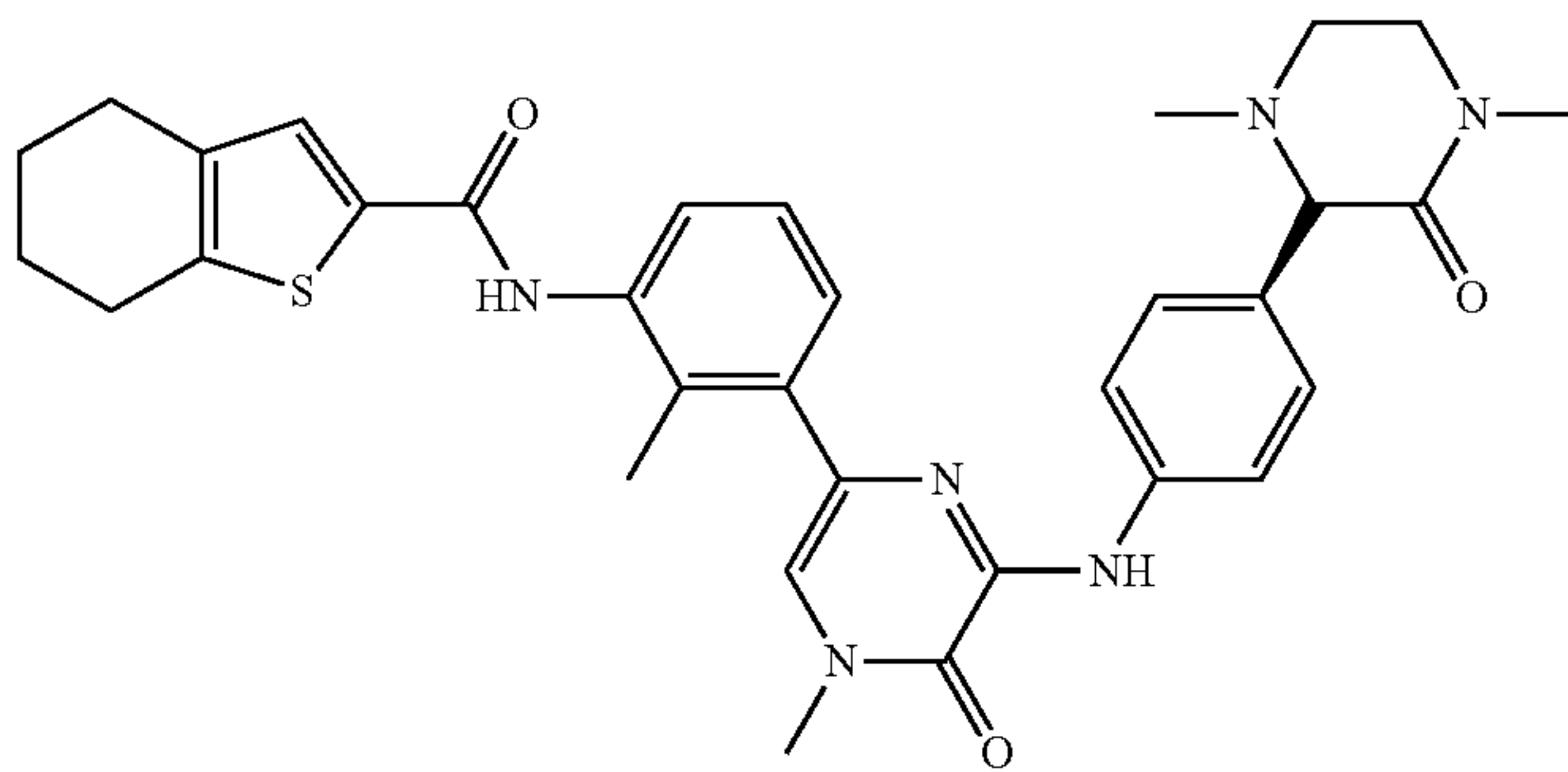
GDC-0834
