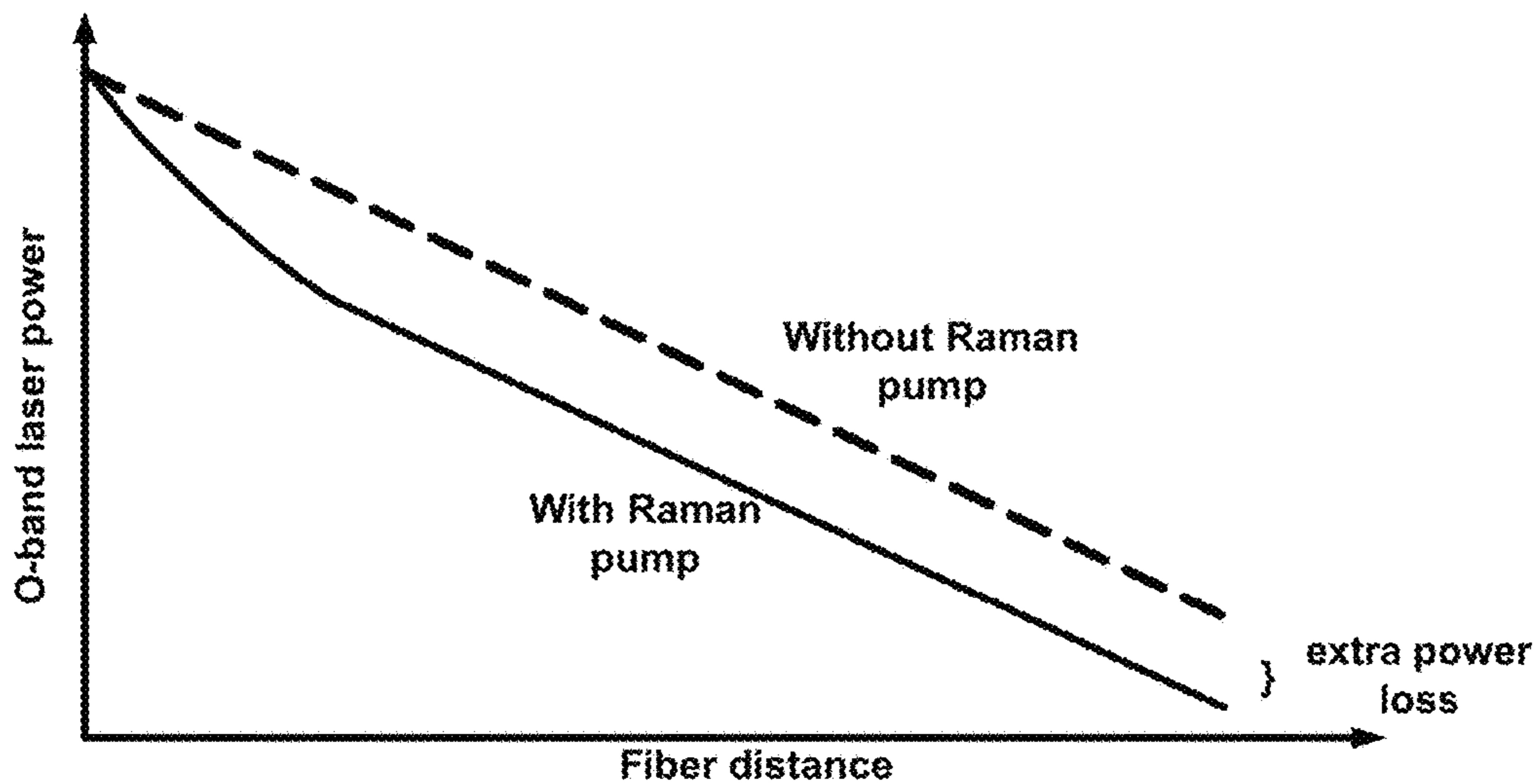
FIG. 8B
