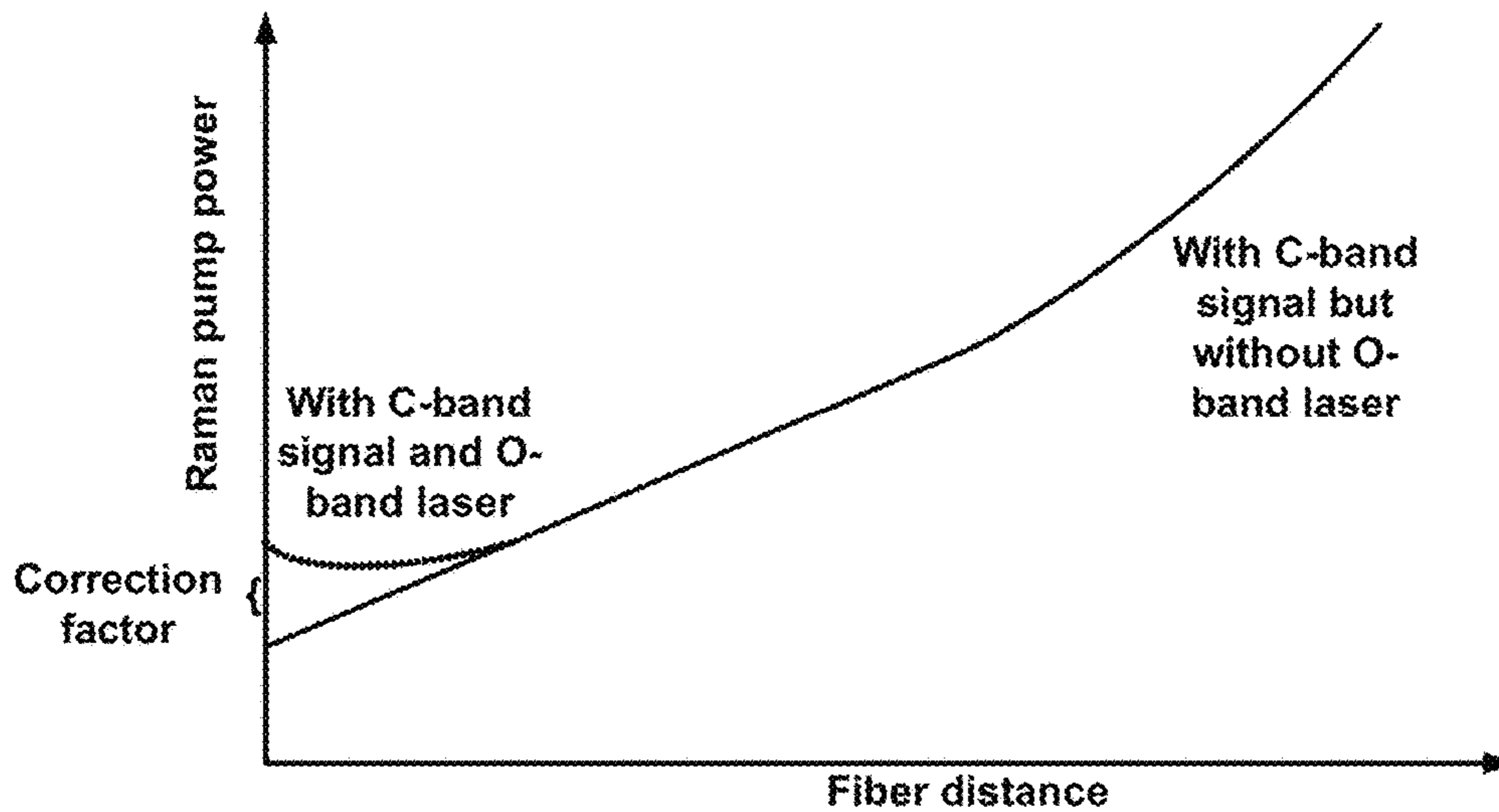
FIG. 8A
