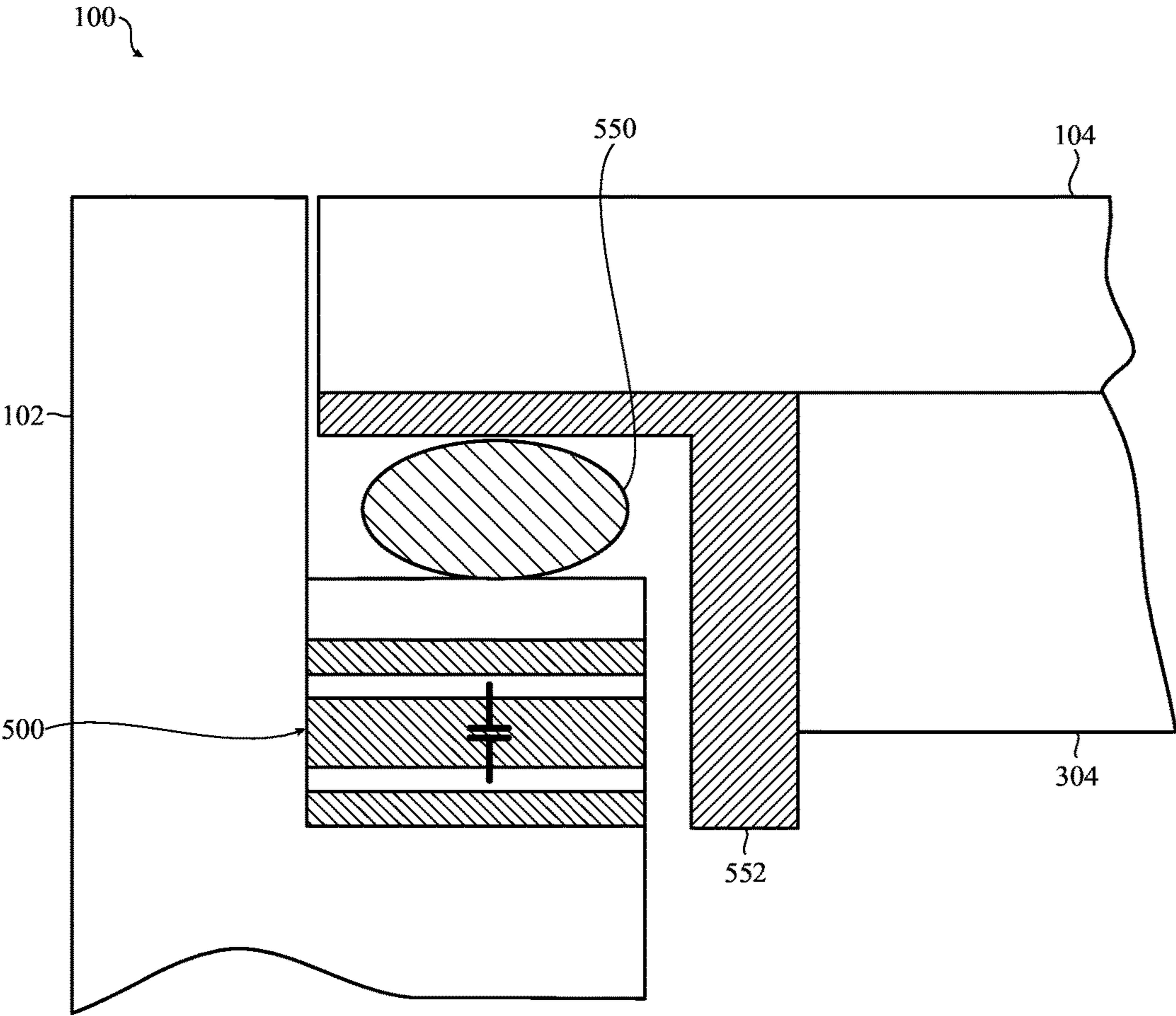
SECTION 2-2 FIG. 5
