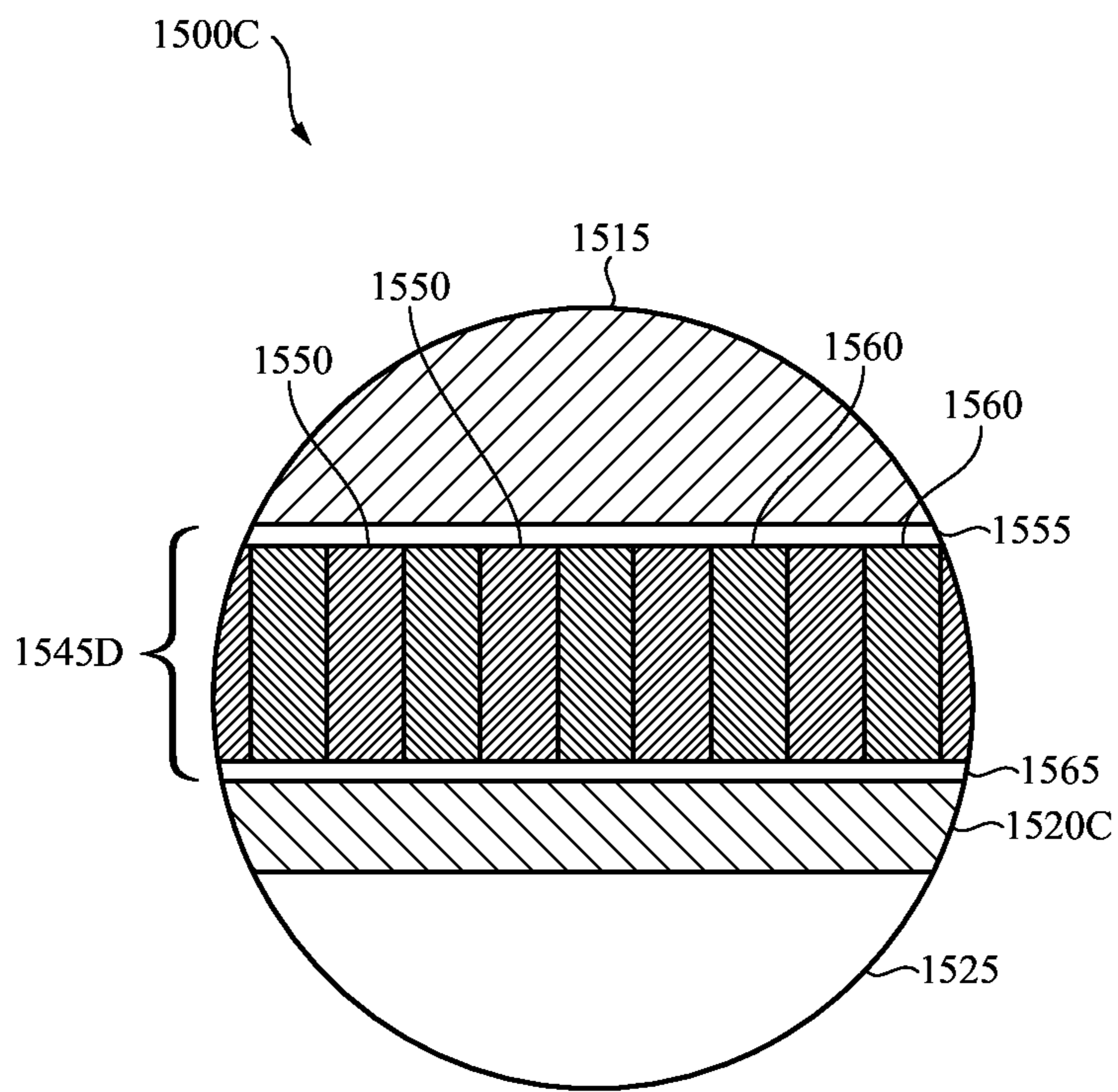
FIG. 15D
