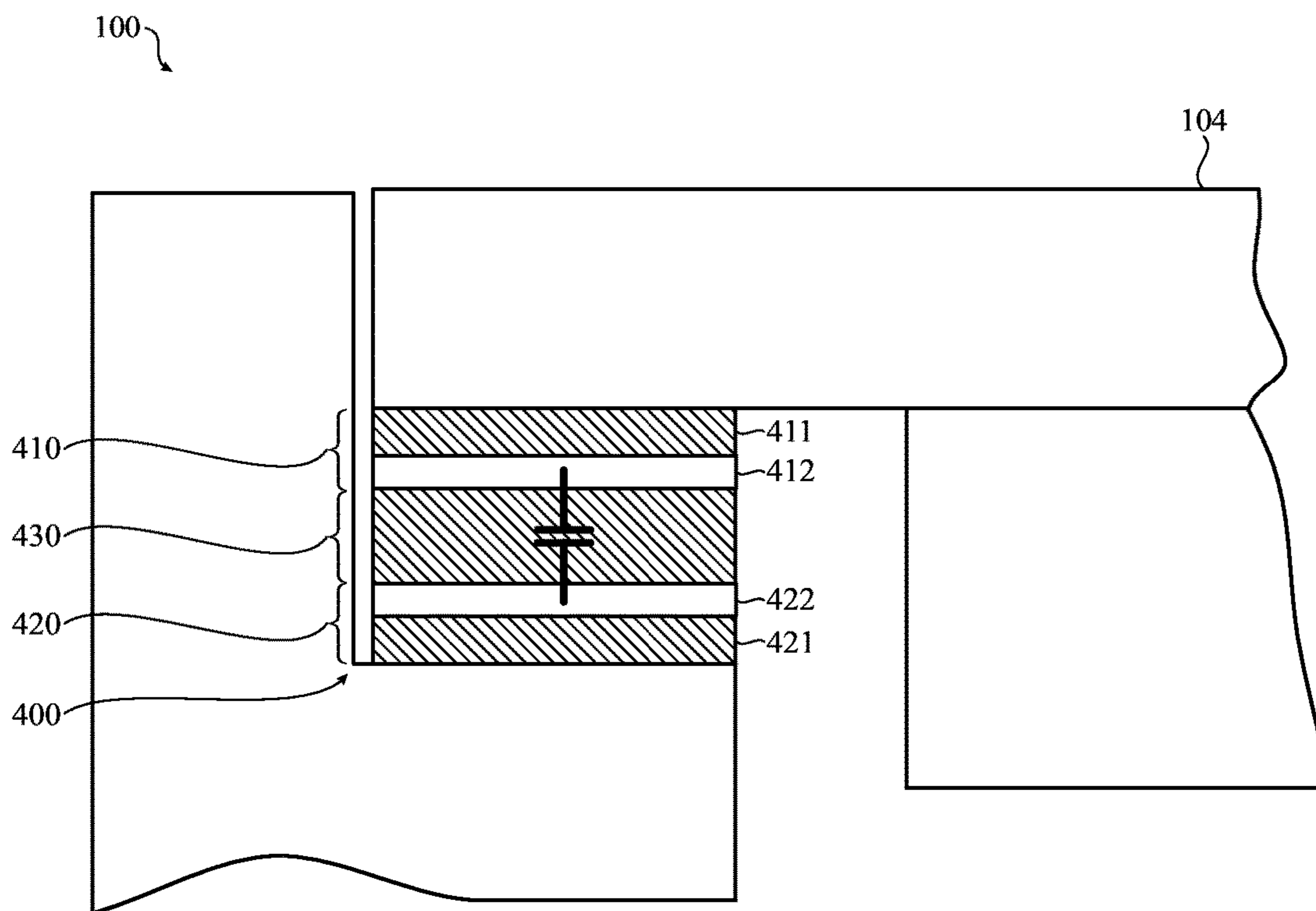
SECTION 2-2 FIG. 4
