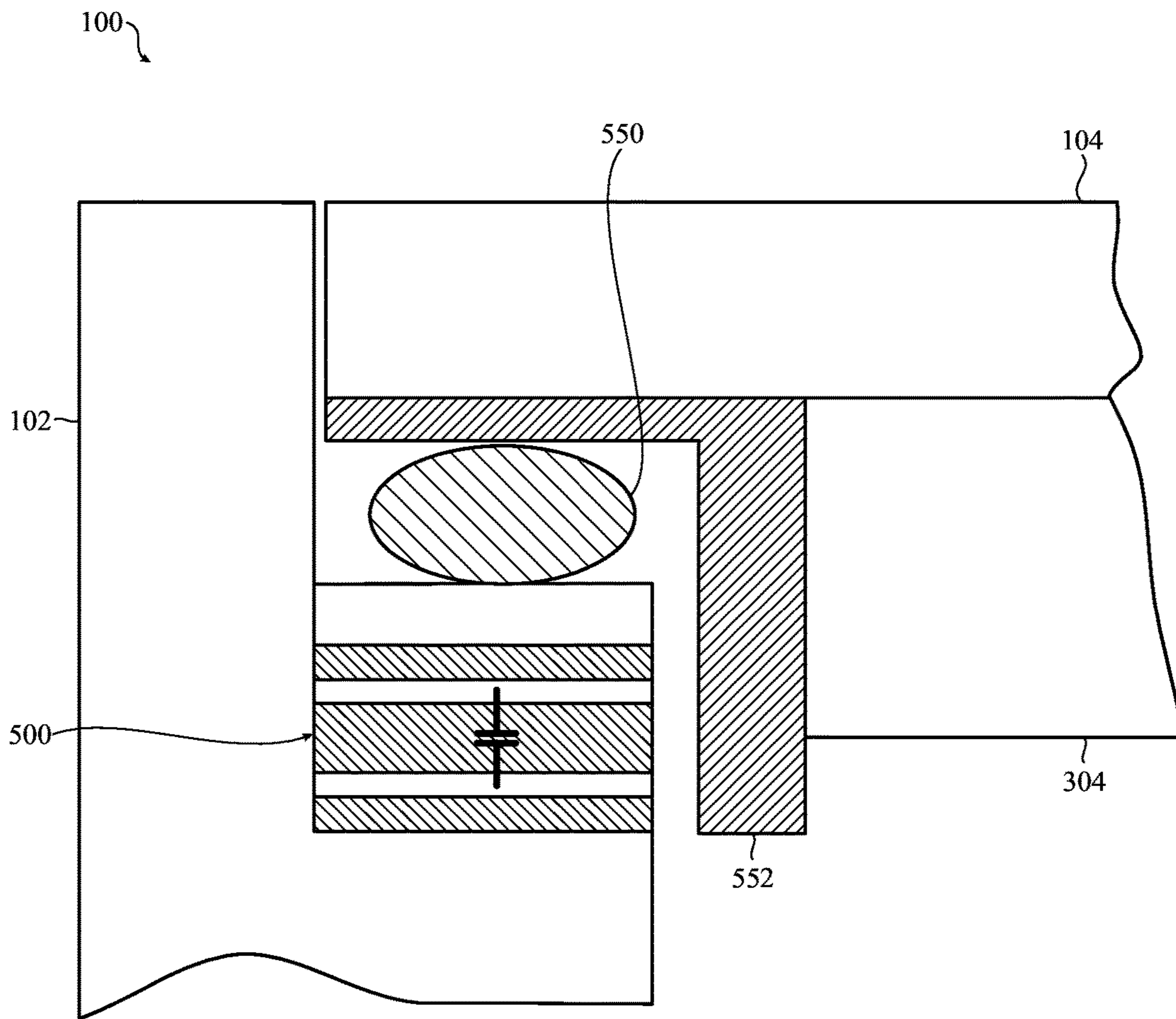
SECTION 2-2 FIG. 5
