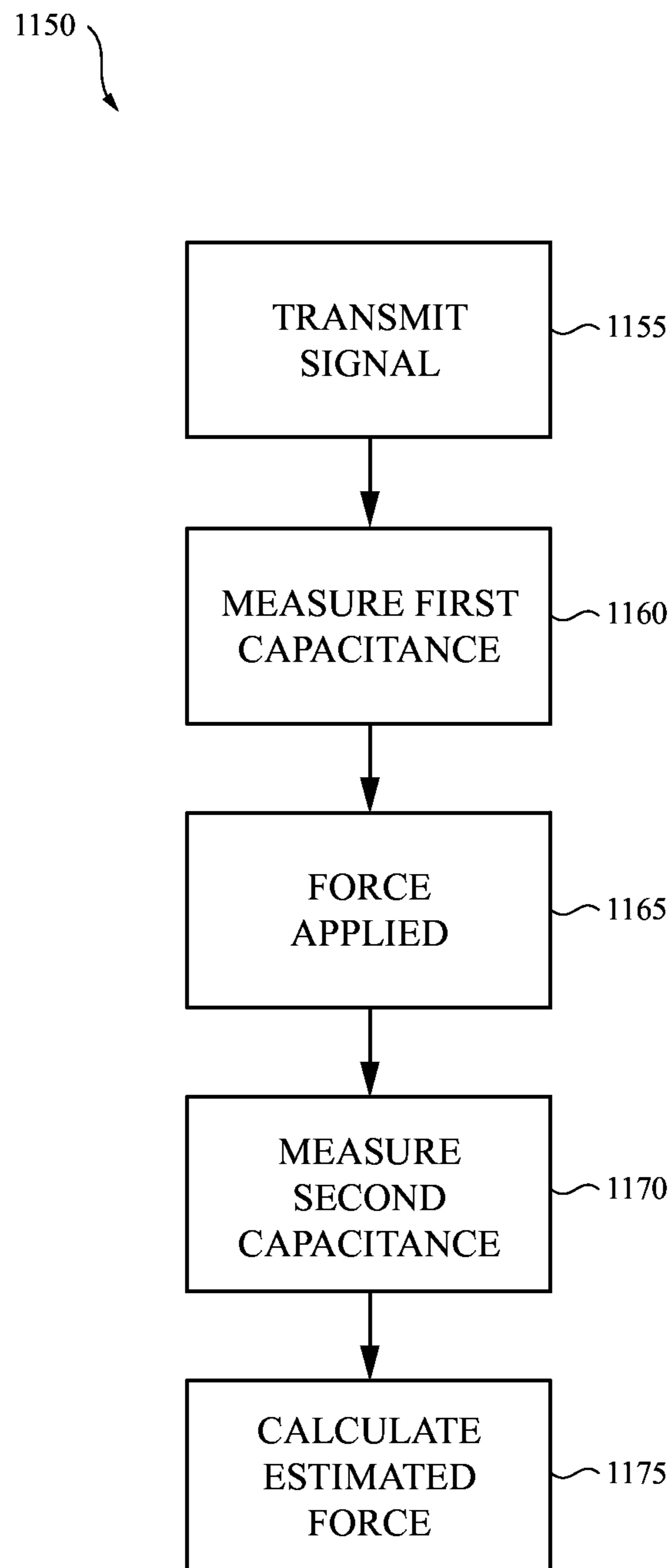
FIG. 11B
