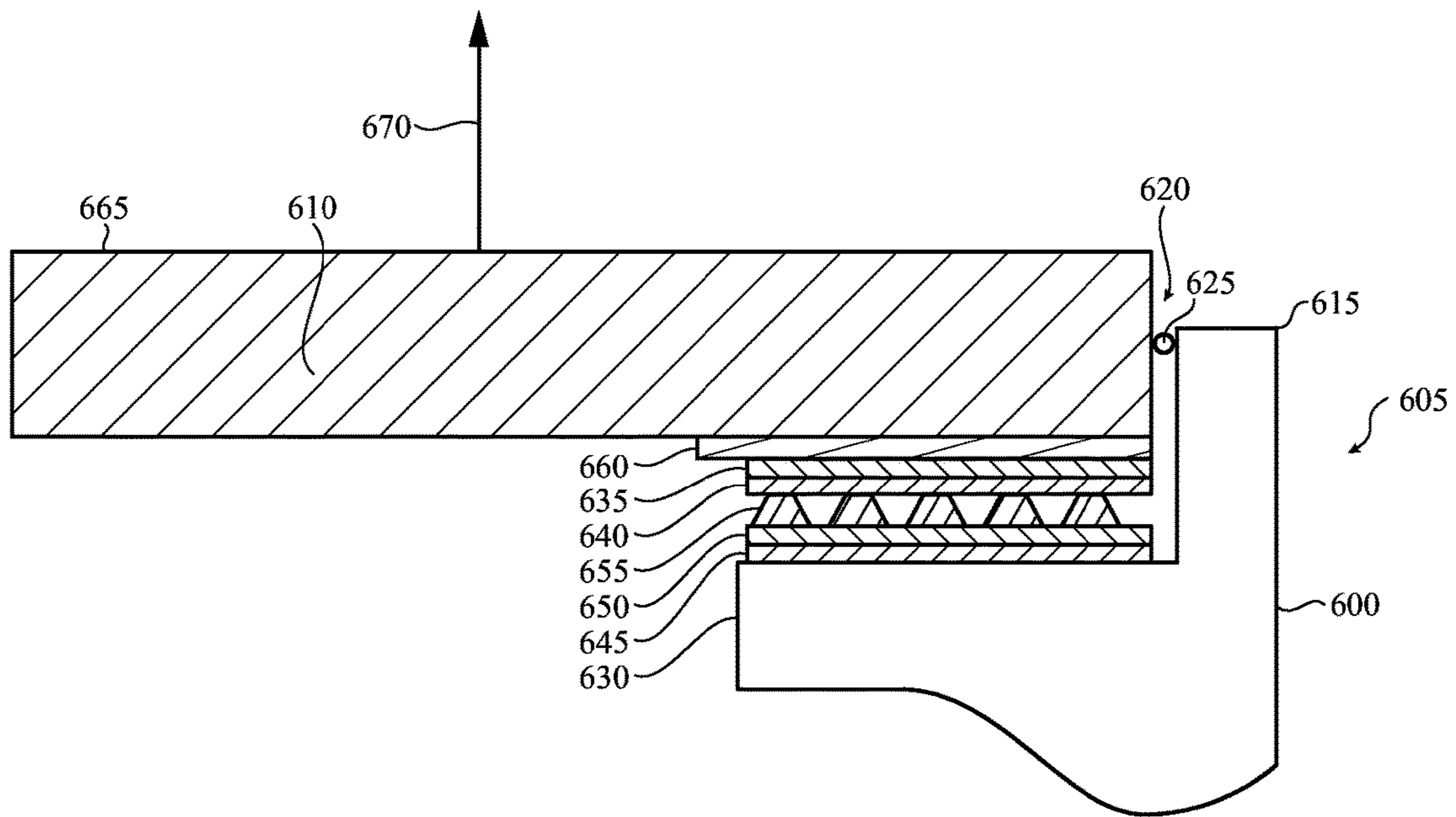
FIG. 6
