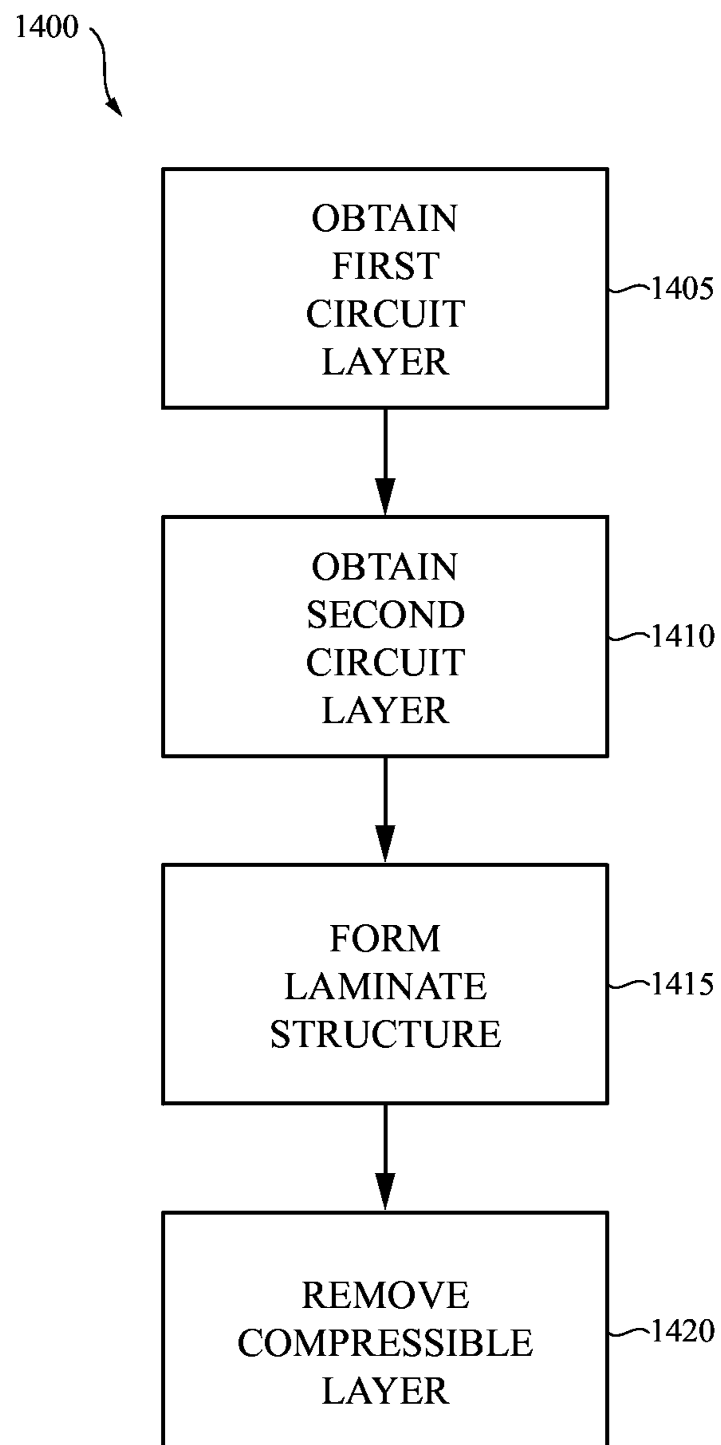
FIG. 14
