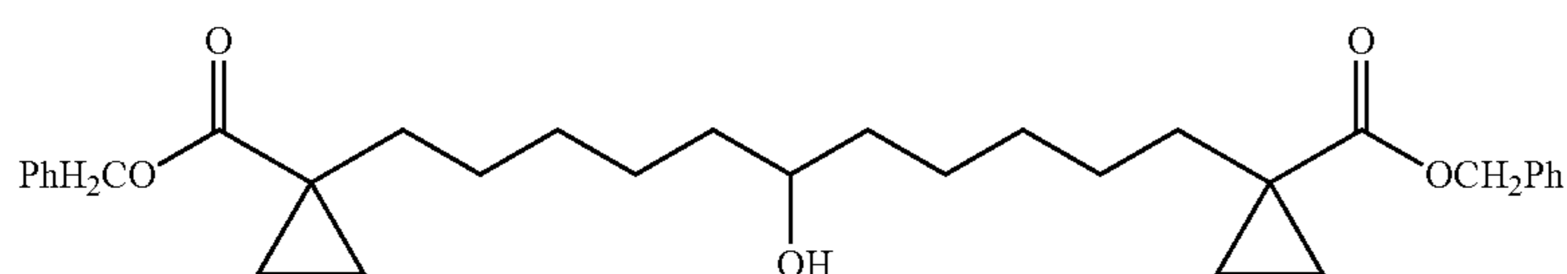
1,11-Bis-(1-benzyloxycarbonyl-cyclopropyl)-undecan-6-ol
