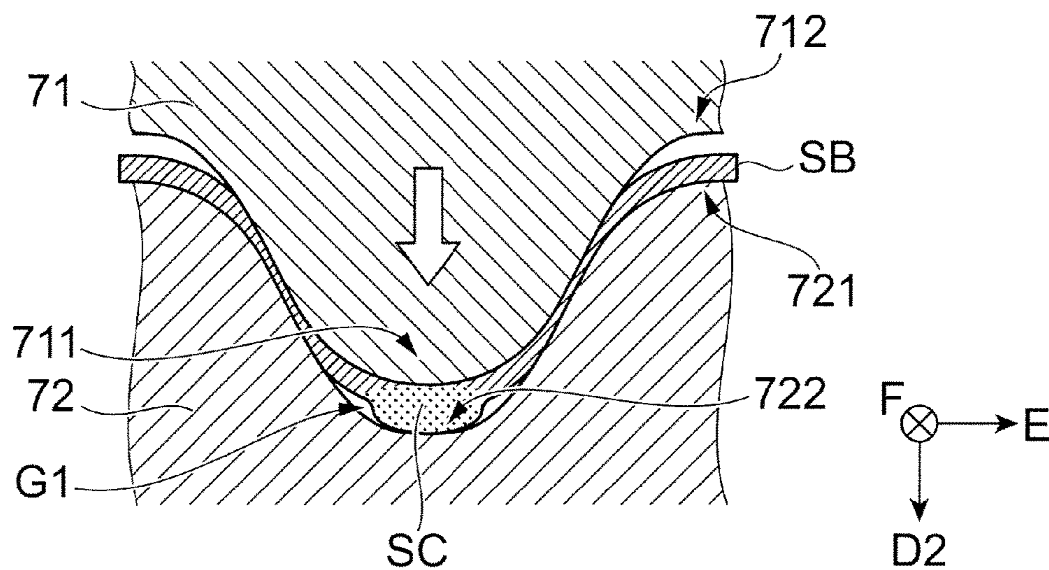
FIG. 5D
