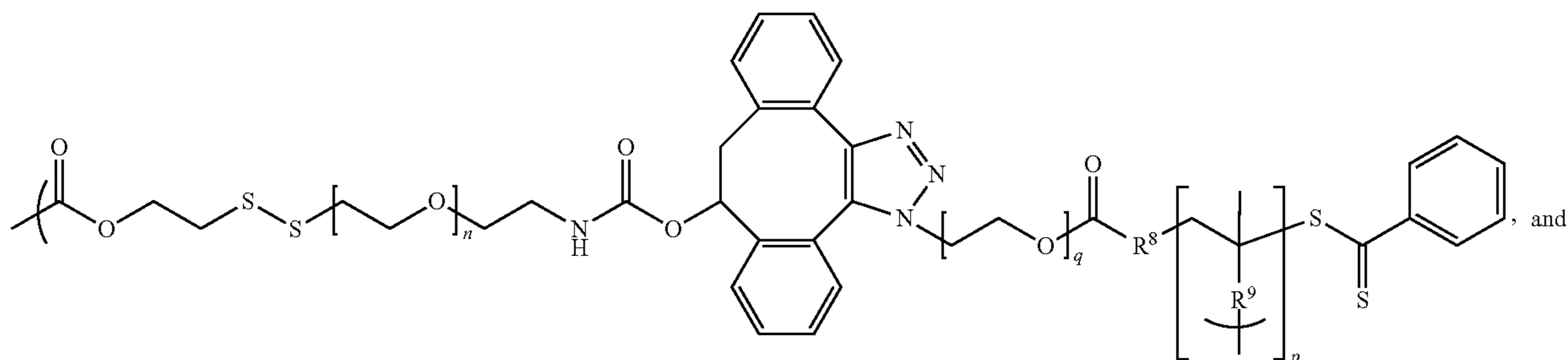
Formula Yn
