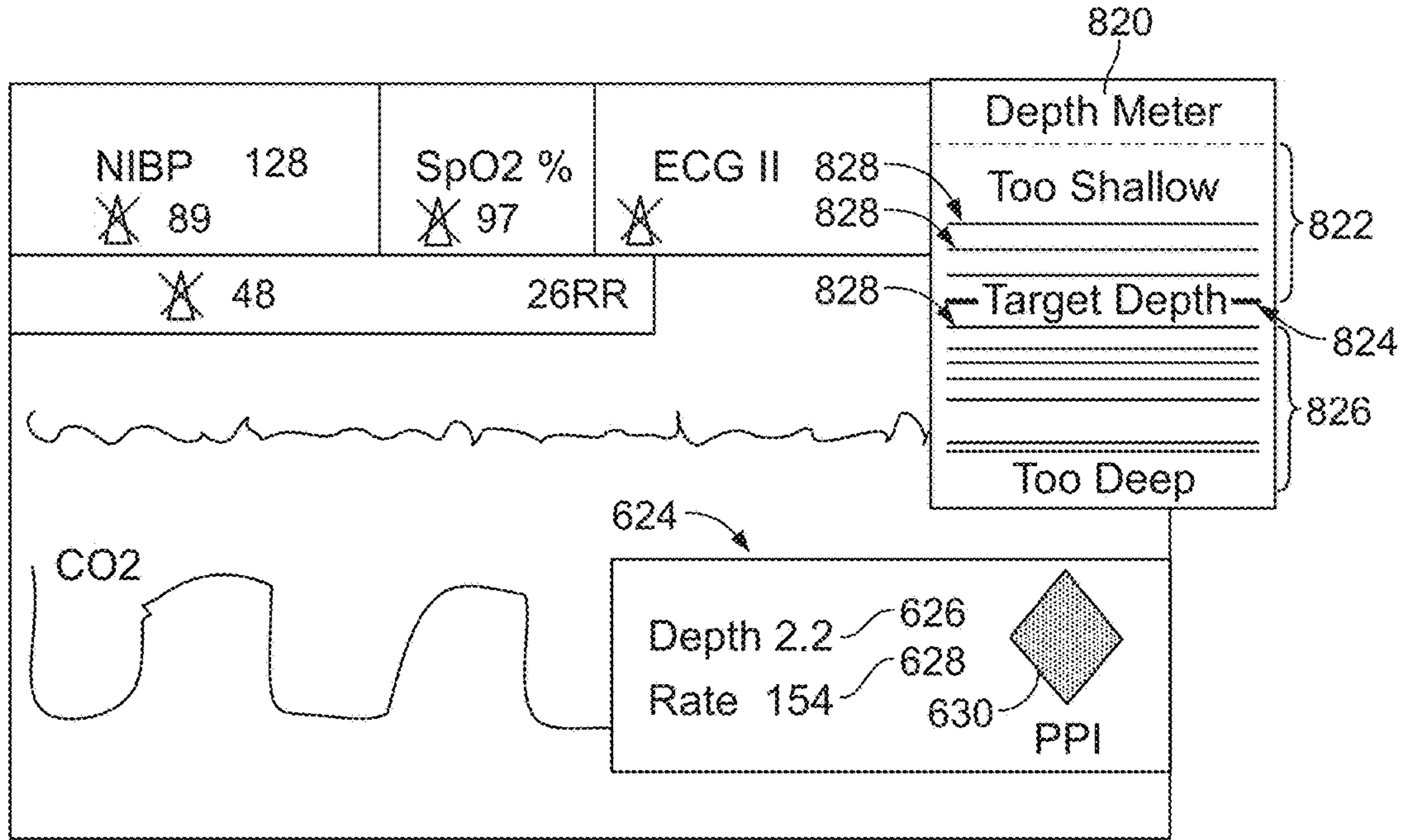
FIG. 8A
