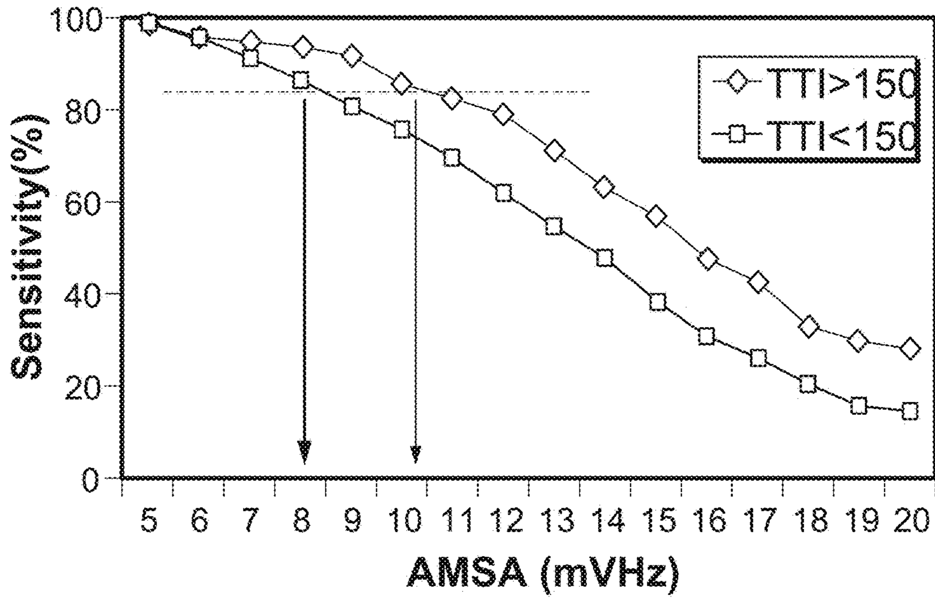
FIG. 4A
