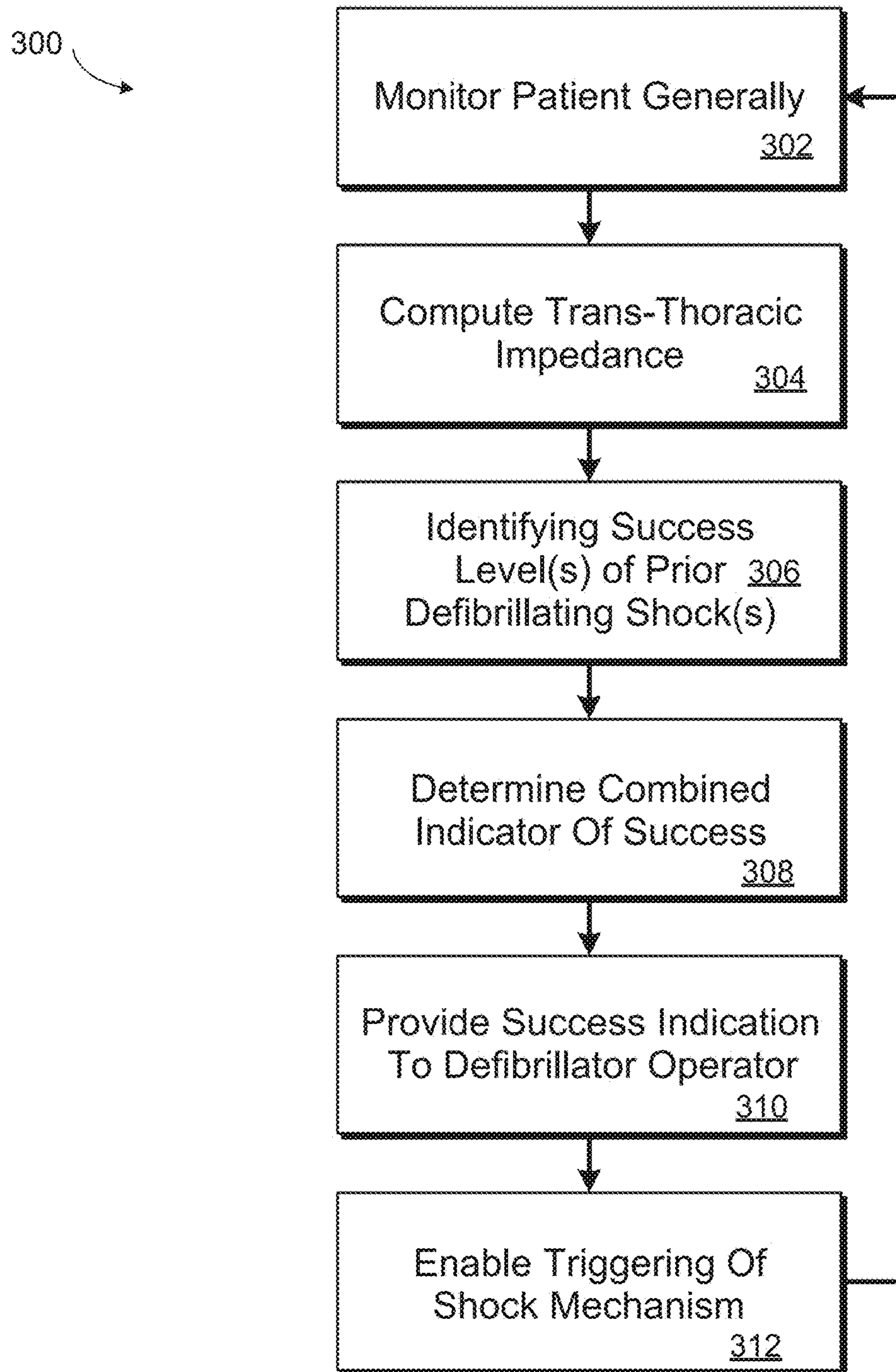
FIG. 3A
