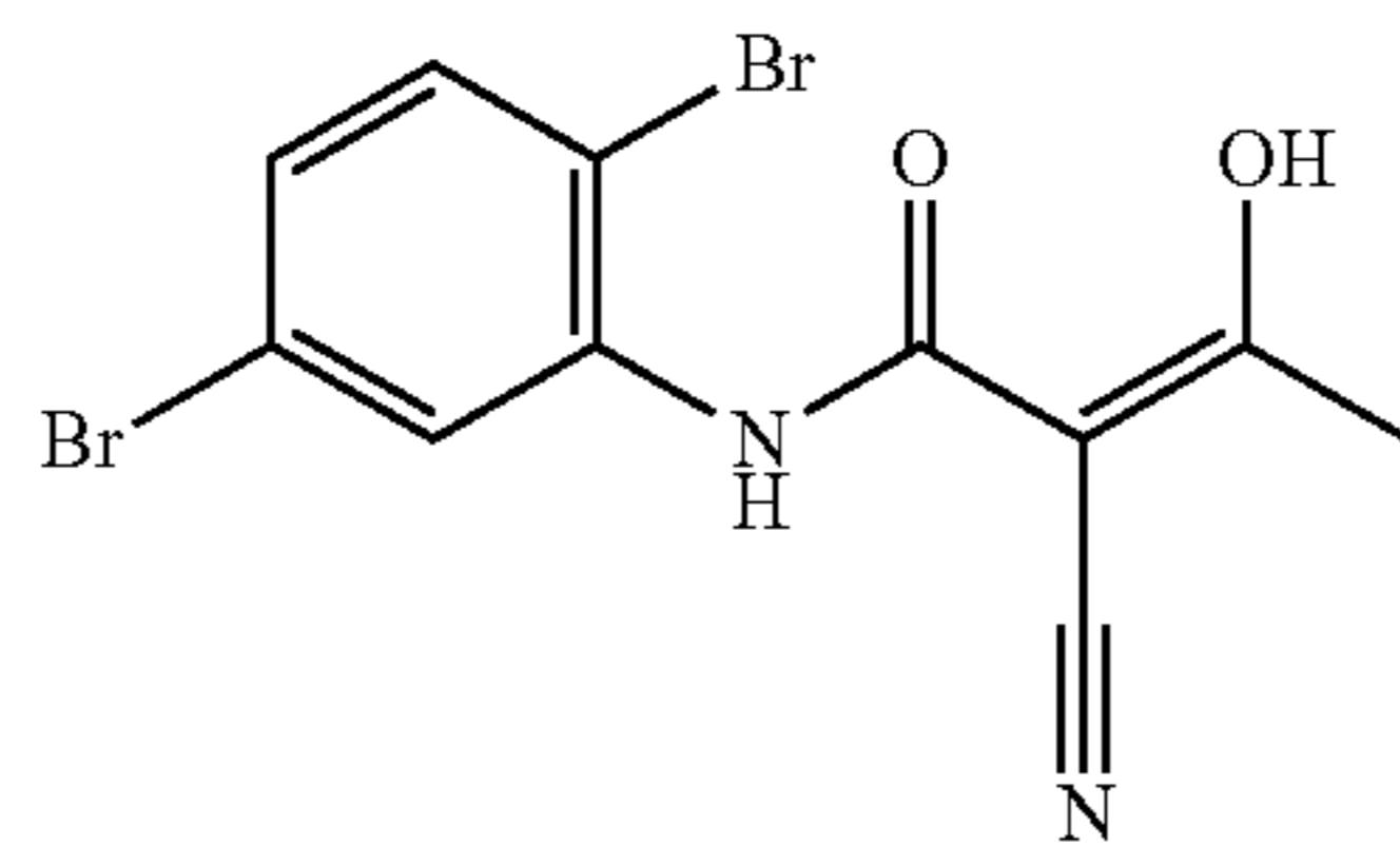
LFM-A13
