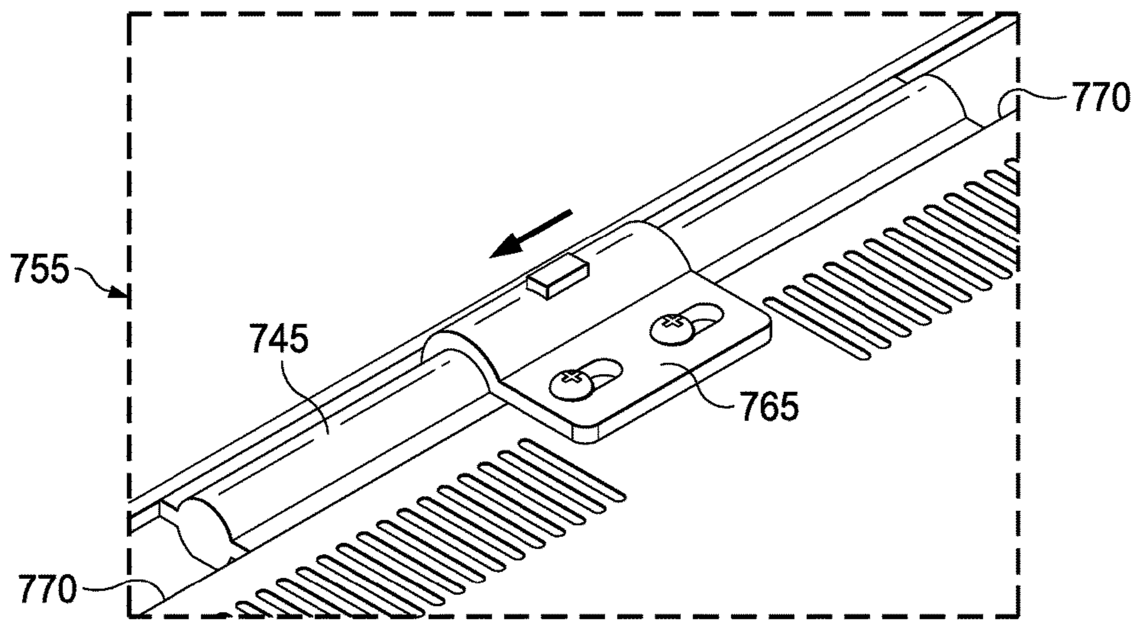
FIG. 7e
