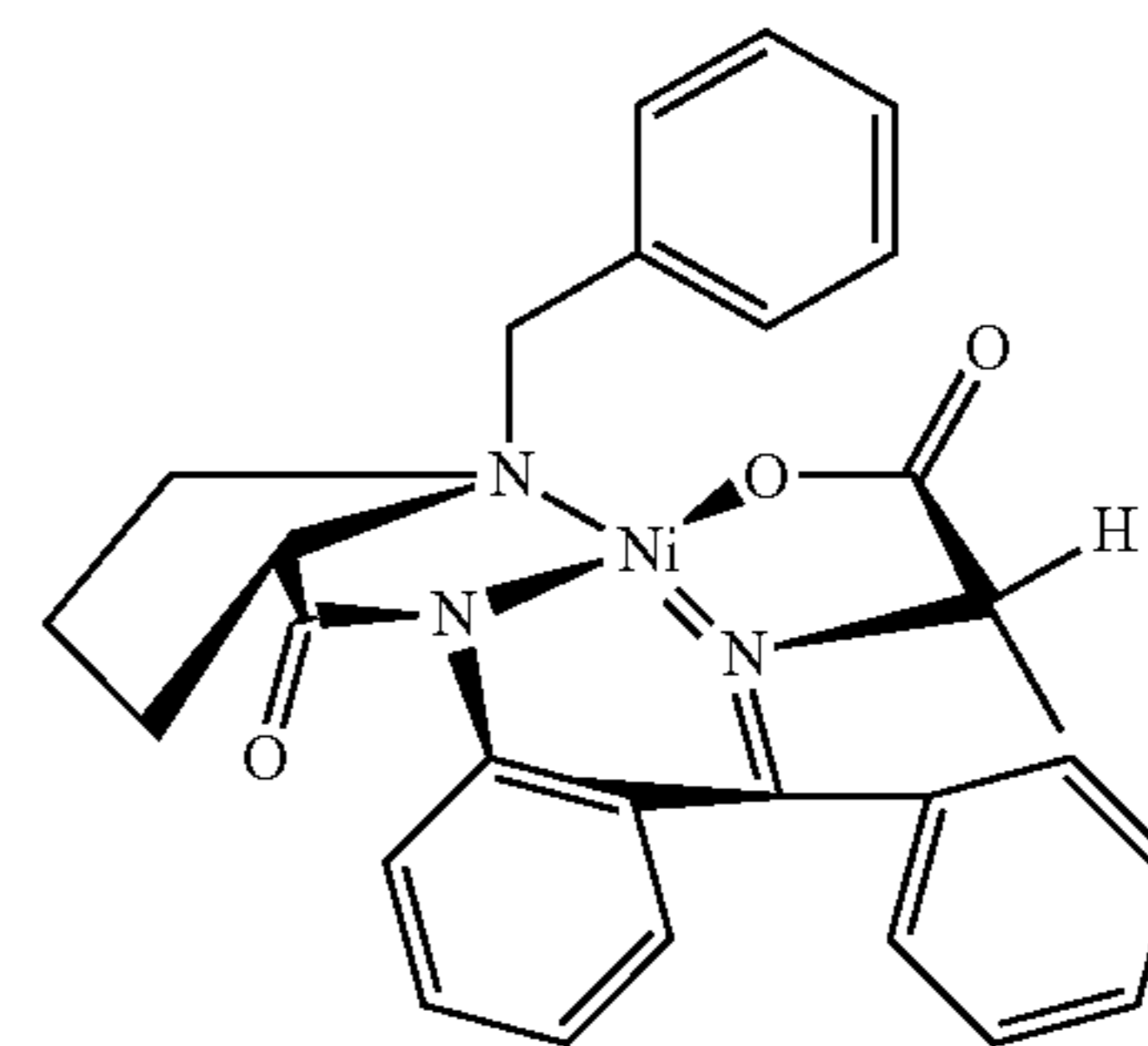
S-Ala-Ni-BPB
