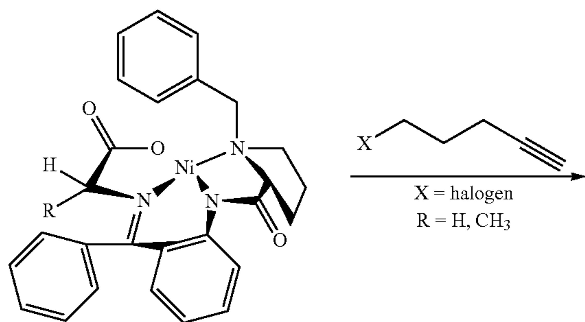
R-AA-Ni-BPB
