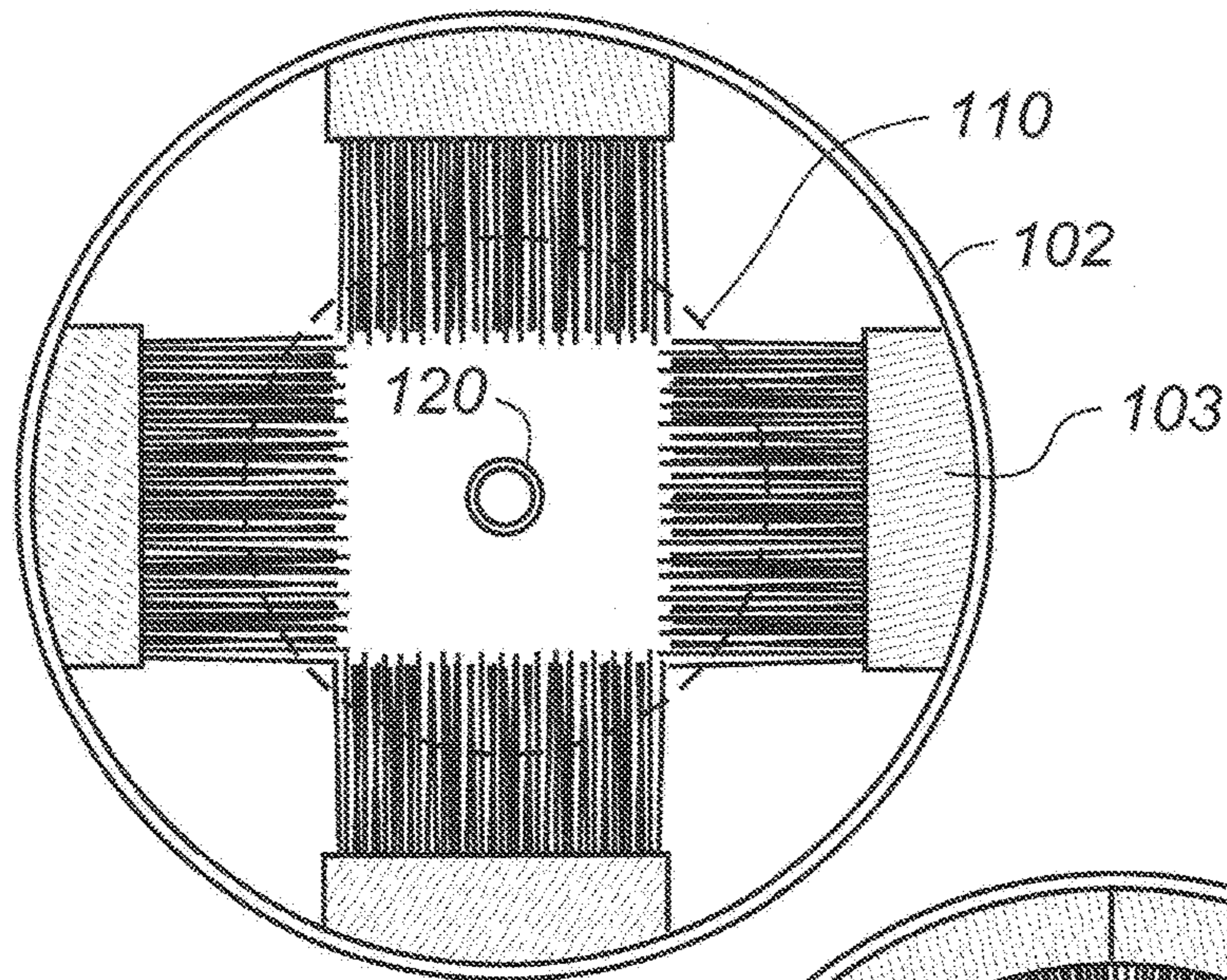
Fig. 2 (Sec. A-A)
