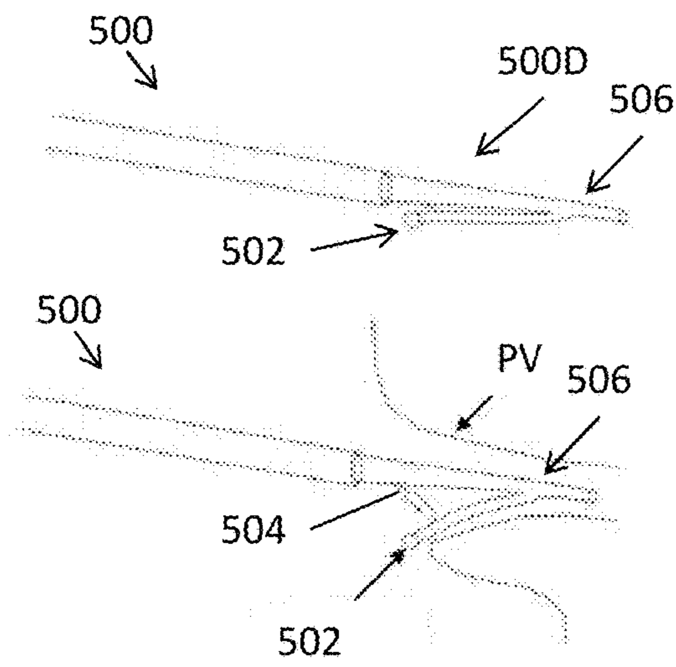
FIG. 5A
