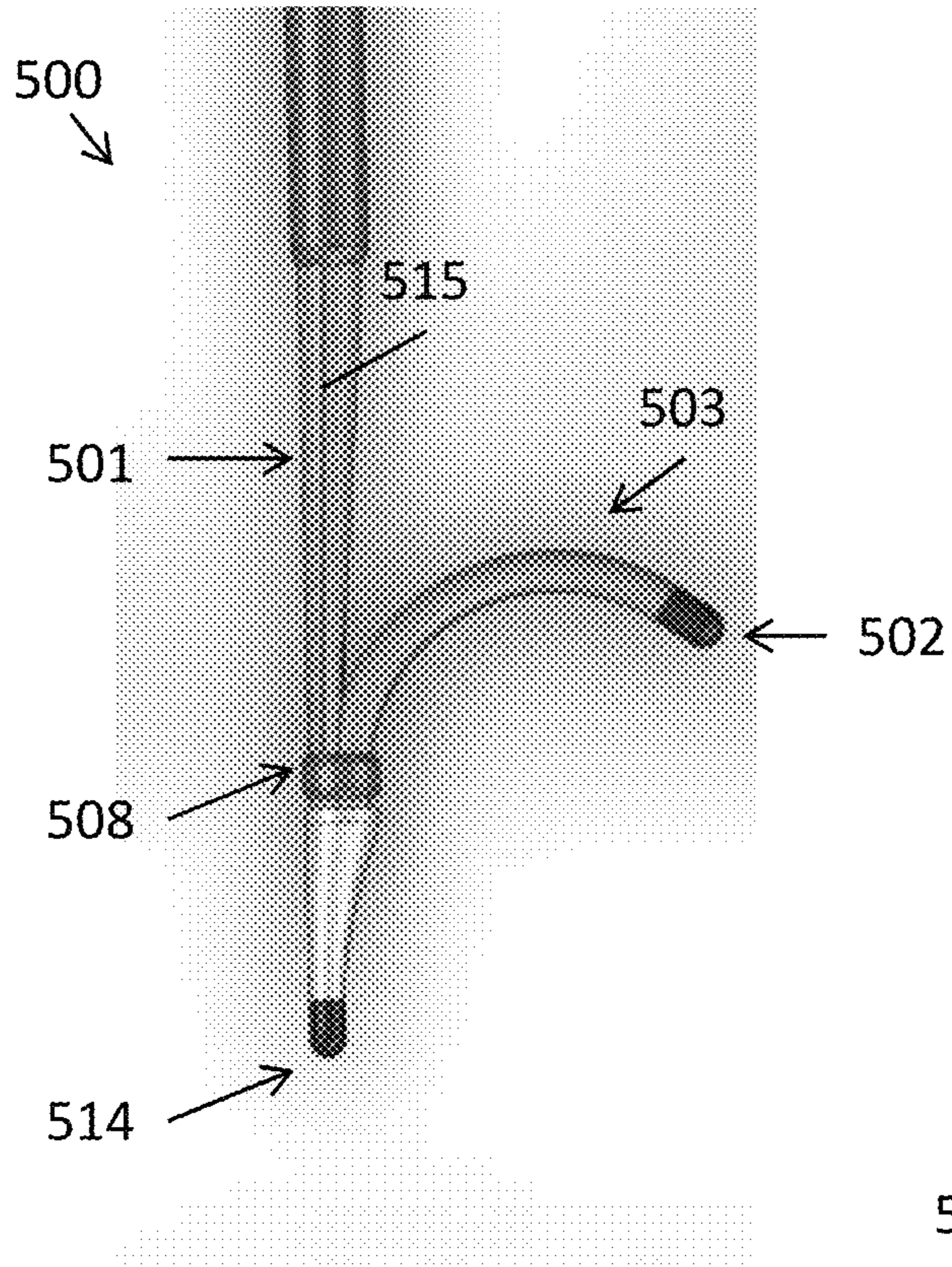
FIG. 16D
