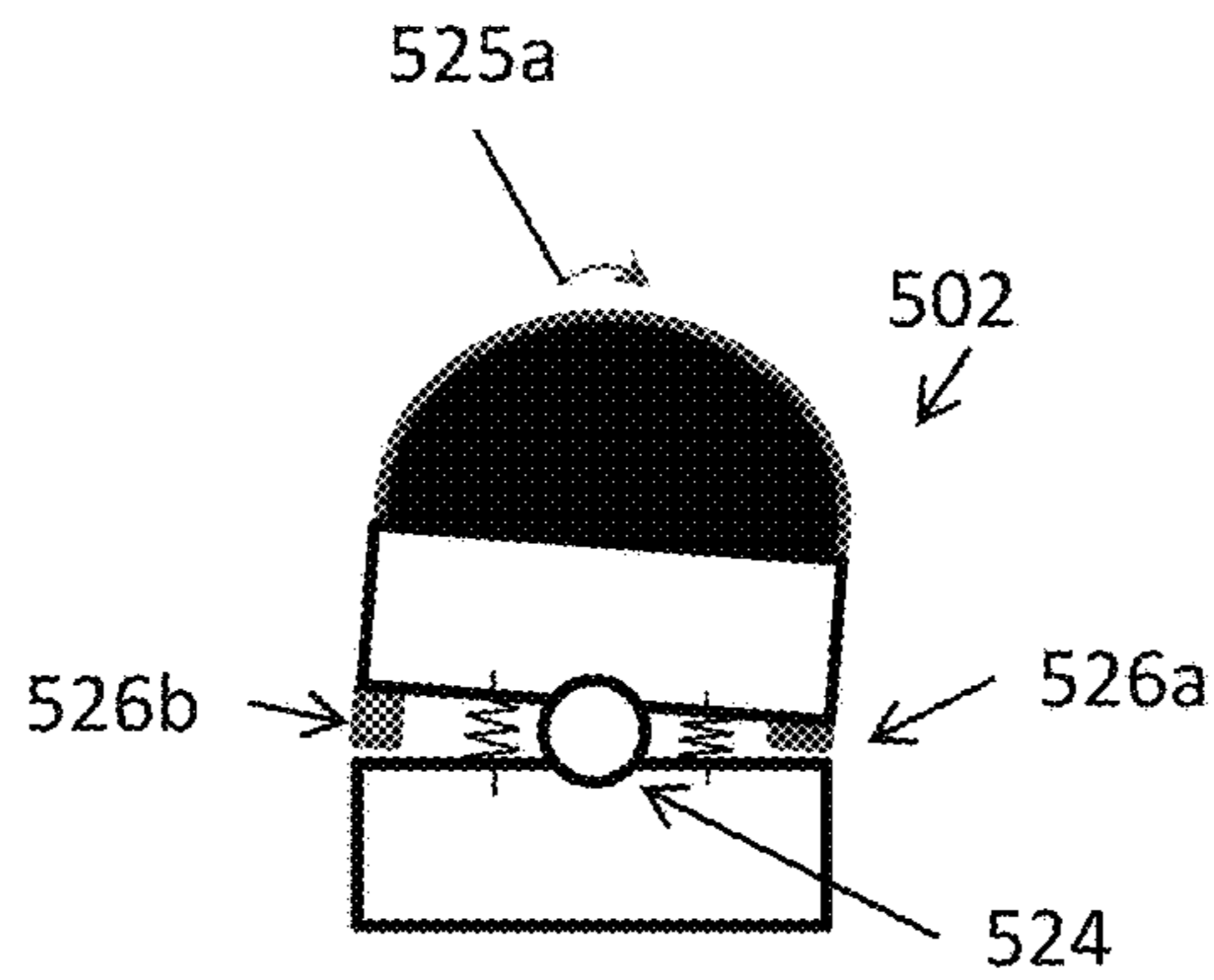
FIG. 20B
