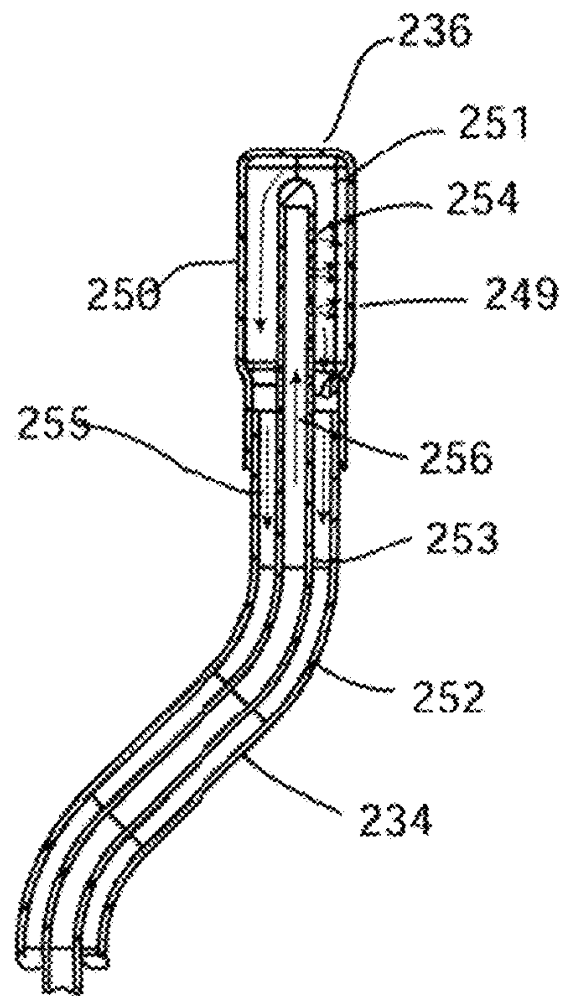
Section A-A
