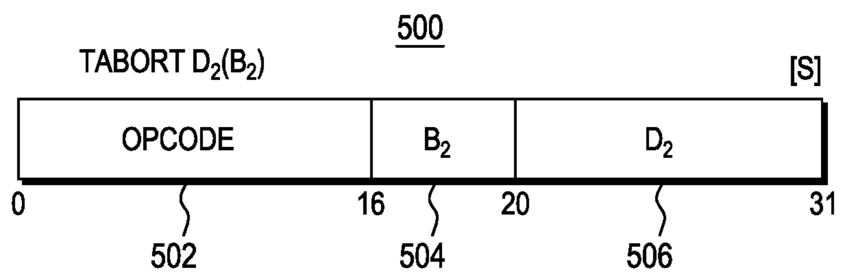
FIG. 5
