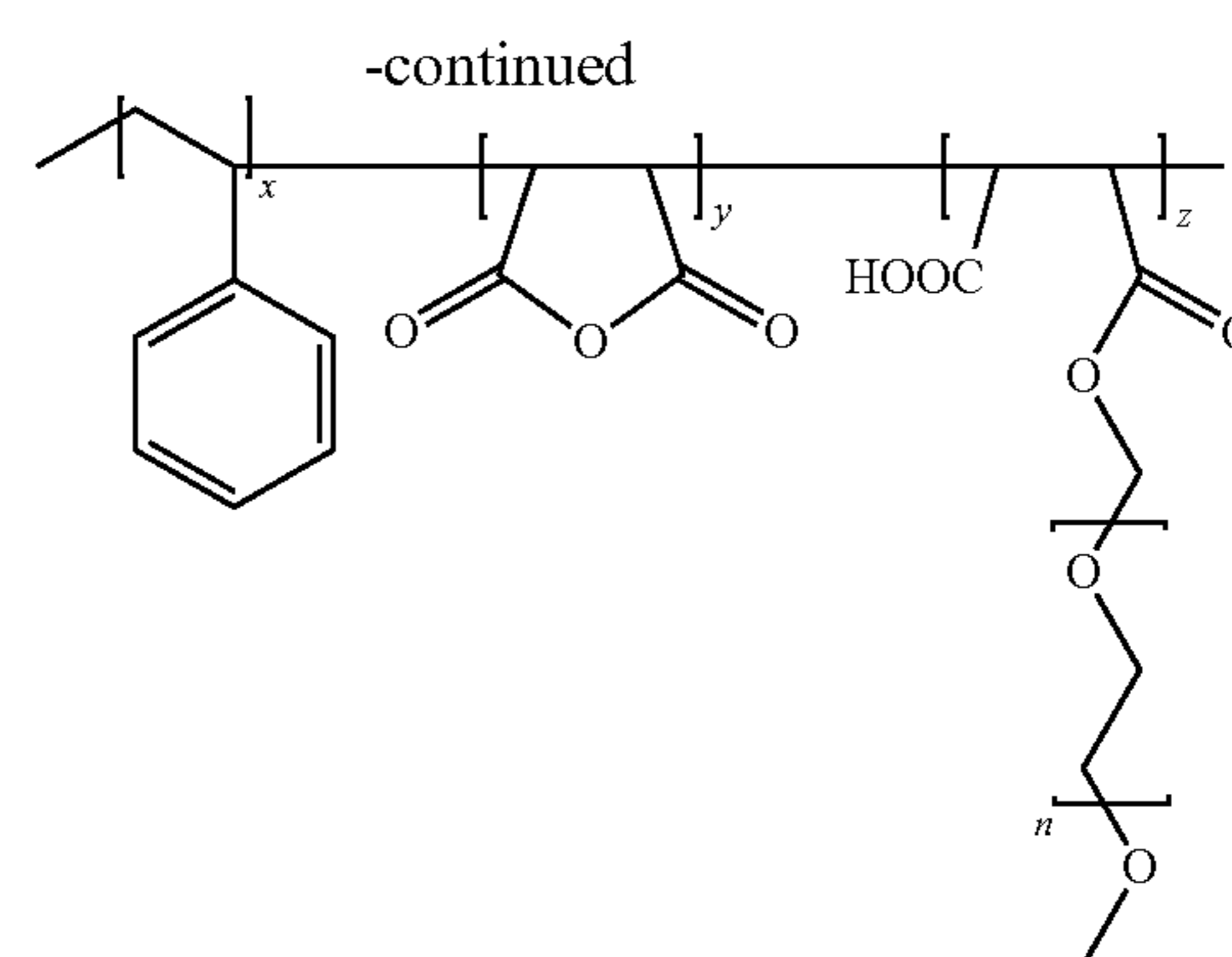
P(S-alt-MA)-g-PEO
