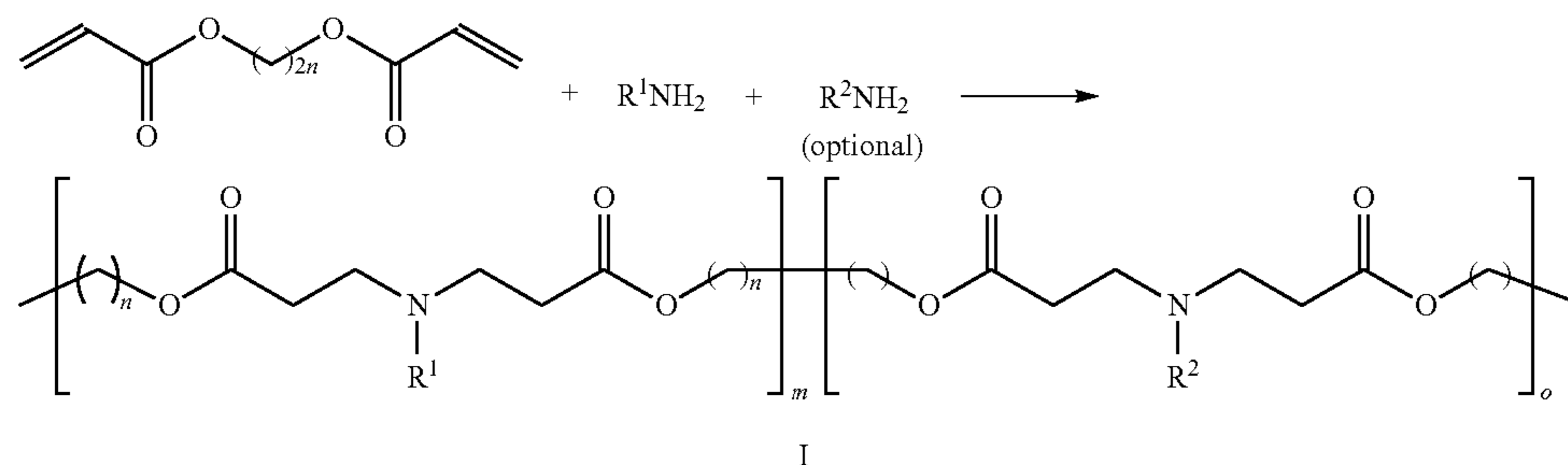
A. Scheme I.
