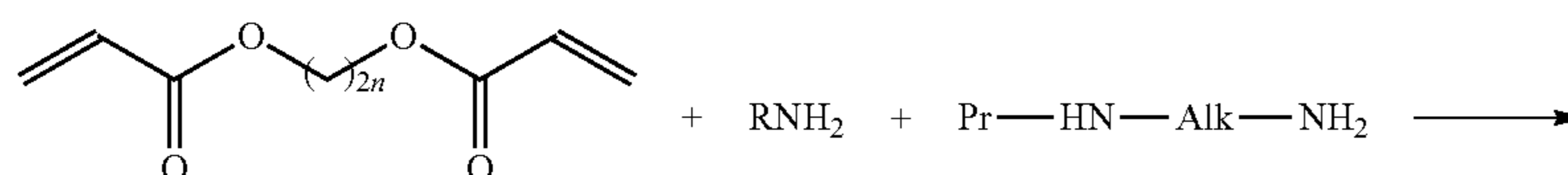
B. Scheme II.
