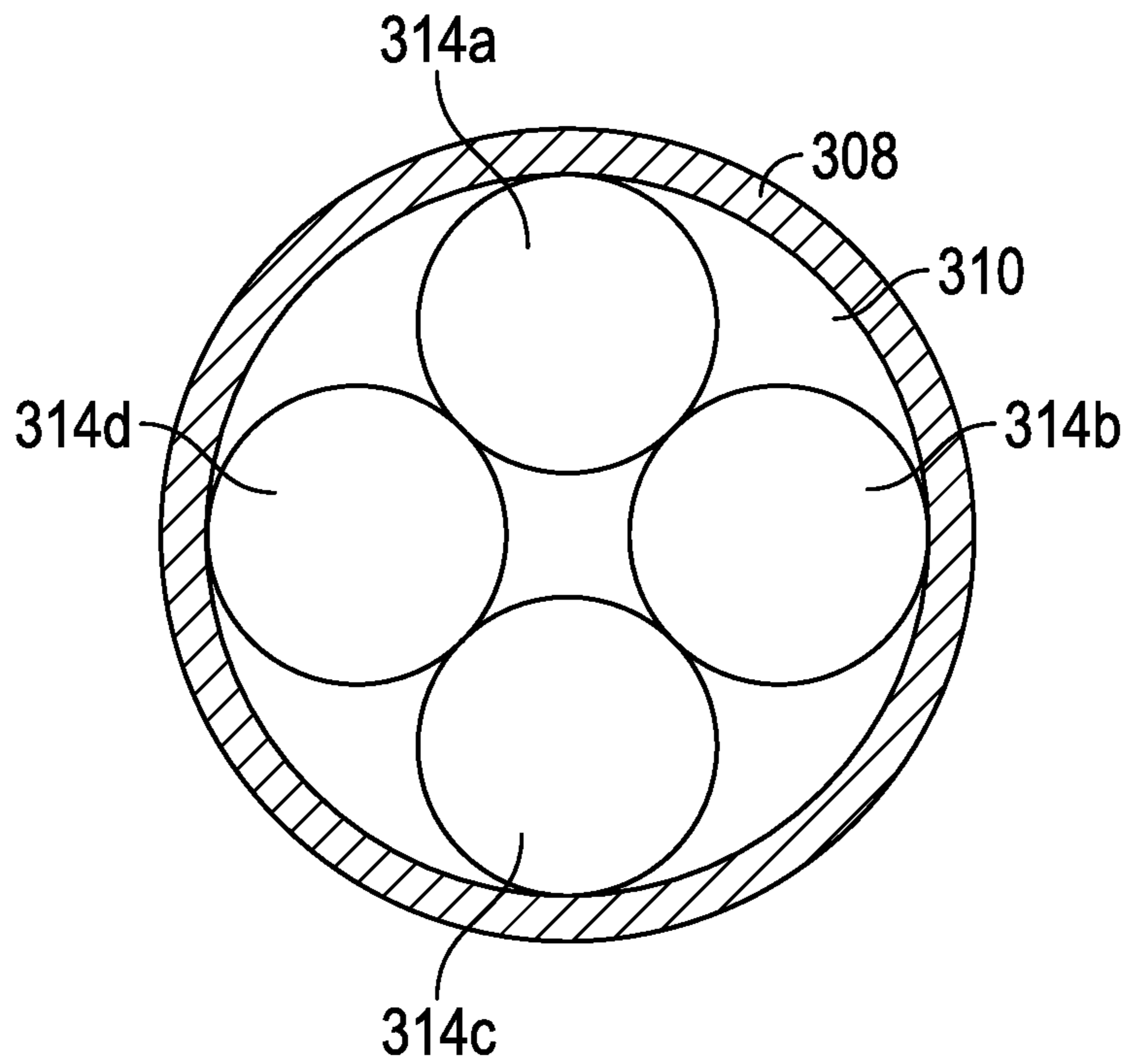
FIG. 14C
