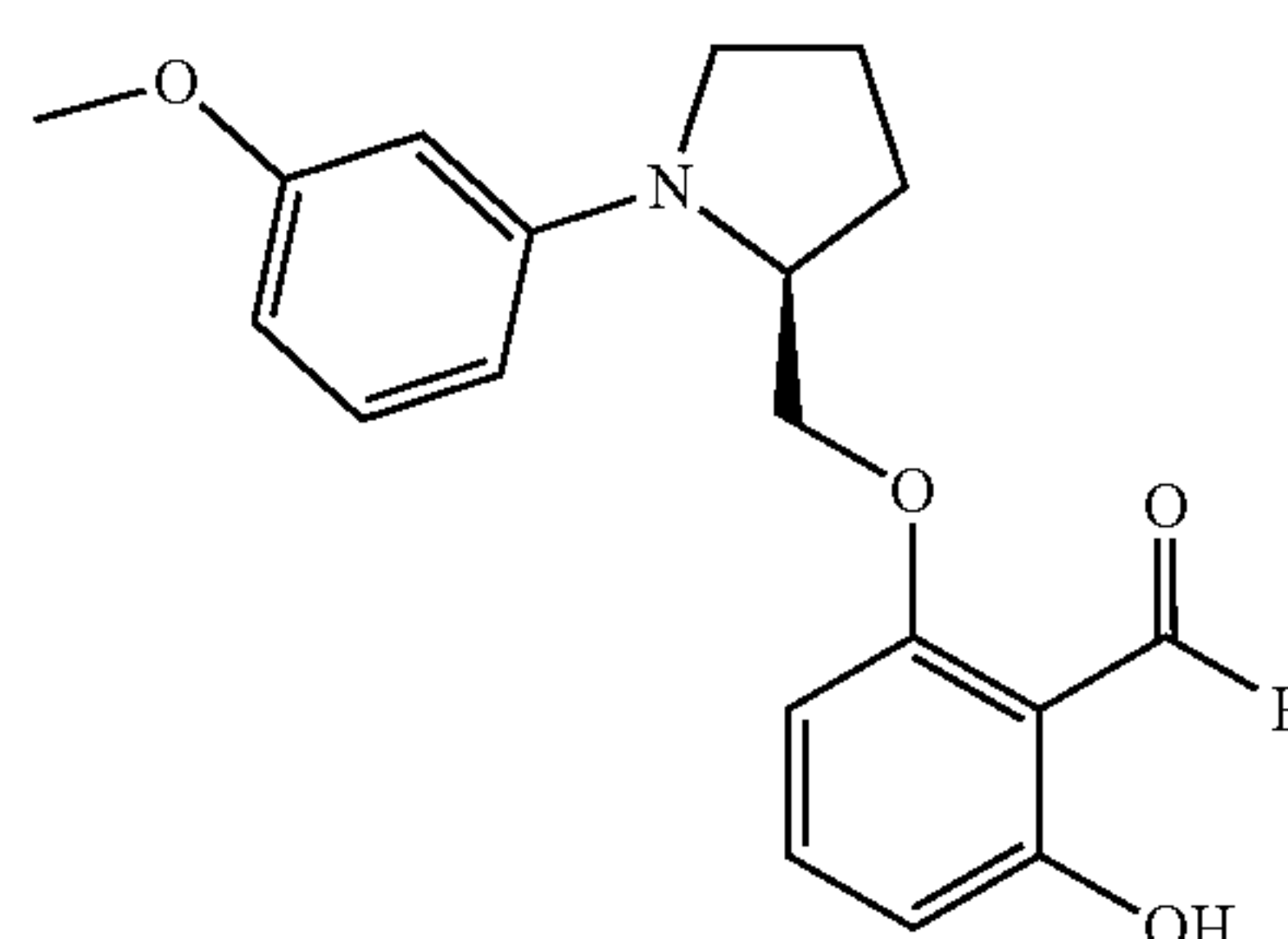
(S)-2-hydroxy-6-((1-(3-methoxyphenyl)pyrrolidin-2-yl)methoxy)benzaldehyde
