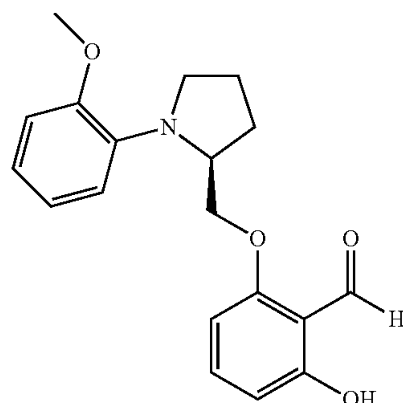
(S)-2-hydroxy-6-((1-(2-methoxyphenyl)pyrrolidin-2-yl)methoxy)benzaldehyde
