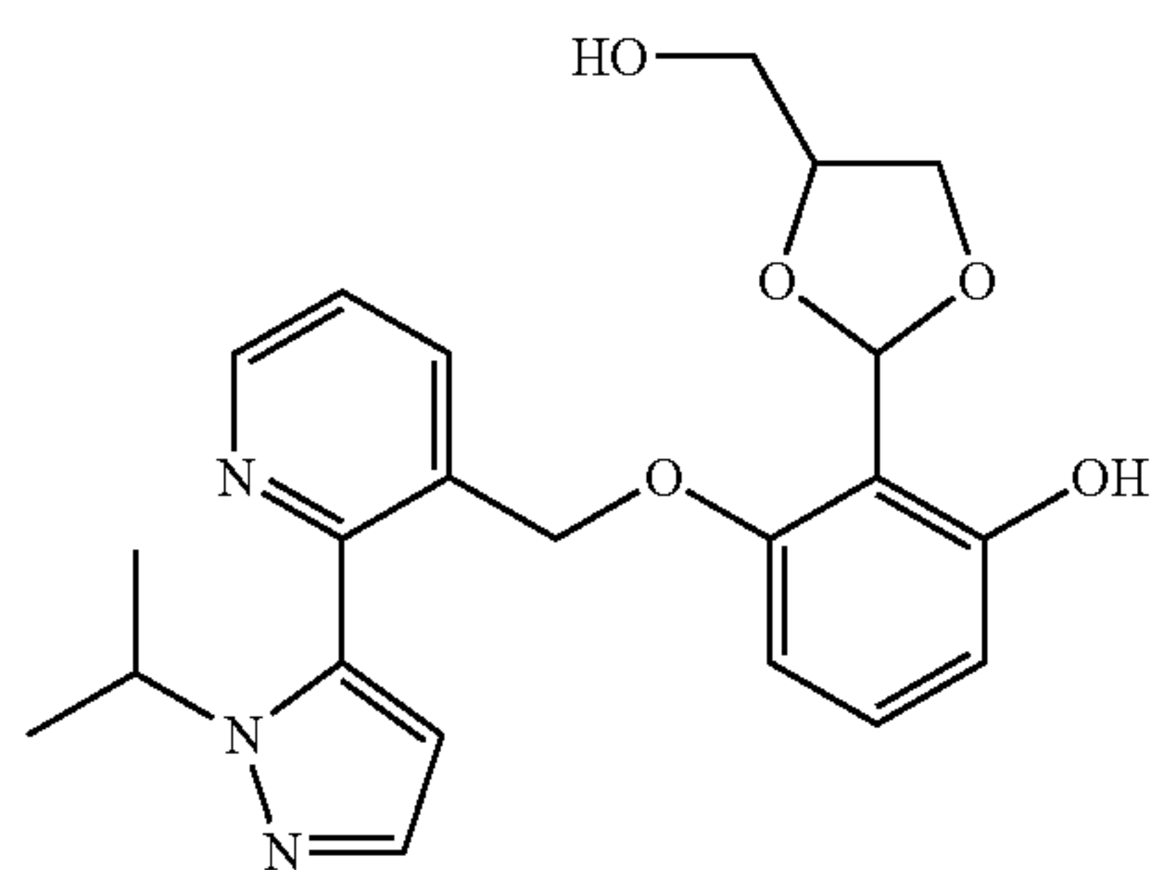
GBT1007—2-(4-(hydroxymethyl)-1,3-dioxolan-2-yl)-3-((2-(1-isopropyl-1H-pyrazol-5-yl)pyridin-3-yl)methoxy)phenol
