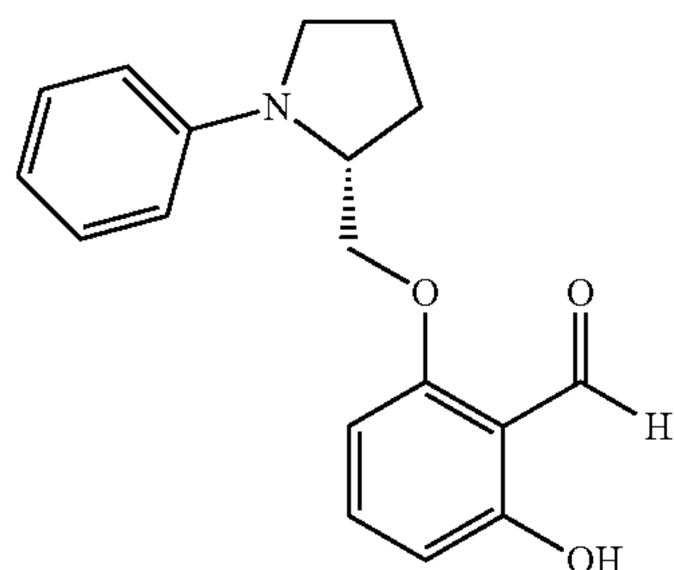
(R)-2-hydroxy-6-((1-phenylpyrrolidin-2-yl)methoxy)benzaldehyde
