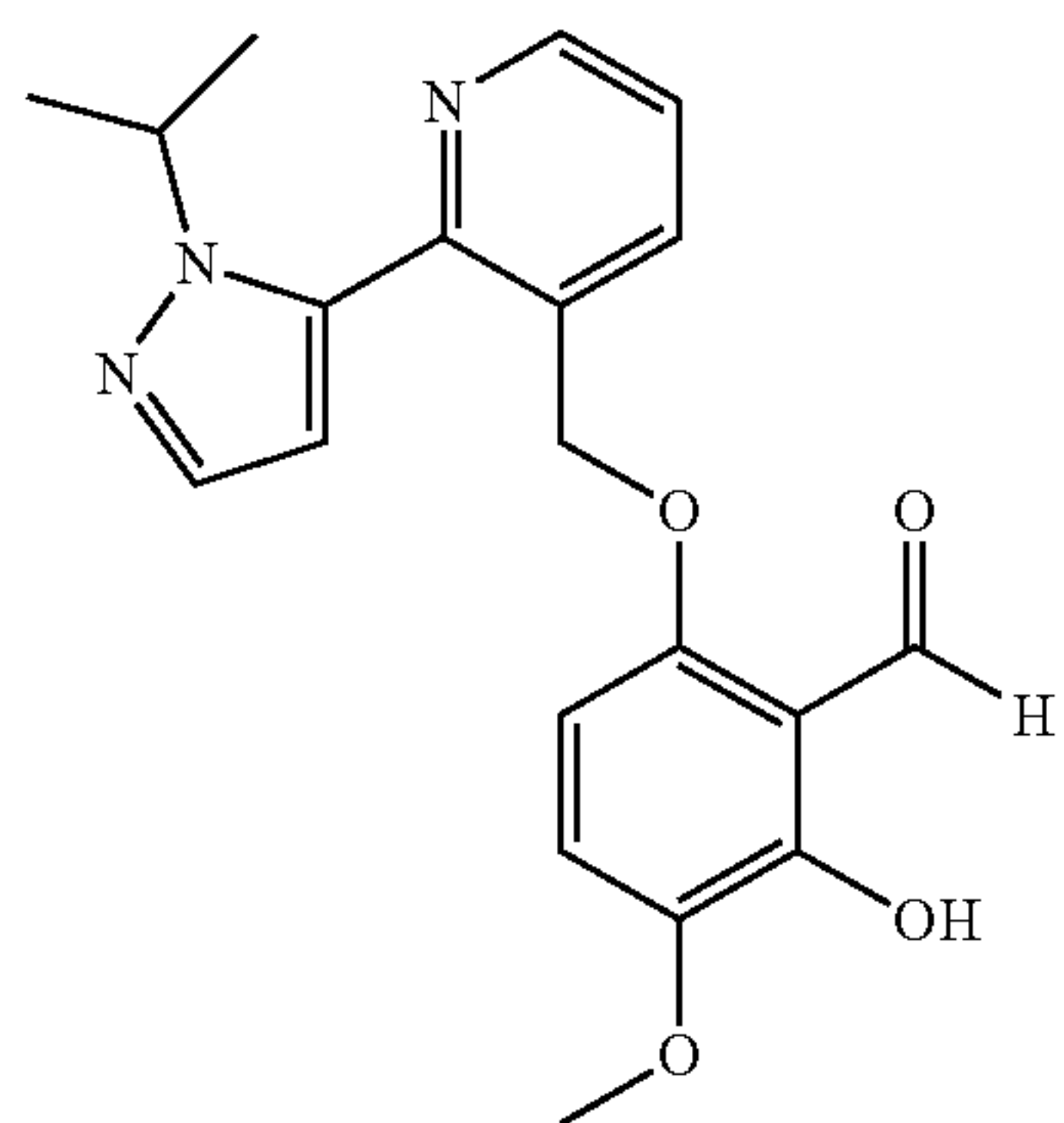
2-hydroxy-6-((2-(1-isopropyl-1H-pyrazol-5-yl)pyridin-3-yl)methoxy)-3-methoxybenzaldehyde
