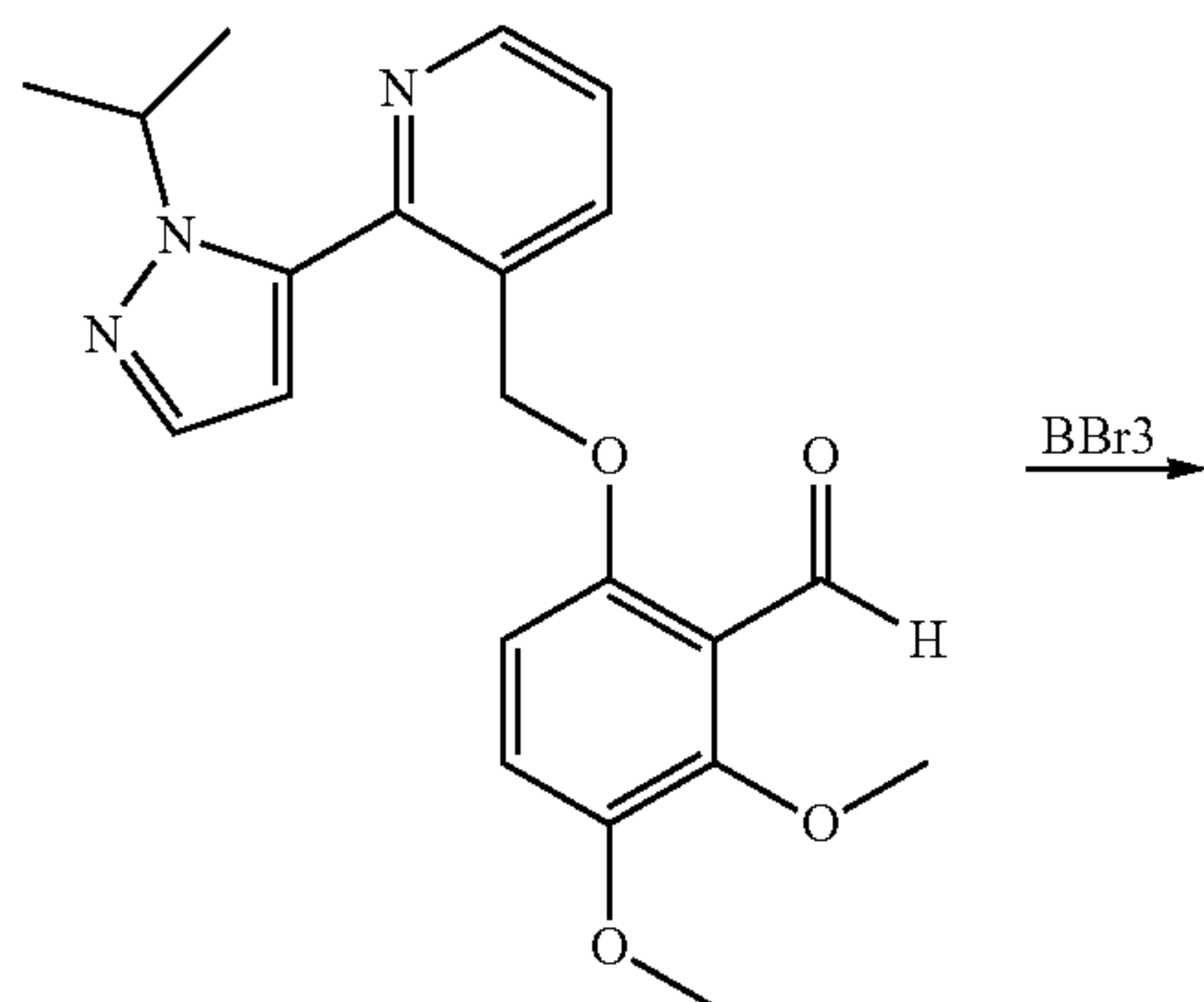
GBT1717
