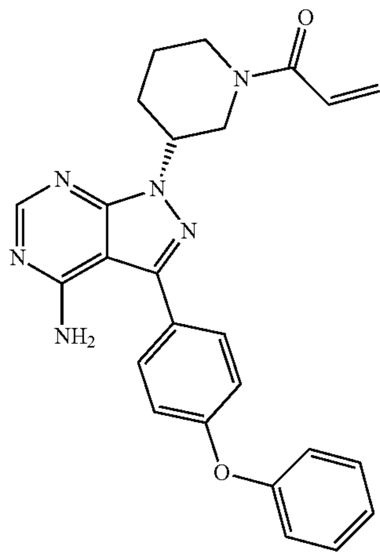
Ibrutinib
