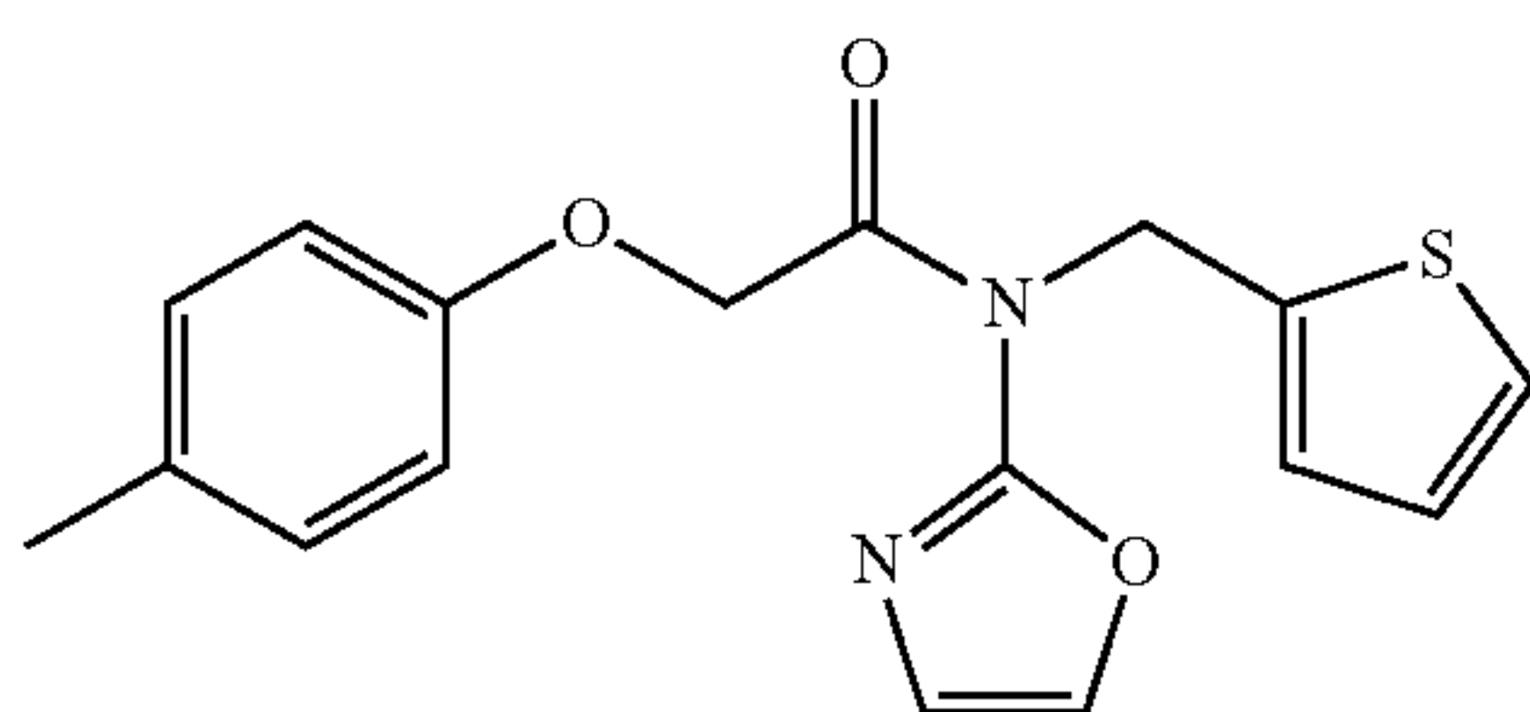
N-(oxazol-2-yl)-N-(thiophen-2-ylmethyl)-2-(p-tolyloxy)acetamide; Example 4
