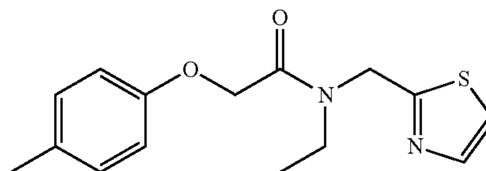
N-ethyl-N-(thiazol-2-ylmethyl)-2-(p-tolyl)oxyacetamide; Example 143
