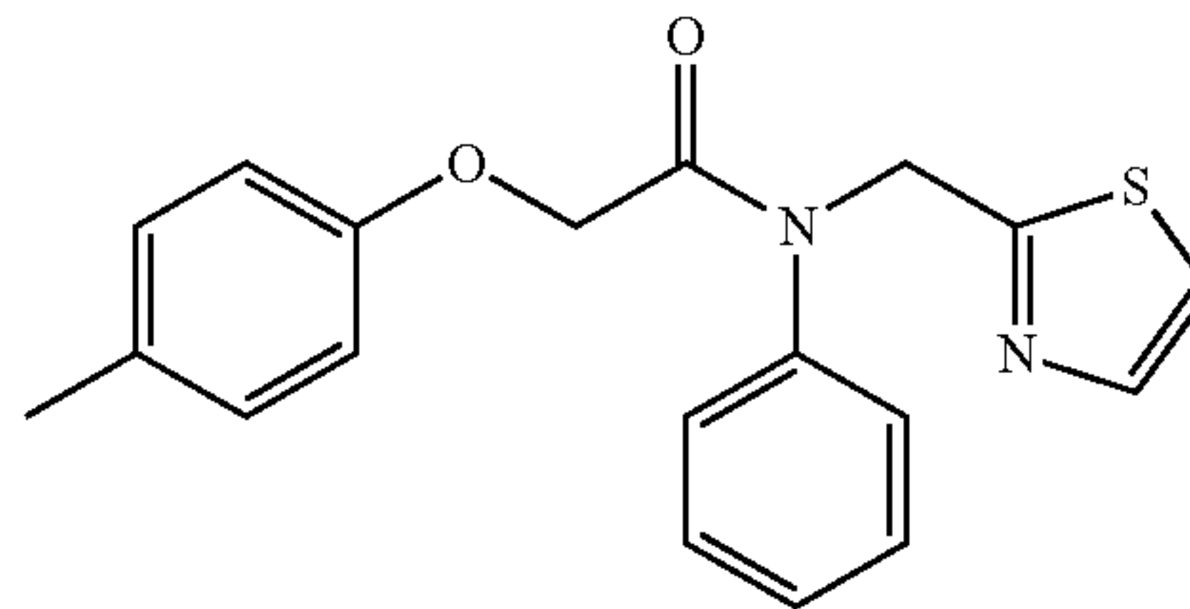
N-phenyl-N-(thiazol-2-ylmethyl)-2-(p-tolyloxy)acetamide; Example 82
