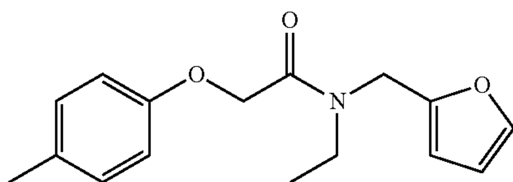
N-ethyl-N-(furan-2-ylmethyl)-2-(p-tolyloxy)acetamide; Example 74
