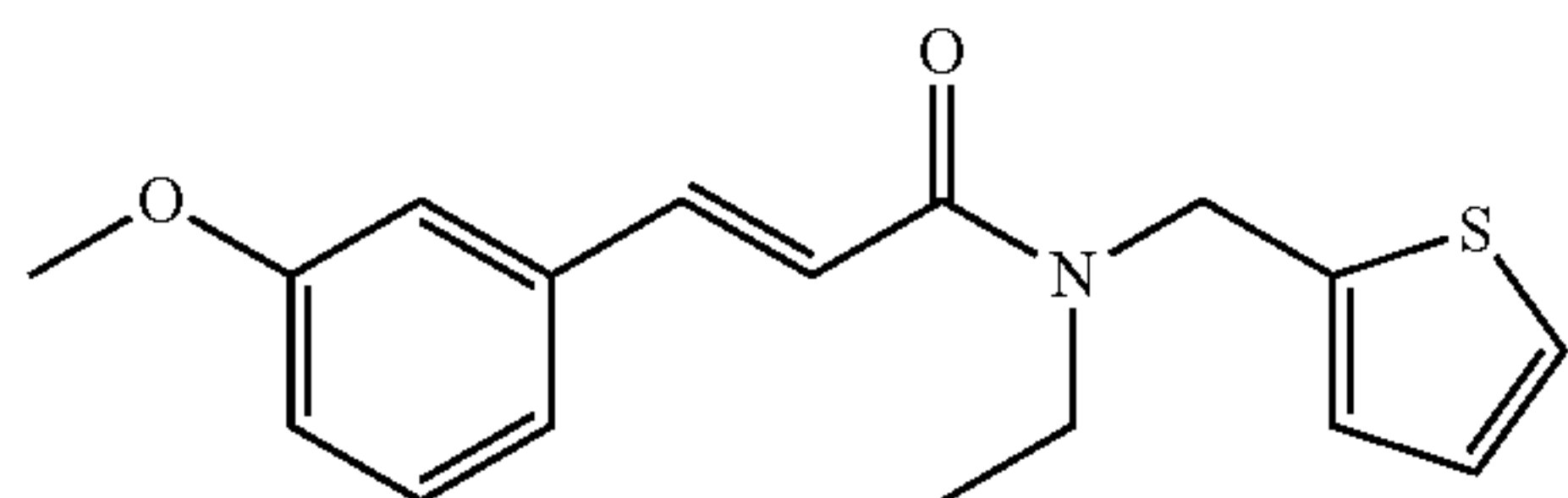
(E)-N-ethyl-3-(3-methoxyphenyl)-N-(thiophen-2-ylmethyl)acrylamide; Example 221
