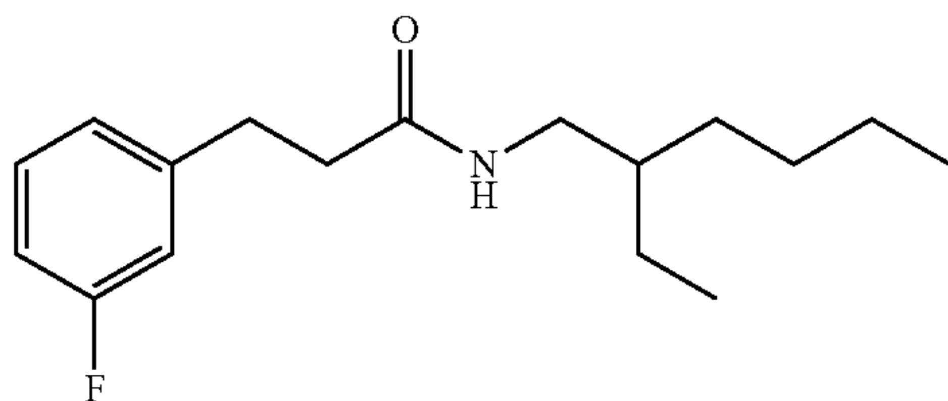
N-(2-ethylhexyl)-3-(3-fluorophenyl)propanamide; Example 140
