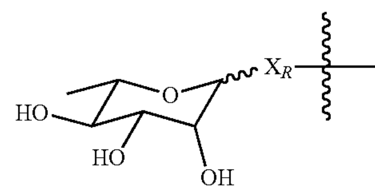
Rhamnose
