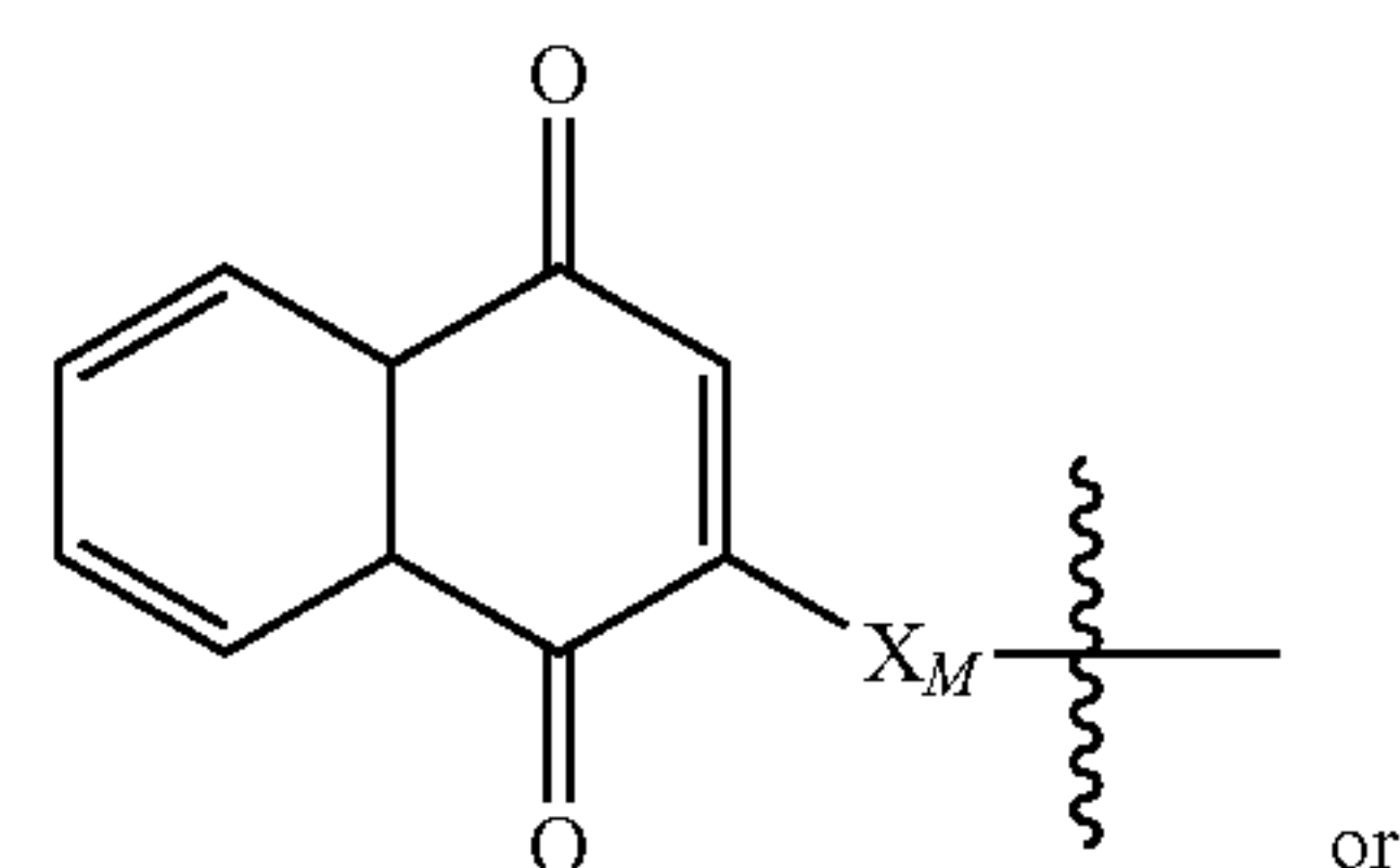
Menadione
