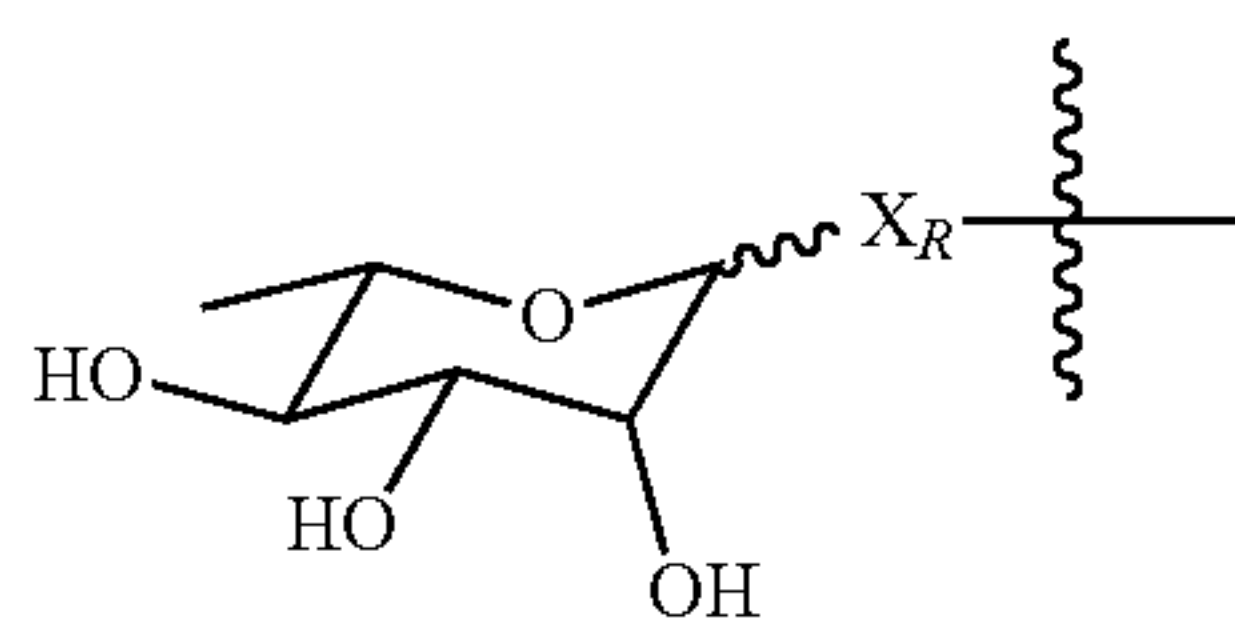
Rhamnose
