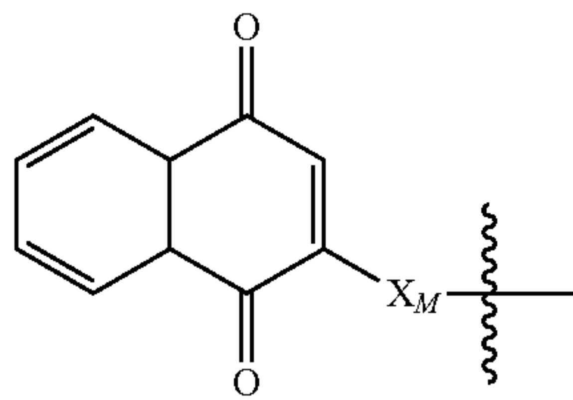
Menadione
