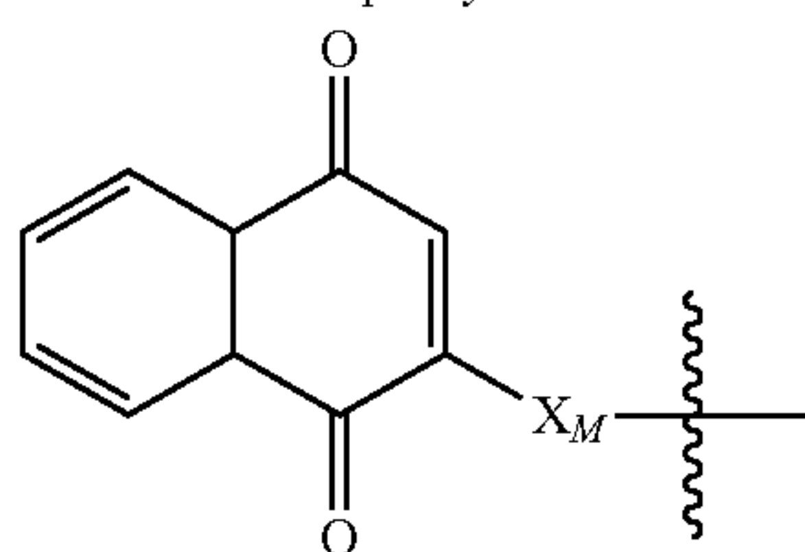
Menadione
