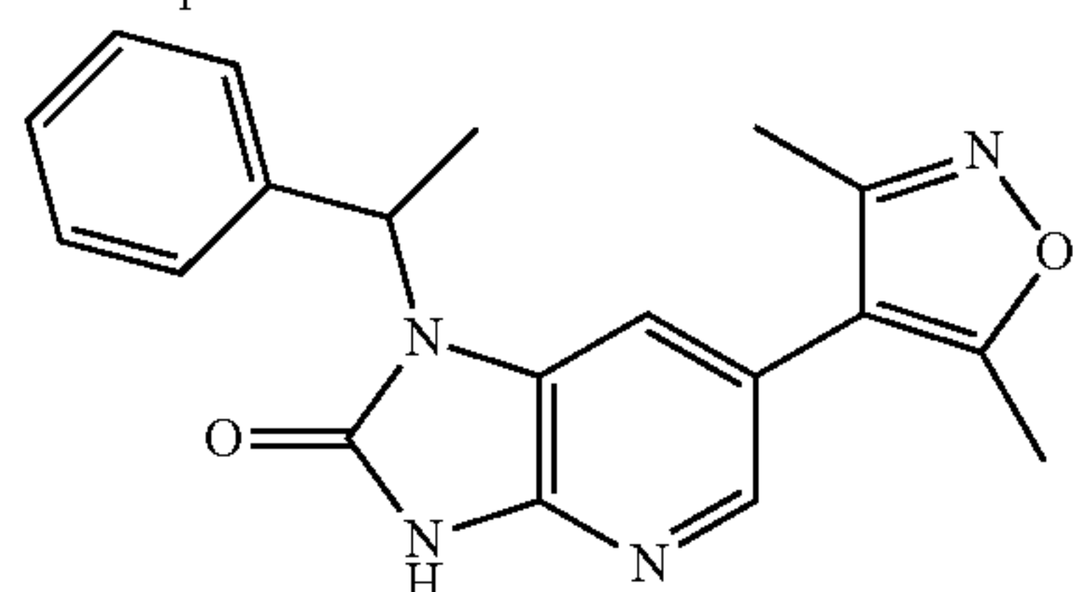
Enantiomer B
