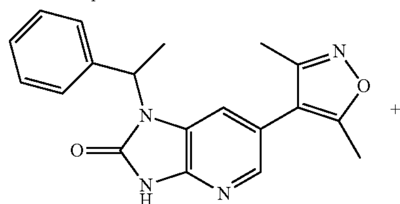
Enantiomer A
