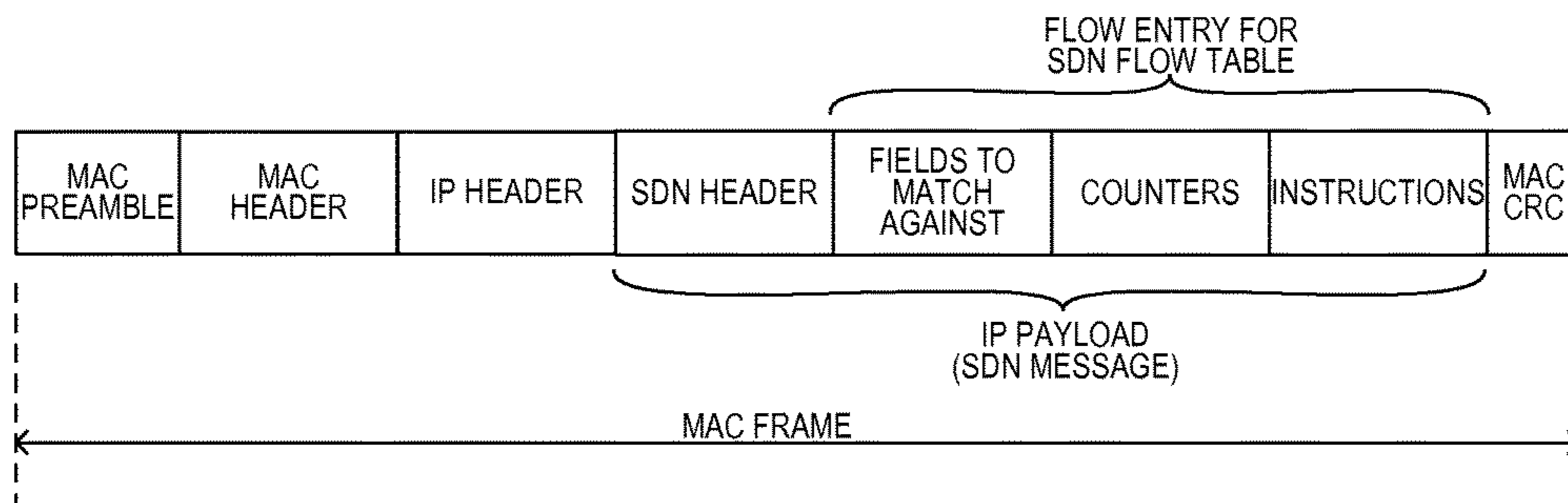
SDN MESSAGE FIG. 9
