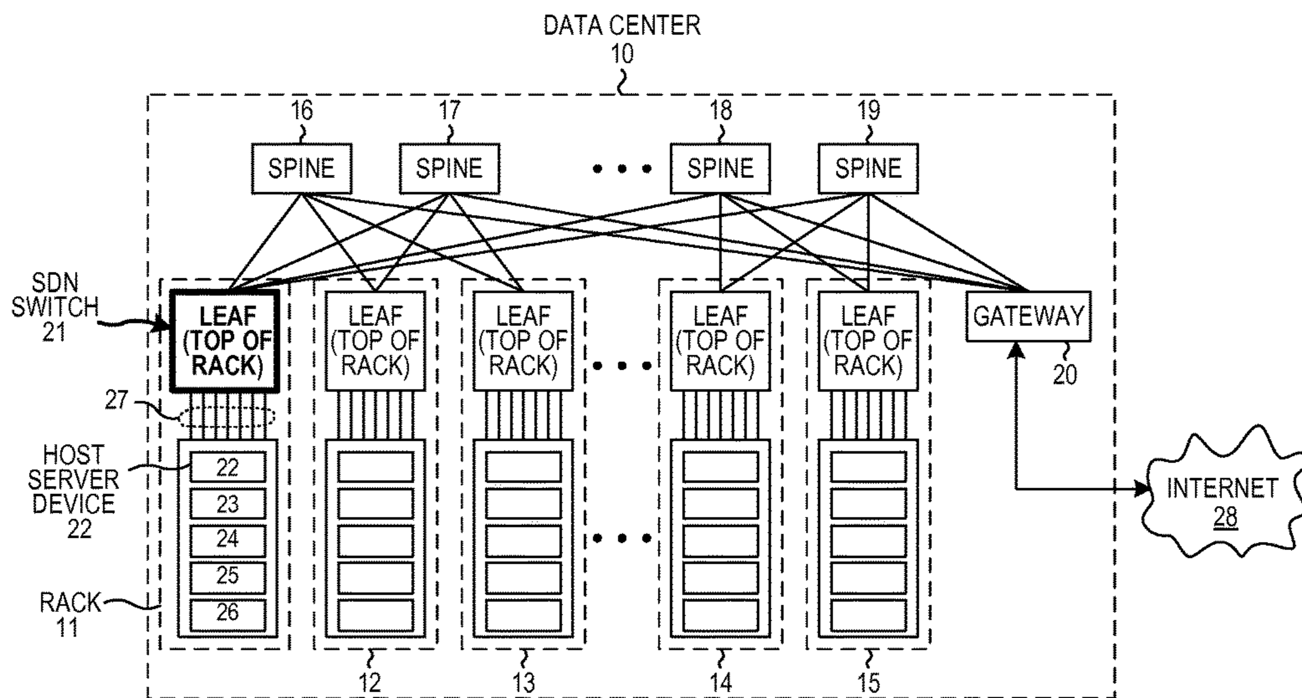
DATA CENTER FIG. 3
